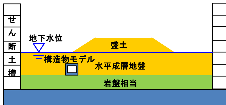
図-1 遠心模型実験の模型地盤及び構造物模型配置の基本イメージ (地下水位あり)
