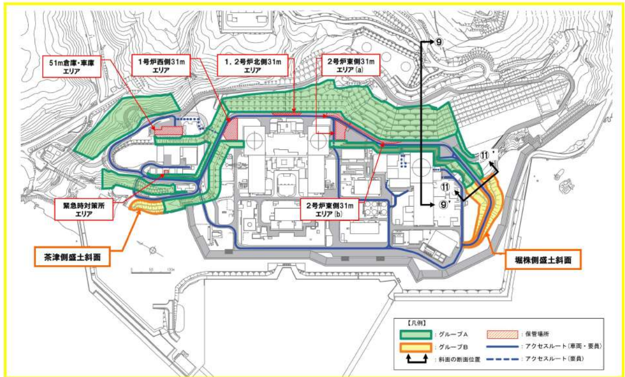
第 6-15 図 評価対象断面位置
