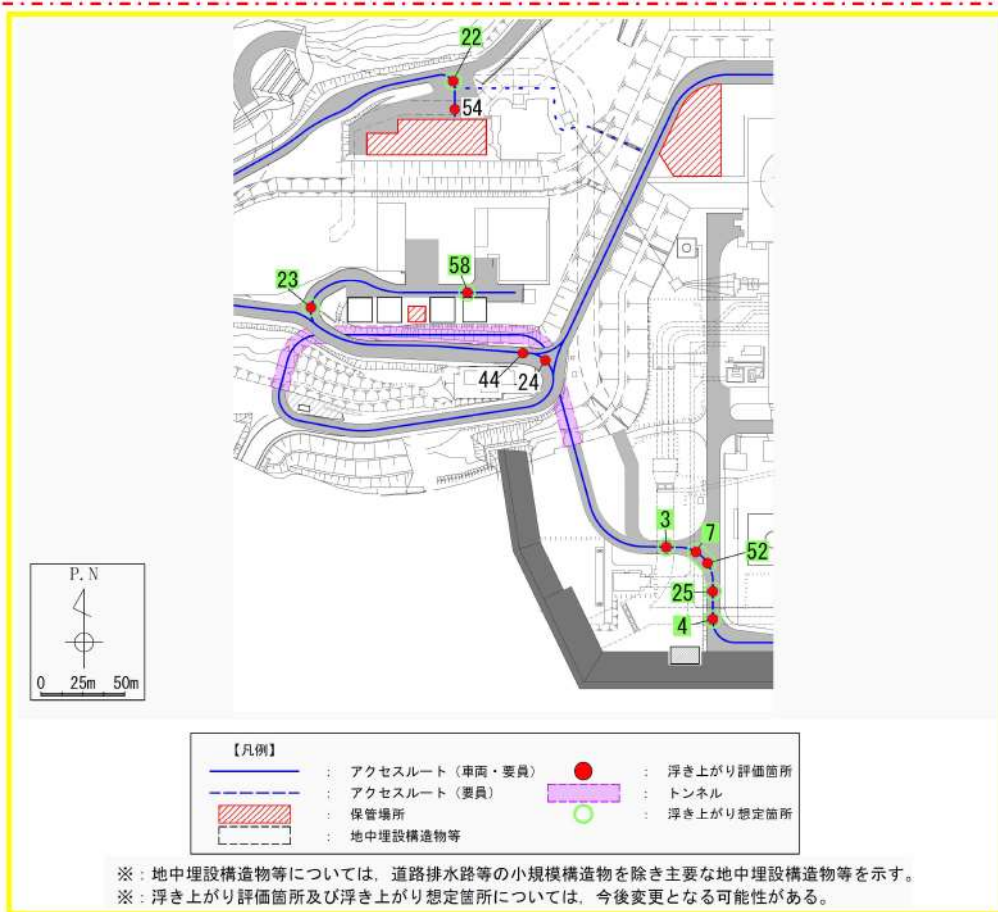
第6-42図 液状化による浮き上がりの評価結果 (2/5) (Aエリア)
