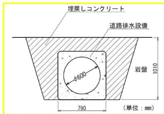
第 5-15 図 道路排水設備断面図
