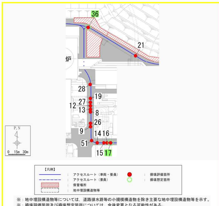
第 6-44 図 構造物損壊による段差発生想定箇所 (3/5) (B エリア)
