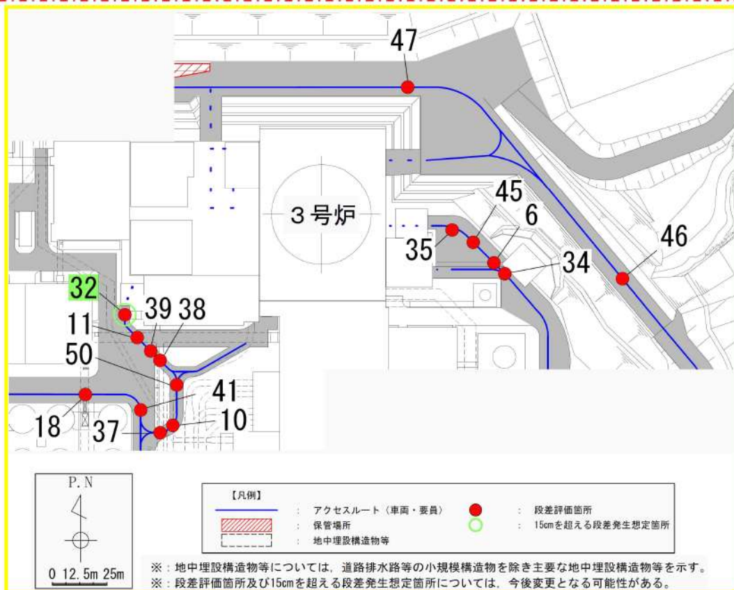
第 6-20 図 地中埋設構造物等と埋戻部との境界部における 段差評価結果（4/5）（C エリア）
