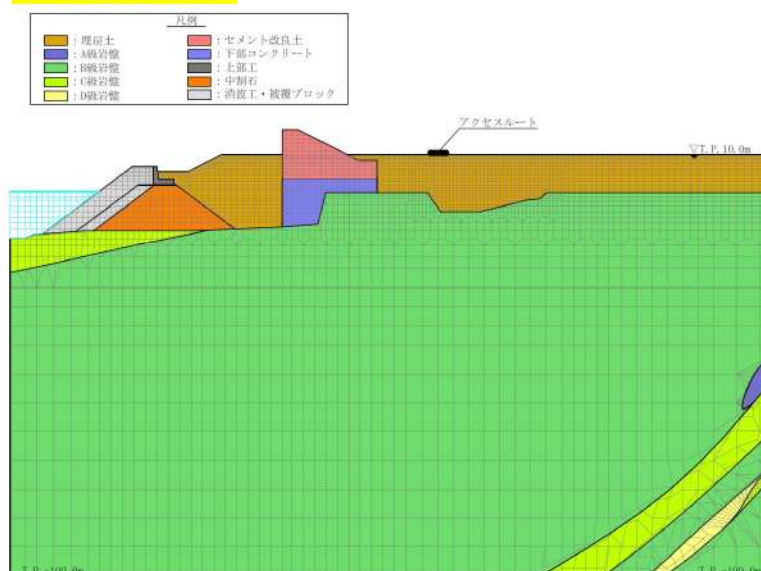
第 6-38 図 解析モデル図
