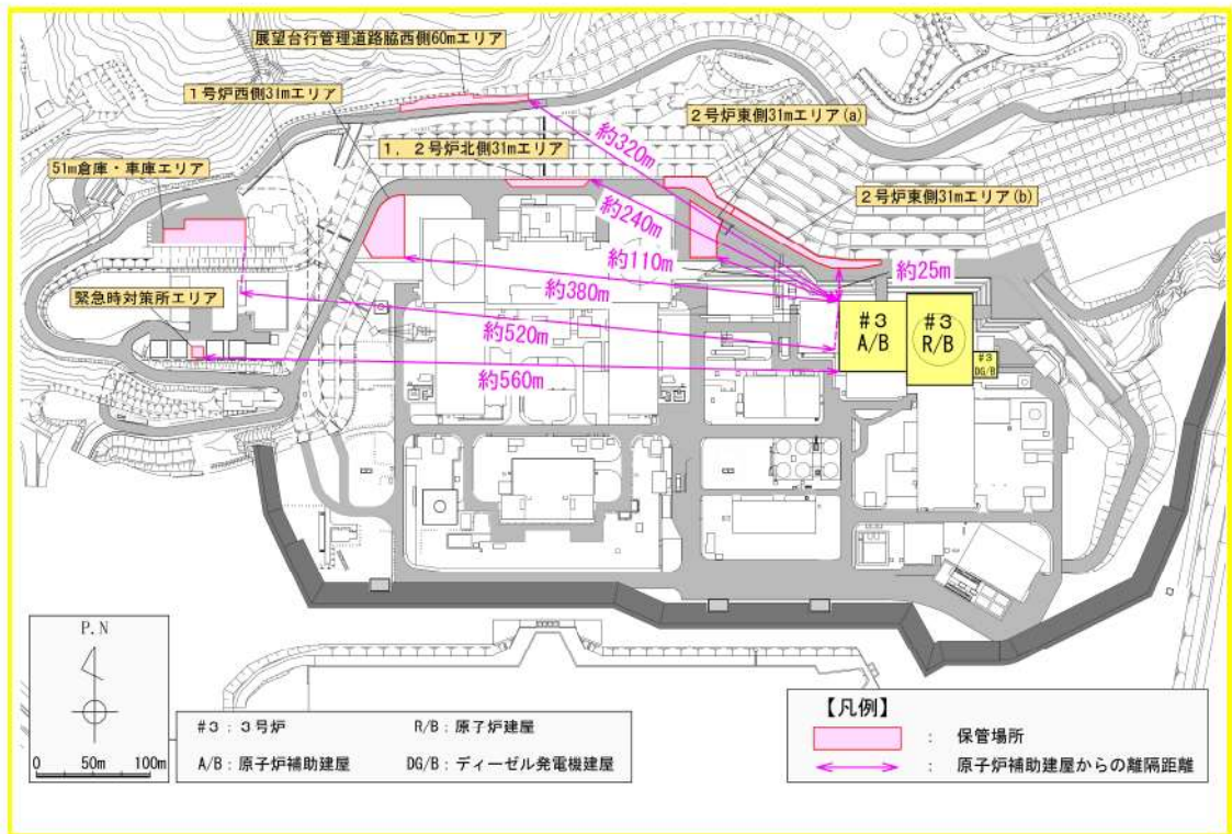
保管場所と原子炉補助建屋との離隔距離
