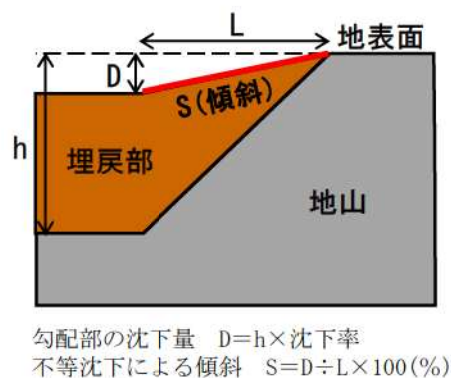
第 6-23 図 液状化及び揺すり込みによる沈下を考慮した傾斜の評価
