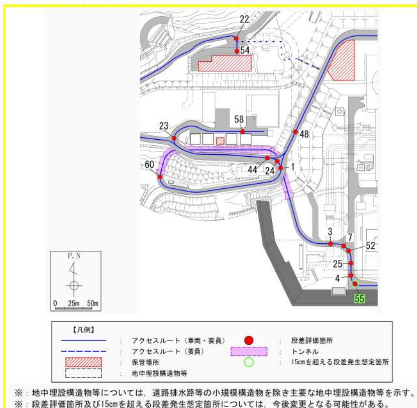
第 6-20 図 地中埋設構造物等と埋戻部との境界部における 段差評価結果 (2/5) (A エリア)
