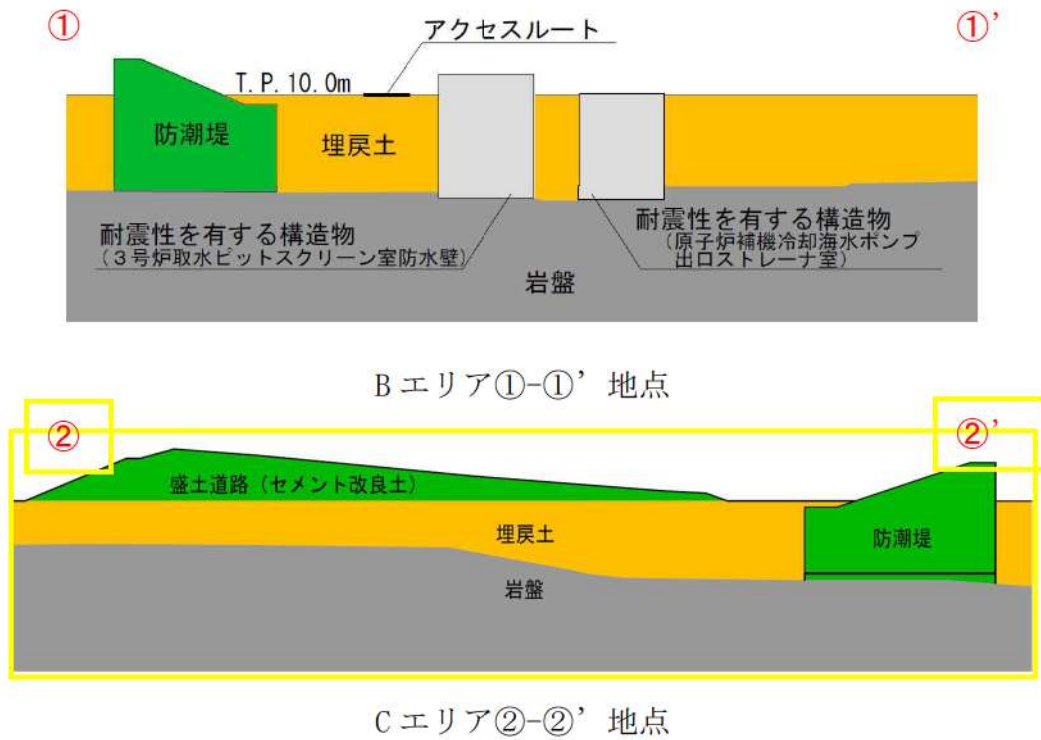
第 6-32 図 Bエリア①-①' 地点及びCエリア②-②' 地点断面図
