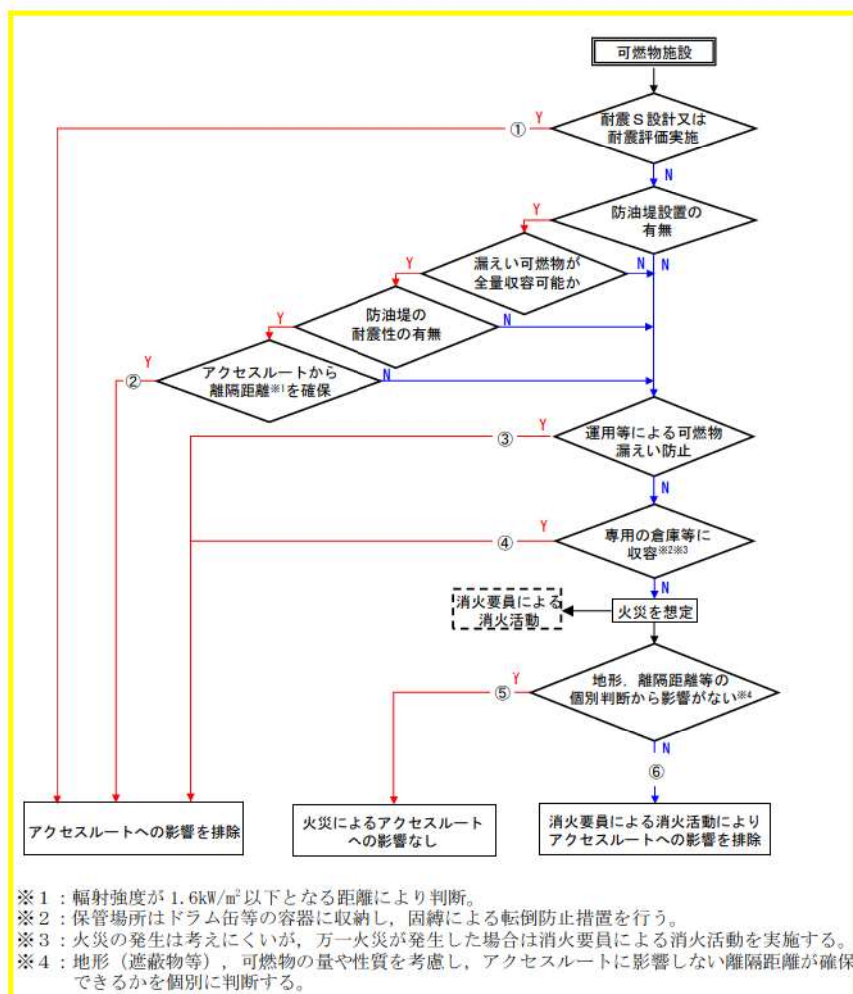
第 6-5 図 可燃物施設の損壊による影響評価フロー
