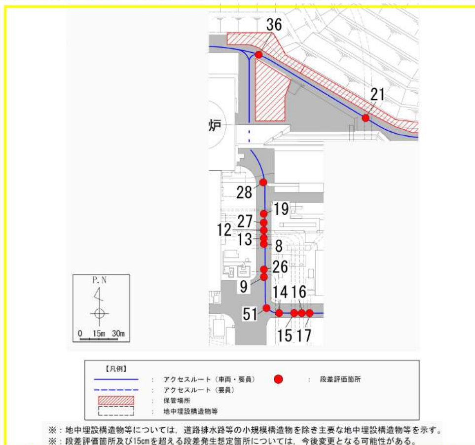
第 6-20 図 地中埋設構造物等と埋戻部との境界部における 段差評価結果 (3/5) (Bエリア)
