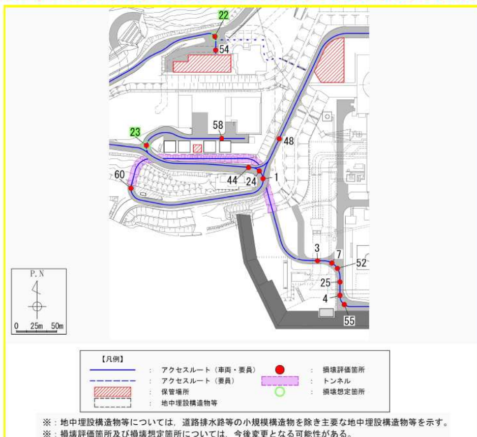
第 6-44 図 構造物損壊による段差発生想定箇所 (2/5) (A エリア)
