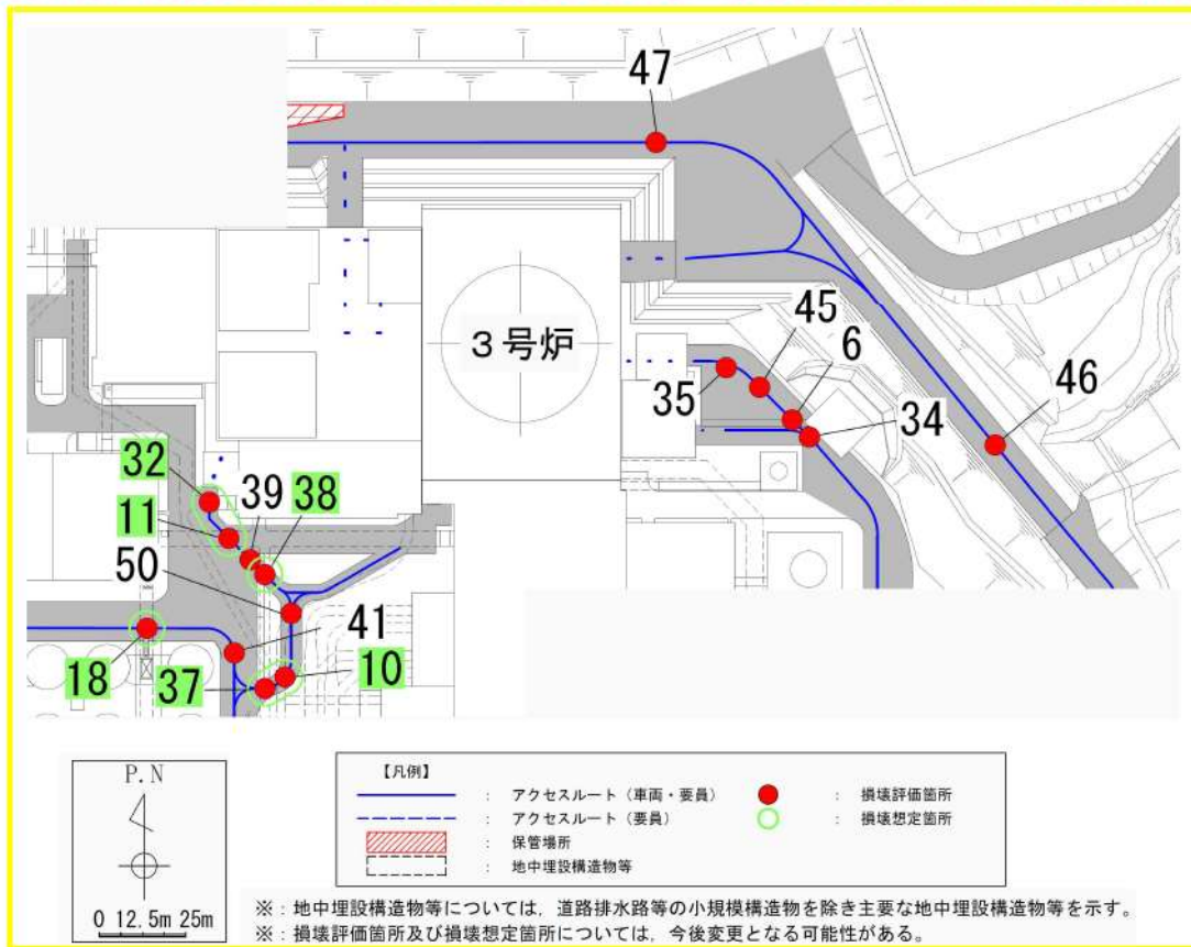
第 6-44 図 構造物損壊による段差発生想定箇所 (4/5) (C エリア)
