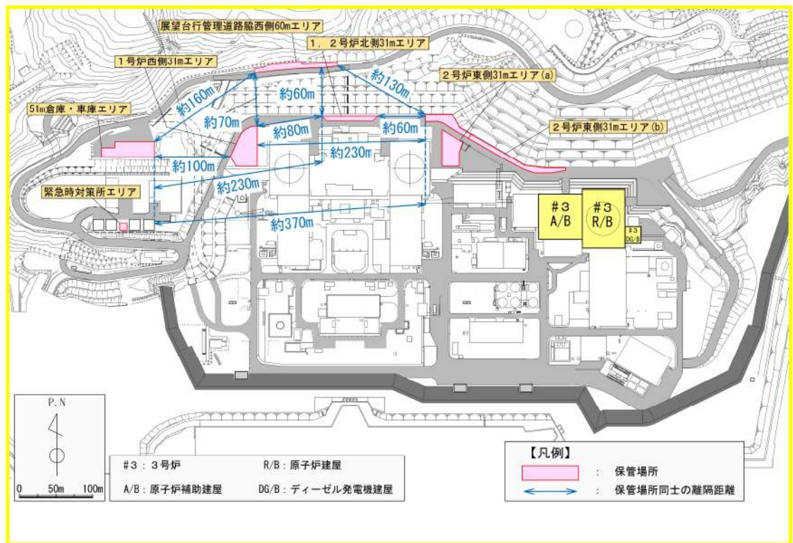
保管場所間の離隔距離
