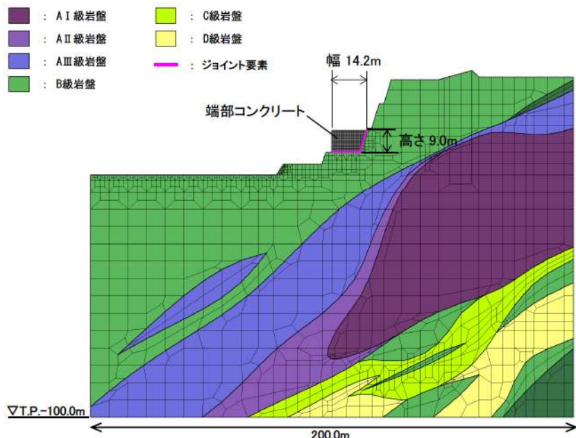
2次元動的FEM解析モデル(8-8'断面)
