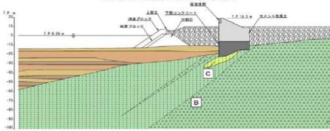
防潮堤（標準部）概要図
