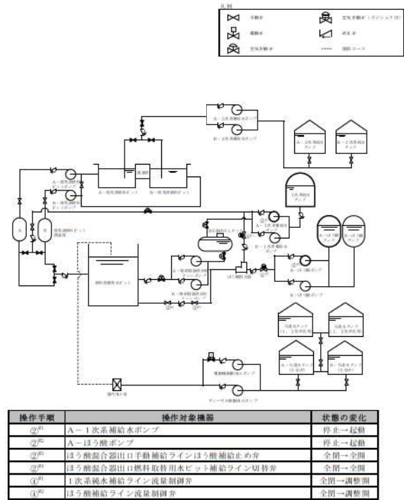
第1.13.16図 1次系純水タンク及びびほう酸タンクを水源とした1次系補給水ポンプ及びびほう酸ポンプによる燃料取替用水ピットへの補給 概要図
