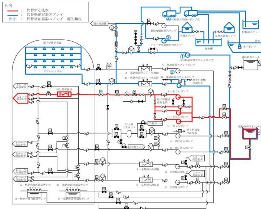
図1 概要図（代替格納容器スプレィと代替炉心注水を同時に行う場合）
