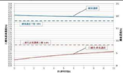
図61-6-1 緊急時対策所 プールム放出期間中の酸素濃度及び二酸化炭素濃度変化
