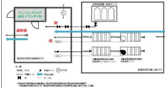
換気空調設備の系統に関する点検（検査性）概要図（ブルーム通過前後）
