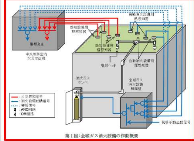
第1図：全城ガス消火設備の作動概要
