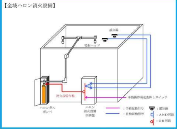
図1 ハロン消火設備概要図
