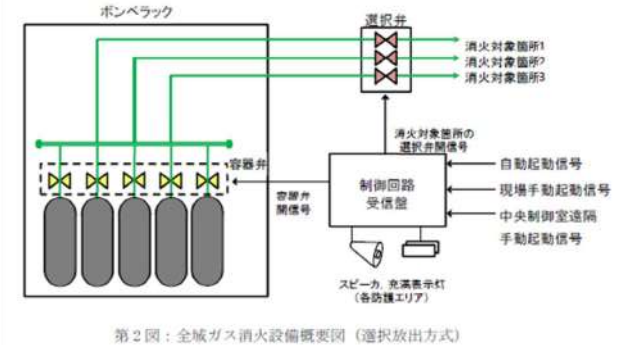
第2図：全城ガス消火設備概要図 (選択放出方式)
