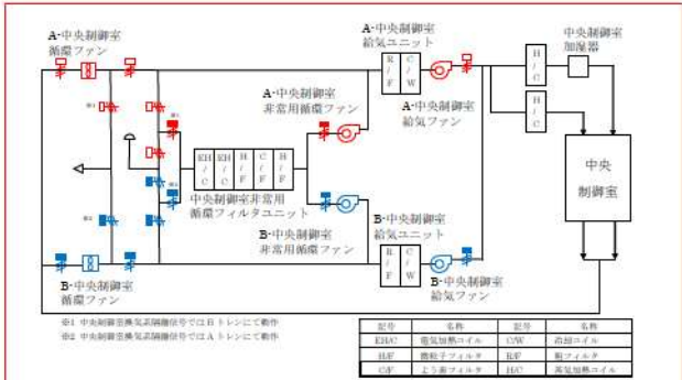
第9図 中央制御室換気空調設備の概要
