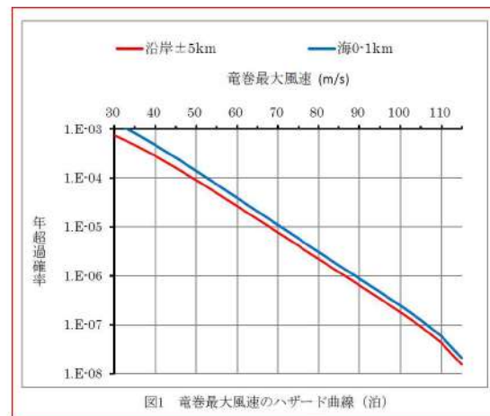
図1 竜巻最大風速のハザード曲線（泊）
