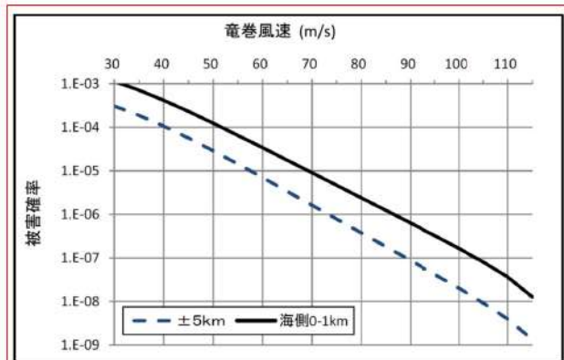
図1 竜巻最大風速のハザード曲線（大飯）
