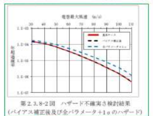
第 2.3.8-2 図 ハザード不確かさ検討結果 (バイアス補正後及び全パラメータ+1σのハザード)
