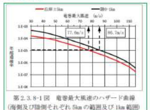
第 2.3.8-1 図 竜巻最大風速のハザード曲線 (海側及び陸側それぞれ 5km の範囲及び 1km 範囲)
