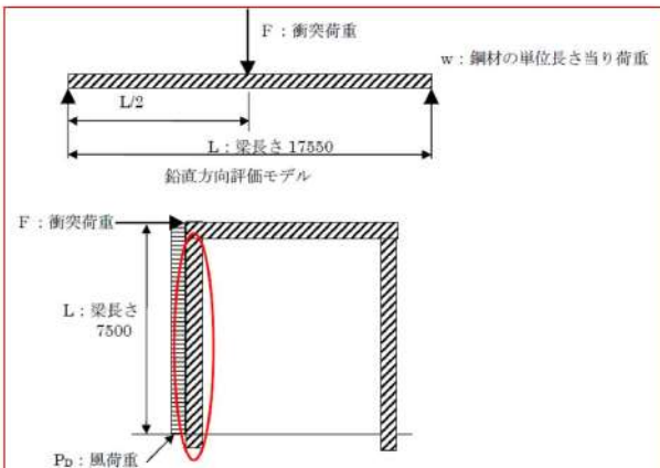
図3 評価モデル（海水ポンプ竜巻防護施設）
