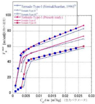
図4 Simiu & Scanlan 及び江口ほか（電中研）による解析結果との比較【飛来物の速度】 ※Type-I、II、IIIのうち、最大風速が最も大きいType-Iと最大風速が最も小さいType-IIについて比較を行った。
