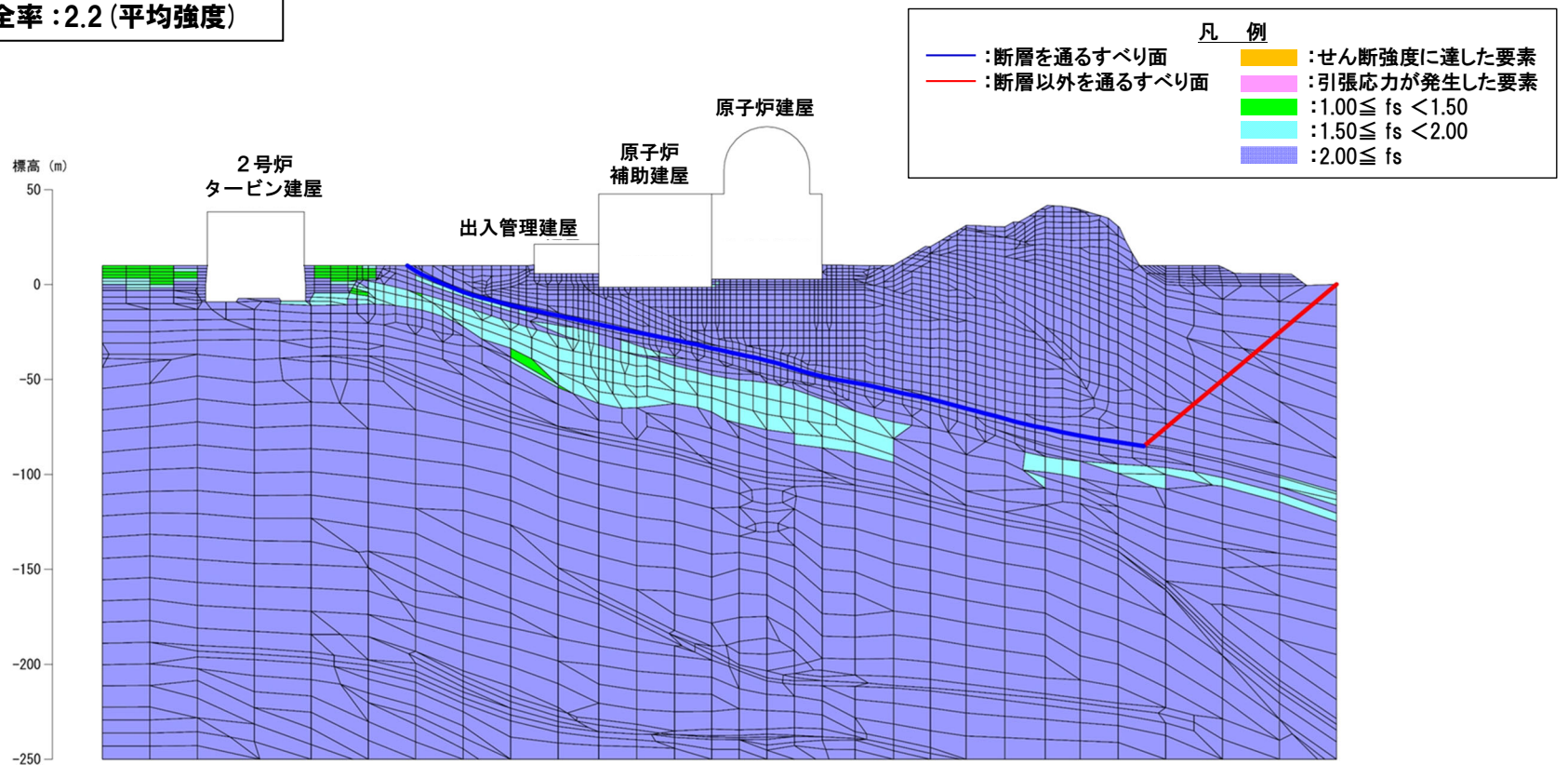
要素ごとの安全係数図（静的非線形解析）：X-X'断面（原子炉建屋基礎地盤）
