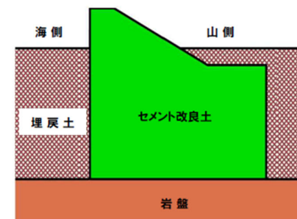
1-2図 防潮堤概要図
