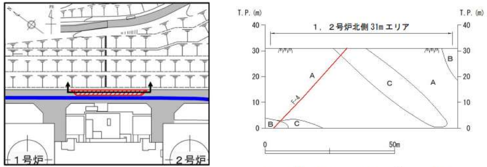
第5-11図 1, 2号炉北側31mエリア平面図及び地質断面図
