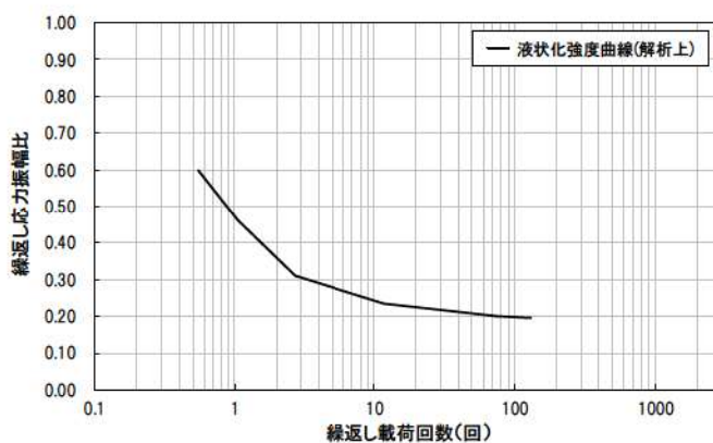
第 6-39 図 液状化パラメータ
