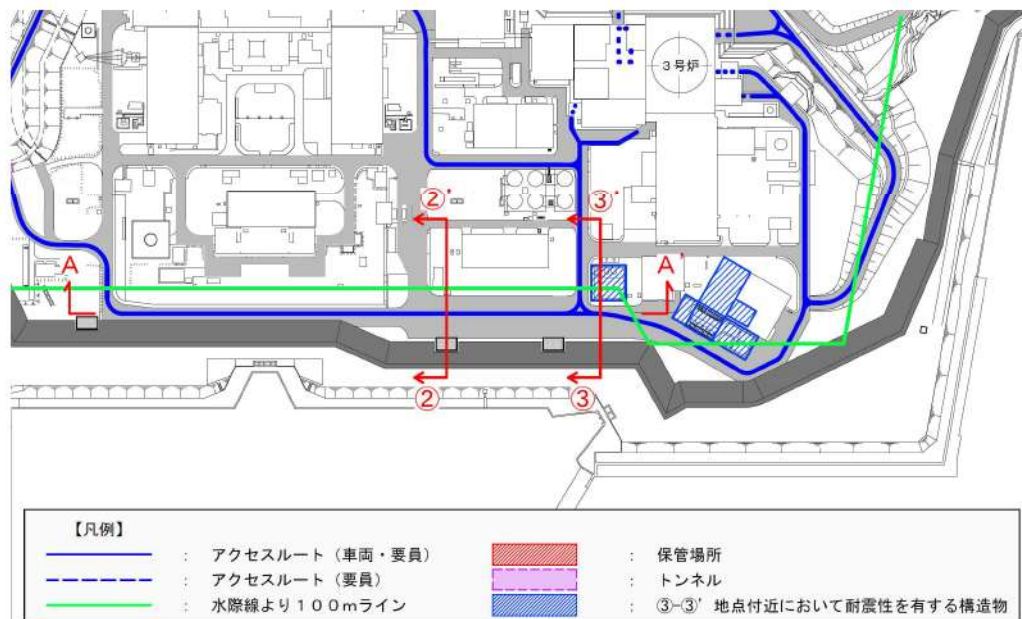
第 6-35 図 検討断面位置図
