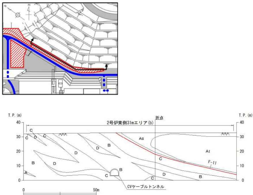
第5-13図 2号炉東側31mエリア(b)平面図及び地質断面図
