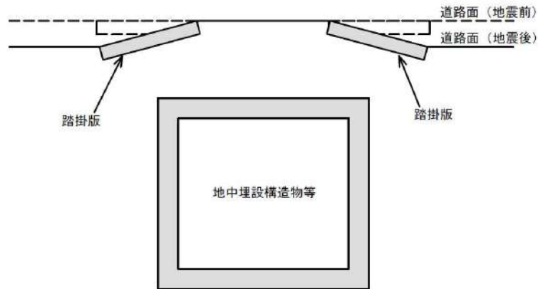
第6-21図 段差緩和対策概念図
