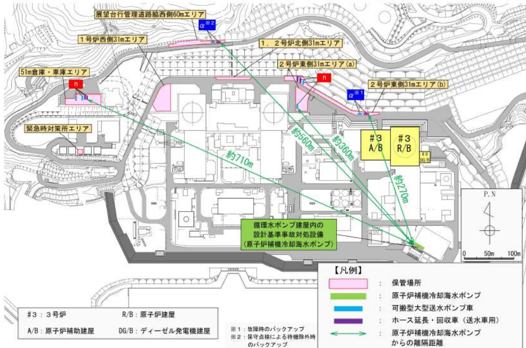
可搬型大型送水ポンプ車及びホース延長・回収車（送水専用）と原子炉補機冷却海水ポンプとの離隔距離
