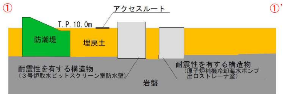
第 6-32 図 B エリア①-①' 地点断面図
