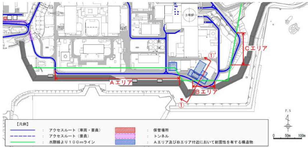
第 6-31 図 検討対象範囲の位置図
