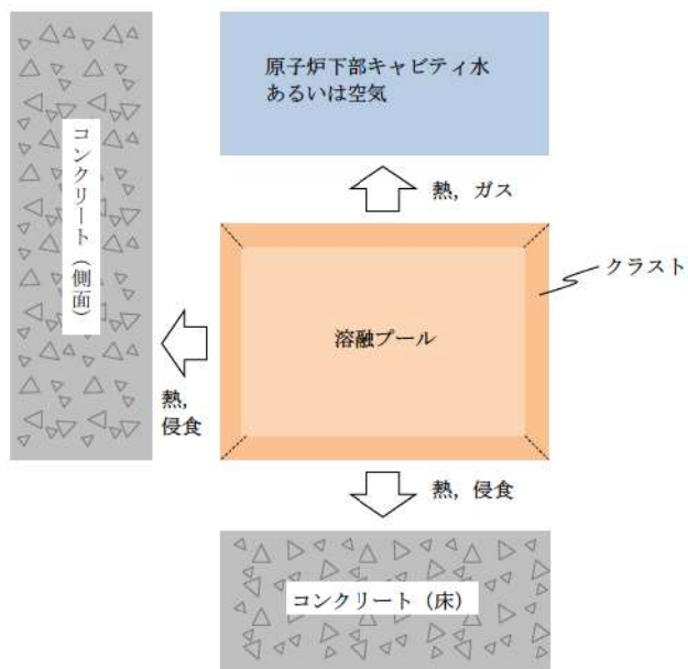
図 3.3-16 溶融炉心の伝熱の概念
