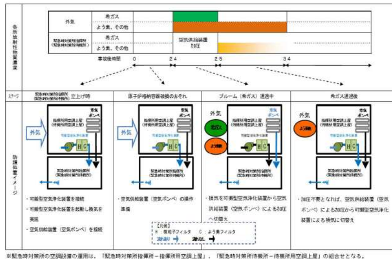
図添10-1 緊急時対策所換気空調設備等のイメージ図 (「61-8 適合状況説明資料(補足説明資料)」から抜粋)
