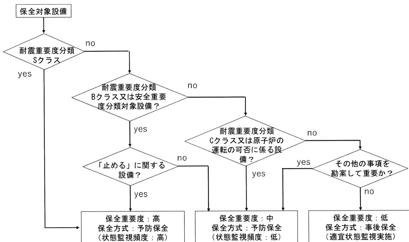
図1 保全重要度分類の選定フロー
