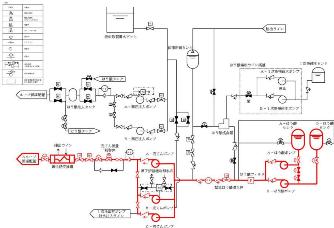
第 10-1 図 ほう酸水注入 (ほう酸タンク→充てんライン) システム概要図
