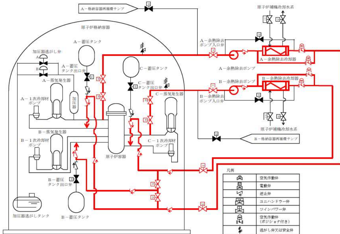
1次冷却系のフィードアンドブリード（余熱除去設備による冷却）
