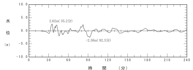
津波地震
