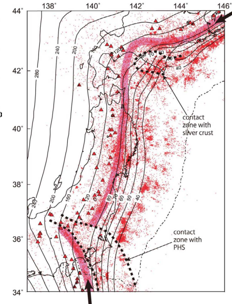
太平洋スラブ地殻内の地震の分布 (長谷川ほか(2012)) 赤点:プレート境界から下方に0~10kmの範囲の地震 ピンク色の網目:上面地震帯 黒線:太平洋スラブ上部境界面の形状 黒点線:太平洋スラブが直上のフィリピン海スラブ及び前弧スリバー地殻と接触している領域
