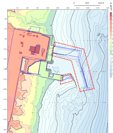
防波堤無し
