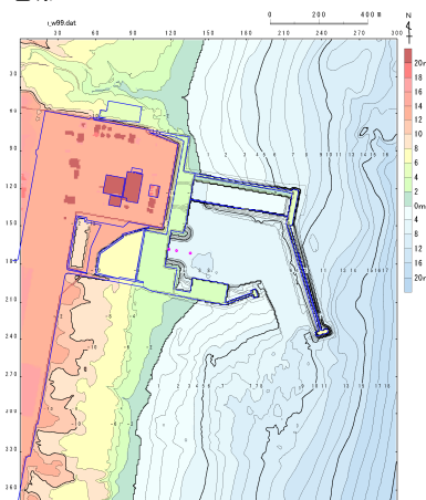
防波堤有り
