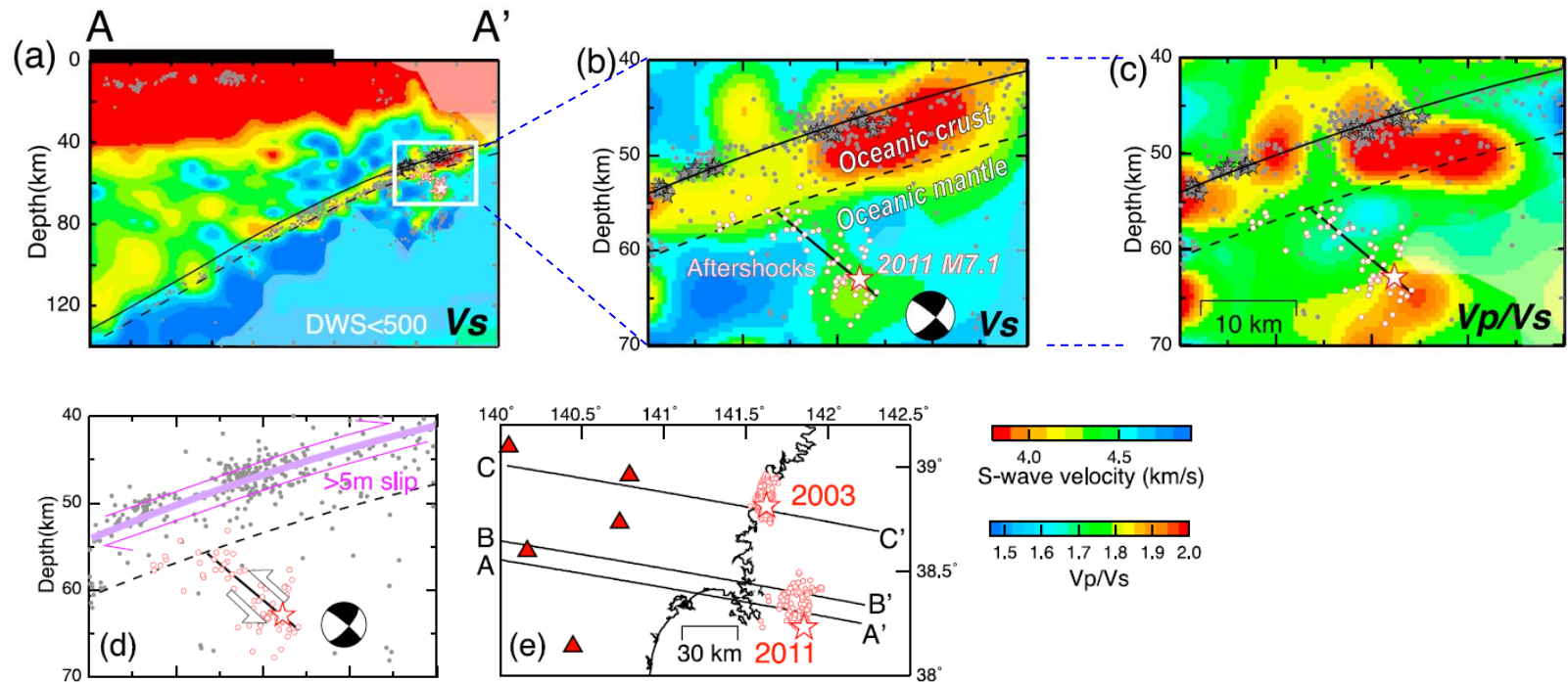
4.7地震の震源域周辺のS波速度構造等の鉛直分布図[Nakajima et al.(2011)に一部加筆] 白丸は再決定した余震。黒の太線はメカニズム解から推定した断層面。黒実線はプレート境界。破線は海洋プレートモホ面。
