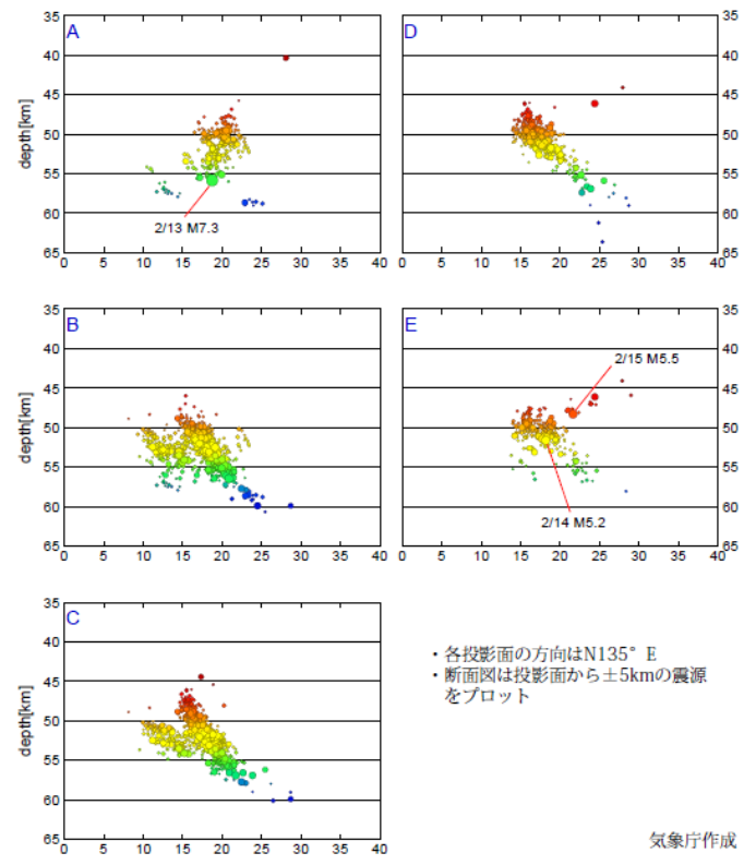
DD法による再計算震源分布
