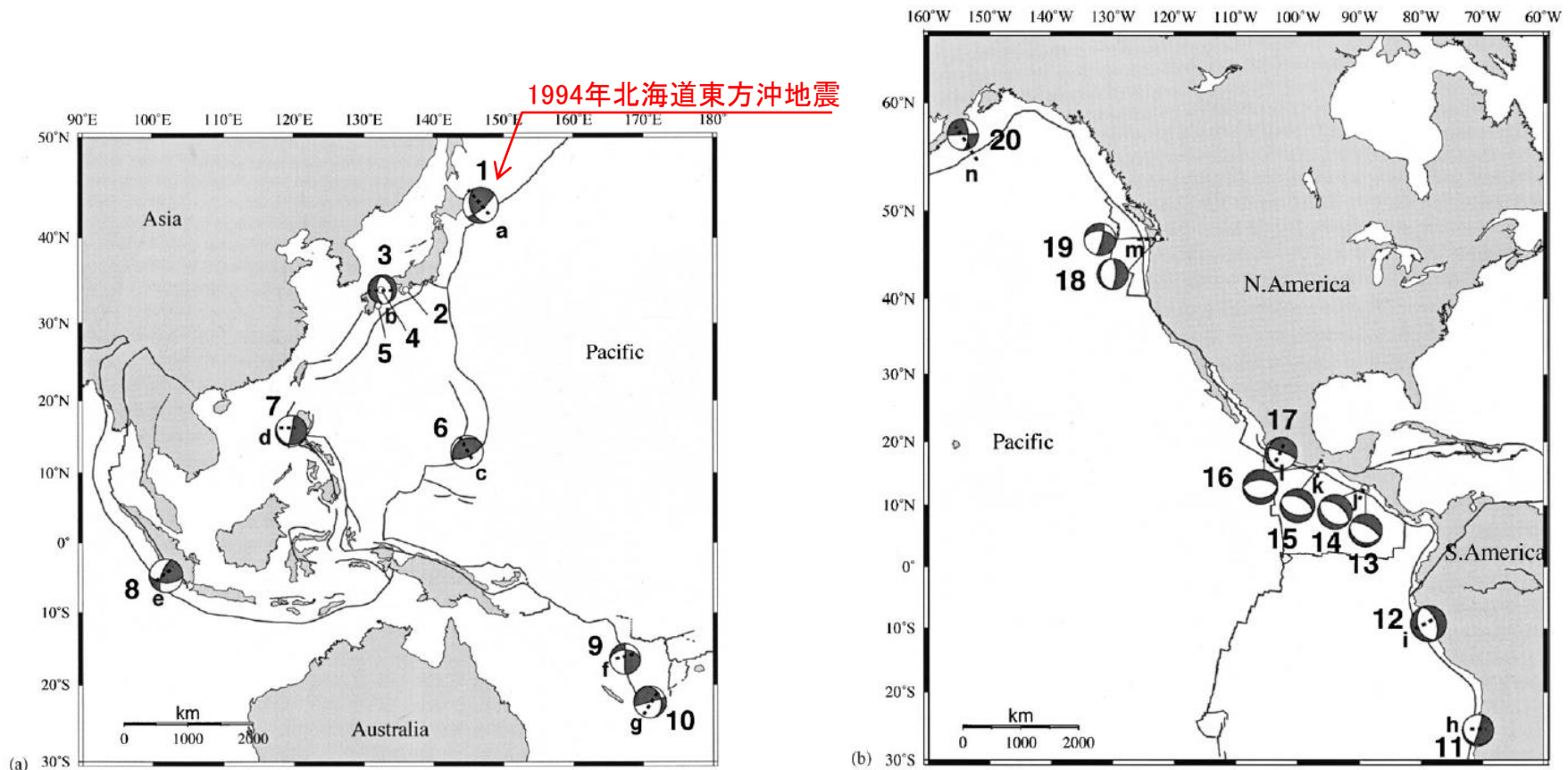
規模の大きな浅い海洋プレート内地震の震源メカニズム [Seno and Yoshida(2004)に一部加筆]
