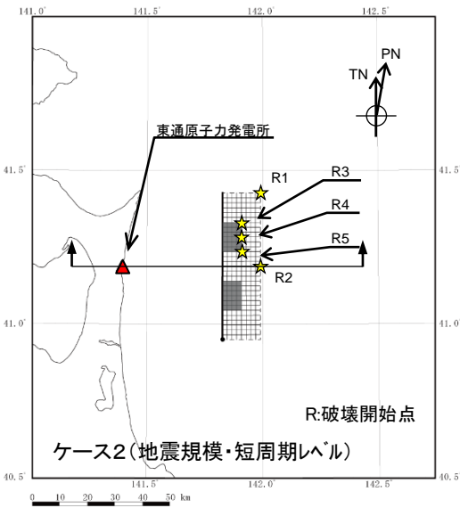
断層配置図
