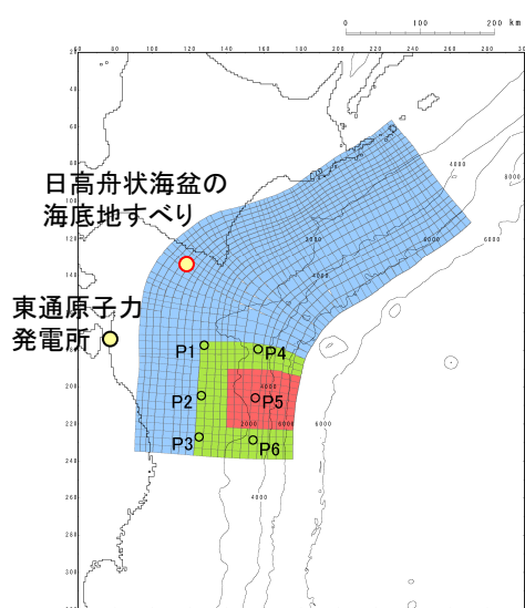
十勝沖・根室沖から岩手県沖北部の連動型地震(基準断層モデル①(内閣府(2012)考慮))
