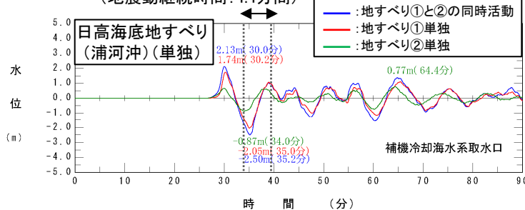
発電所地点(補機冷却海水系取水口前面位置)における水位時刻歴波形
