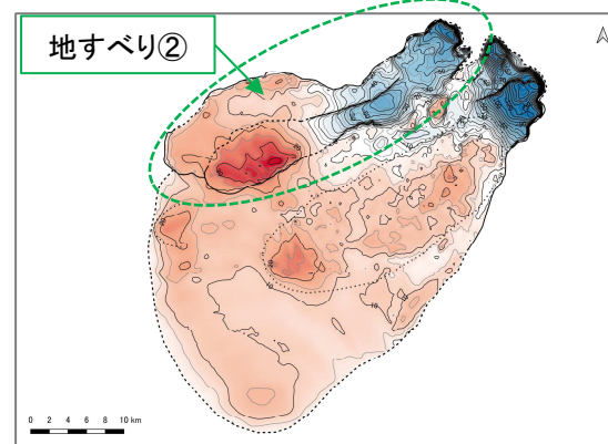
日高舟状海盆の海底地すべり (地すべり②単独) (比高変化分布)
