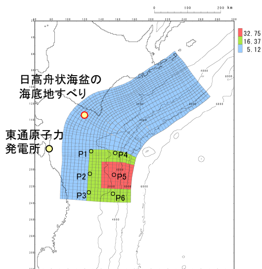
十勝沖・根室沖から岩手県沖北部 の連動型地震 (基準断層モデル①(内閣府(2012)考慮))
