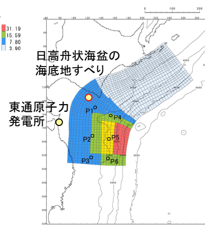
基準断層モデル③(海溝側強調) 破壊開始点:P1
