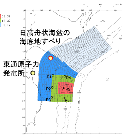
基準断層モデル②(すべり量割増) 破壊開始点:P4
