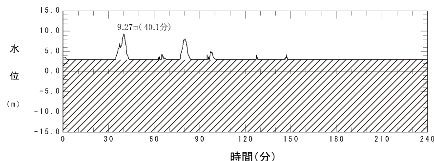
十勝沖・根室沖から岩手県沖北部の連動型地震に伴う津波 (基準断層モデル①(内閣府(2012)考慮))※
