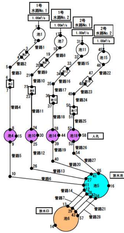
【1号及び2号炉放水施設の管路解析モデル図】
