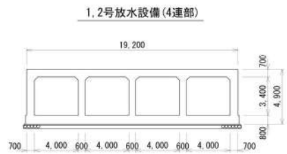
1,2号放水設備 (4連部)
