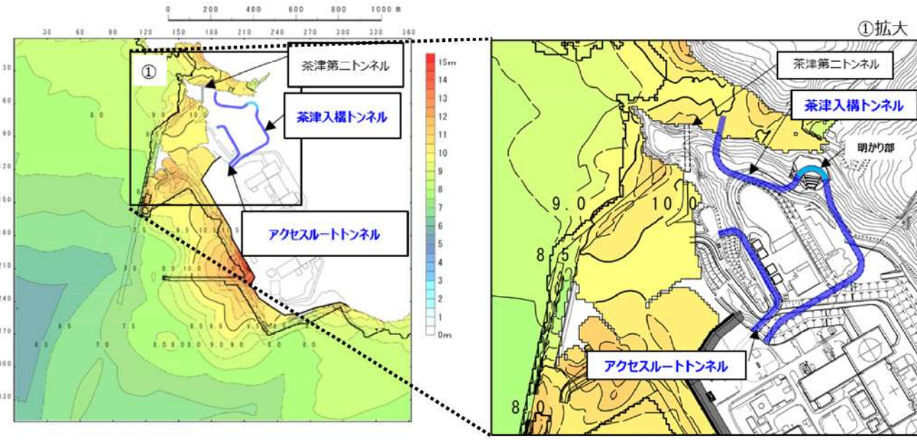
最大水位上昇量分布図※2
