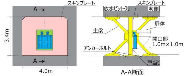
【1号及び2号炉放水路逆流防止設備概念図】
