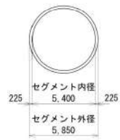
1,2号放水設備 (4連部)
