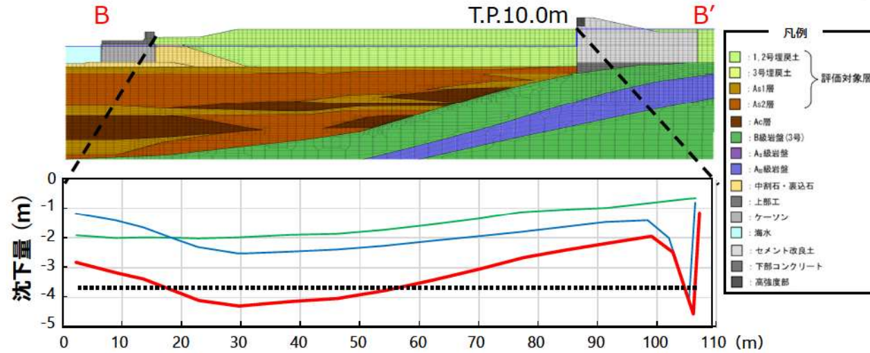
— : 揺すり込み及び過剰間隙水圧消散に伴う沈下量【①】 — : 基準地震動による液状化に伴う側方流動による沈下量【②】 — : 津波評価における沈下量【①+②】 (..... : 平均沈下量 = 3.32m)
