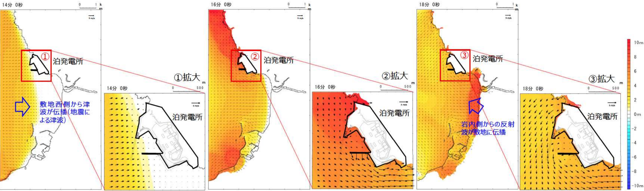
水位変動量・流速分布の経時変化(スナップショット)(1/2)※ ※現時点の評価における防潮堤前面が最大水位となるケース(波源F・北防波堤損傷)を例示する。
