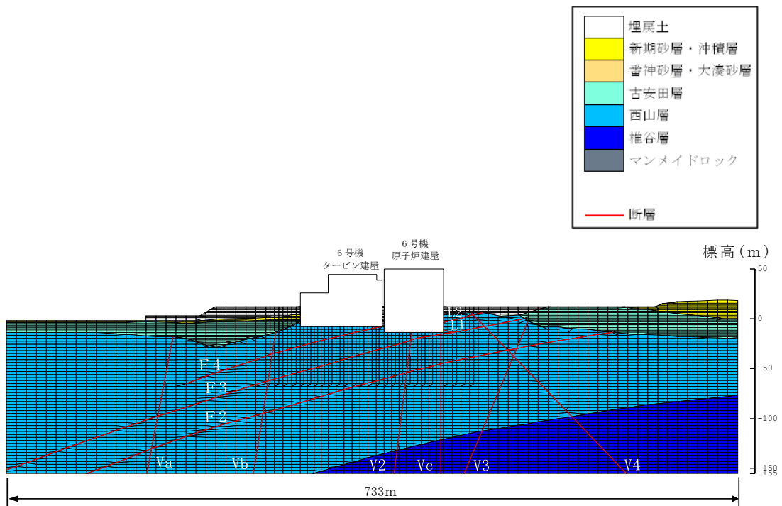
図-3 解析用要素分割図 (6号機原子炉建屋汀線直交断面)
