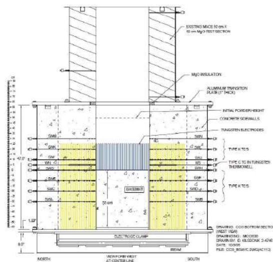
図 3. 1-35 CCI 実験装置
