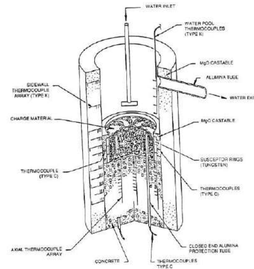
図 3.1-9 WETCOR 実験装置
