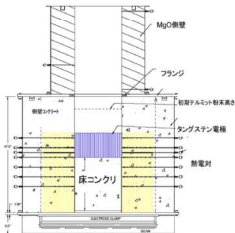
付図 2-13 C C I 実験のテスト部 [12]
