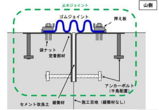
施工目地における止水ジョイント構造 (A-A' 断面)
