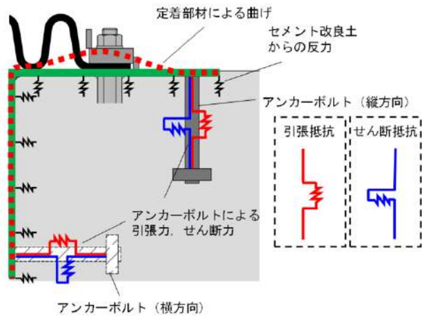
解析②のモデルとセメント改良土に固定するために生じる力のイメージ図
