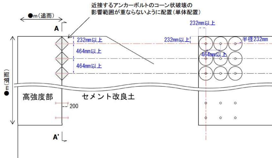
断面図
