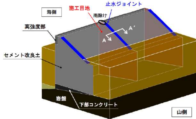
施工目地及び止水ジョイントの設置位置
