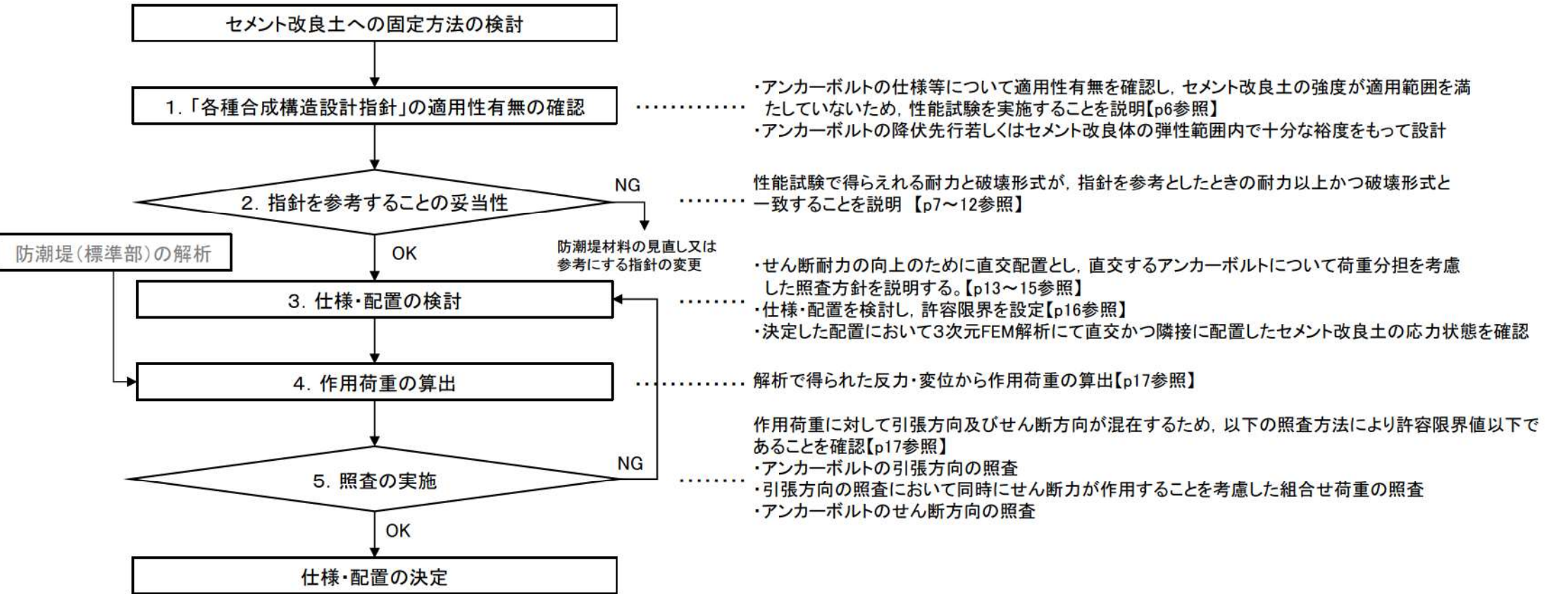
アンカーボルトの設計フロー
