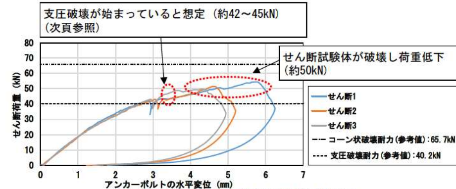
アンカーボルトの水平変位とせん断荷重の関係
