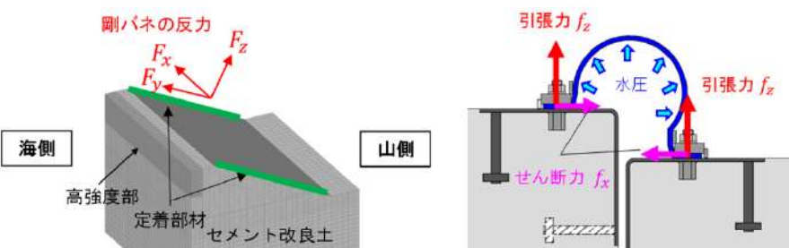
アンカーボルトの作用荷重
