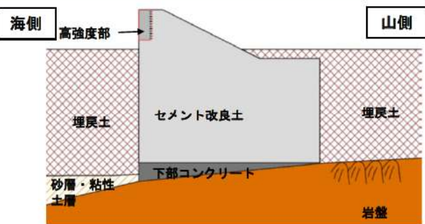
セメント改良土 (高強度含む) 概略図
