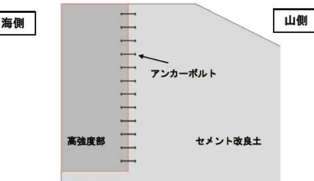
高強度部拡大図 (イメージ図)
