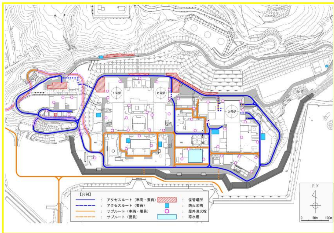
第2図 屋外消火栓及び防火水槽の配置図
