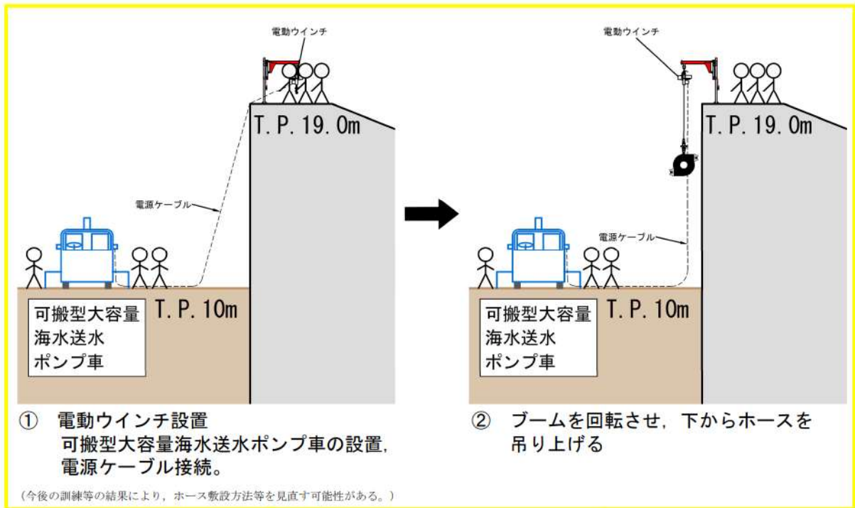
第 12 図 電動ウインチ使用手順
