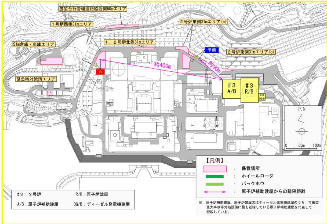
ホールローダ及びバックホウと原子炉補助建屋との離隔距離
