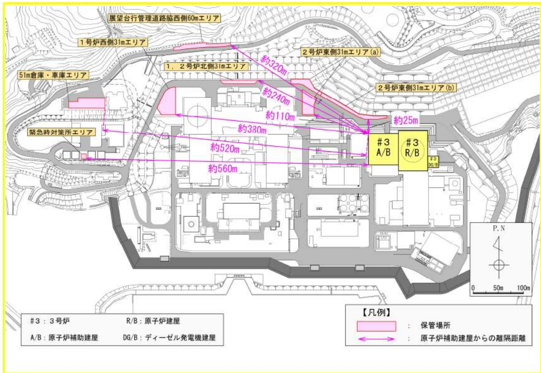
保管場所と原子炉補助建屋との離隔距離
