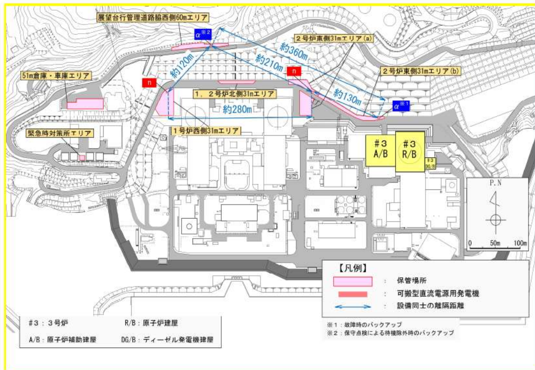
可搬型直流電源用発電機の相互の離隔距離
