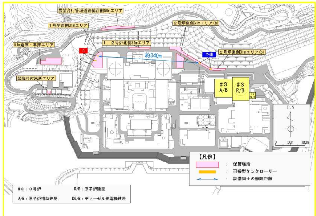
可搬型タンクローリーの相互の離隔距離
