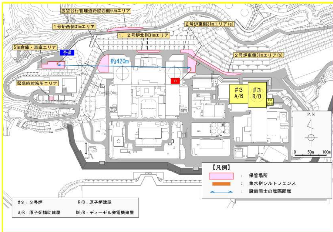
集水枥シルトフェンスの相互の離隔距離
