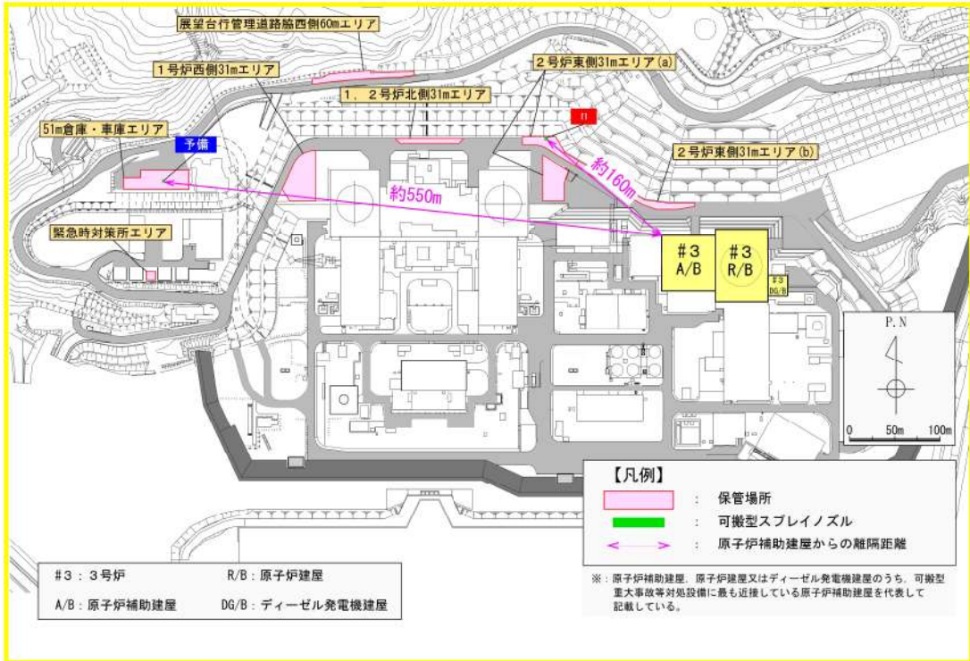
可搬型スプレインゾルと原子炉補助建屋との離隔距離
