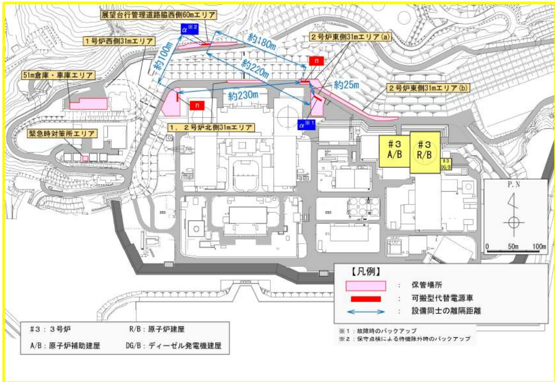
可搬型代替電源車の相互の離隔距離
