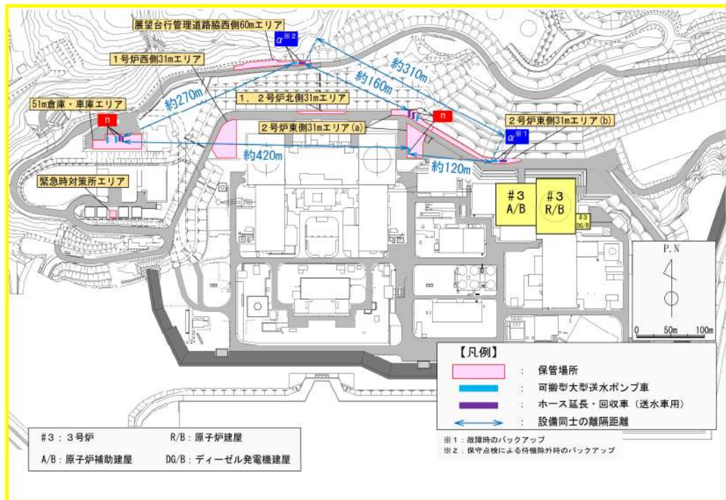
可搬型大型送水ポンプ車及びホース延長・回収車（送水車用）の相互の離隔距離 第3-3図 可搬型設備の配置(1/10)
