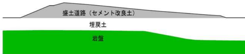
第6-28図 B-B' 概略断面図
