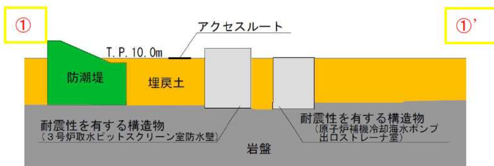
第 6-32 図 B エリア①-①' 地点断面図
