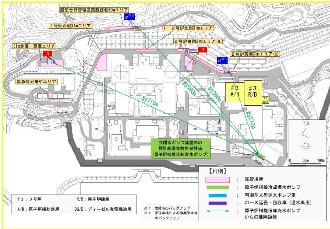
可搬型大型送水ポンプ車及びホース延長・回収車（送水車用）と原子炉補機冷却海水ポンプとの離隔距離
