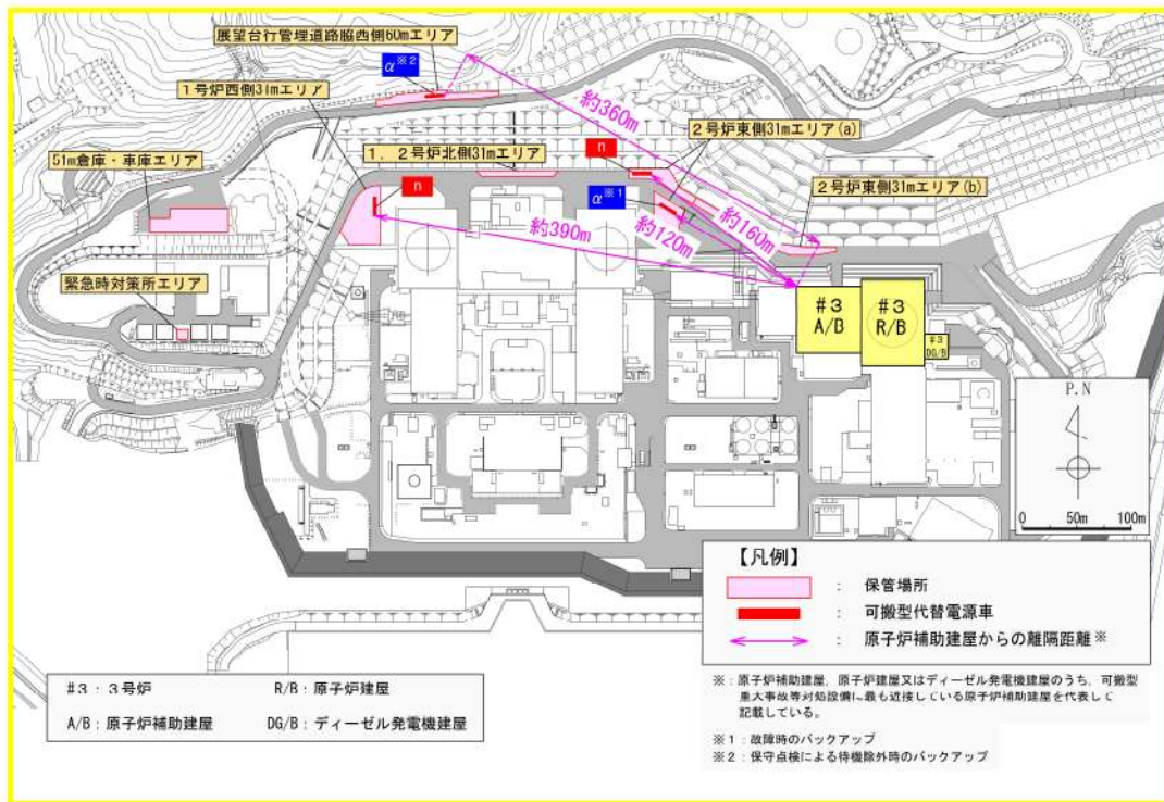
可搬型代替電源車と原子炉補助建屋との離隔距離
