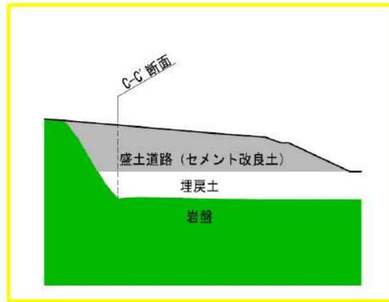
第6-27図 A-A' 概略断面図
