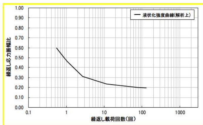
第 6-39 図 液状化パラメータ
