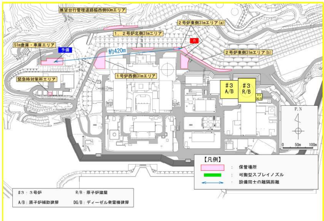
可搬型スプレインゾルの相互の離隔距離
