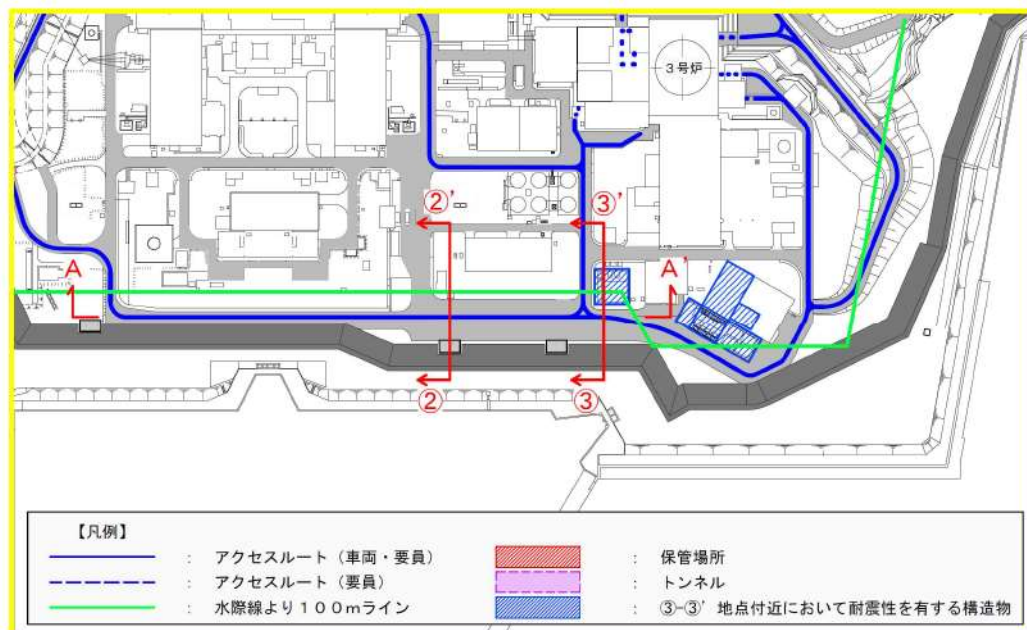
第6-35図 検討断面位置図
