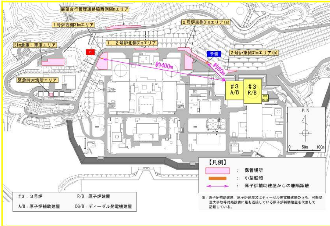
小型船舶と原子炉補助建屋との離隔距離
