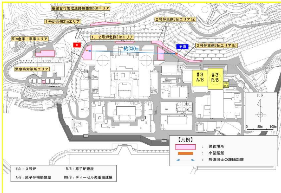
小型船舶の相互の離隔距離
