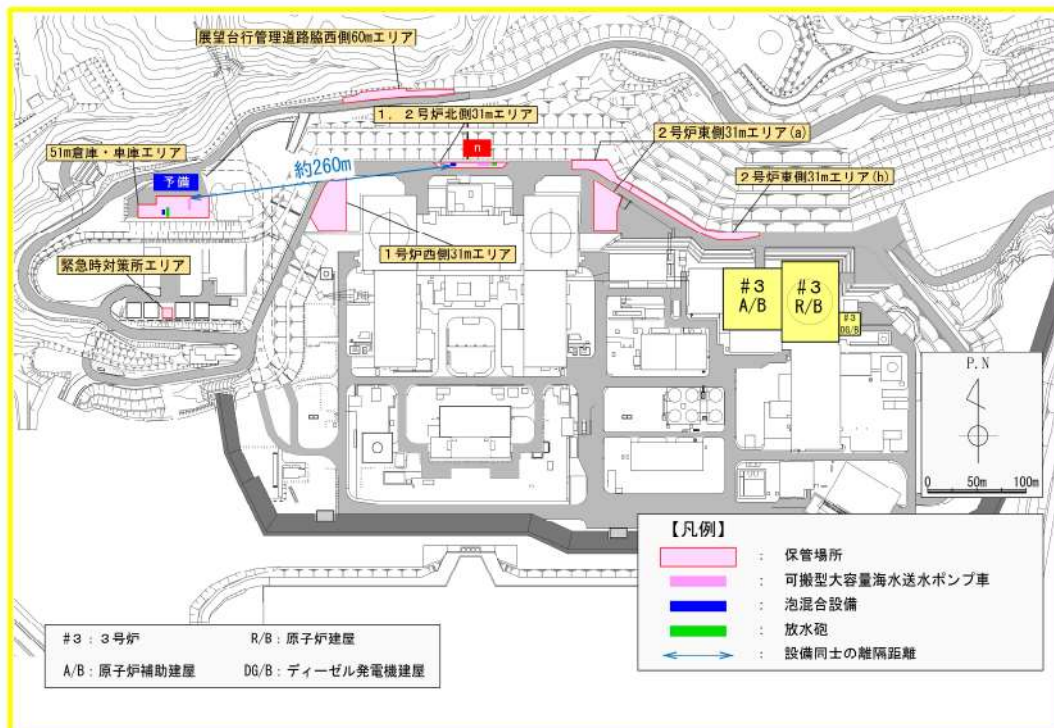
可搬型大容量海水送水ポンプ車，泡混合設備及び放水砲の相互の離隔距離
