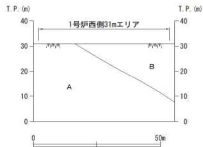
第 5-10 図 1号炉西側 31m エリア平面図及び地質断面図
