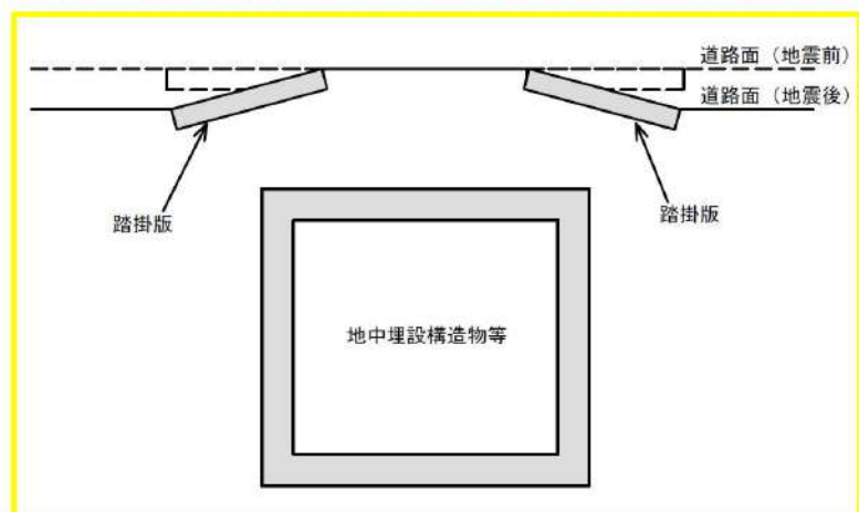
第6-21図 段差緩和対策概念図
