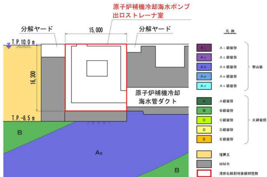
第 3.2-11 図 原子炉補機冷却海水ポンプ出口ストレナ室断面図
