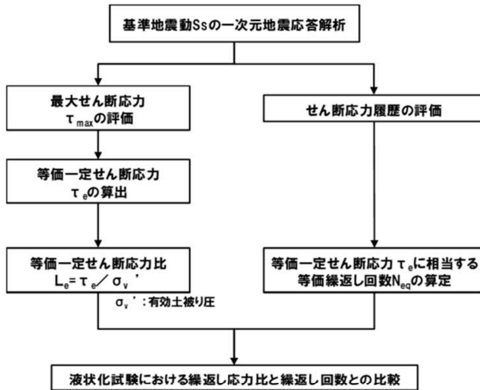
第 5.4-1 図 累積損傷度理論に基づく等価繰返し回数の評価フロー
