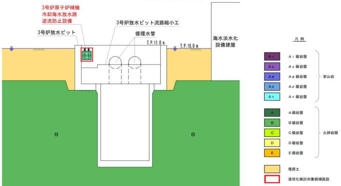
第 3.2-17 図 3 号炉原子炉補機冷却海水放水路逆流防止設備断面図
