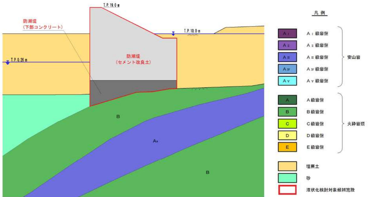
第 3. 2-14 図 防潮堤断面図
