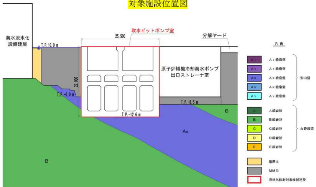
第 3.2-10 図 取水ピットポンプ室断面図
