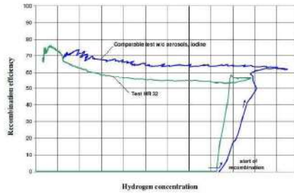
Fig. 5-6: Test HR-32: Recombination efficiency and onset of recombination for test HR 32 and for a comparable HR test without aerosols and iodine 上図の横軸はPAR入口水素濃度 (7&スケール6.0vol%, 1目盛0.5vol%(wet))、縦軸はPAR出入口間の水素除去効率を示している。
