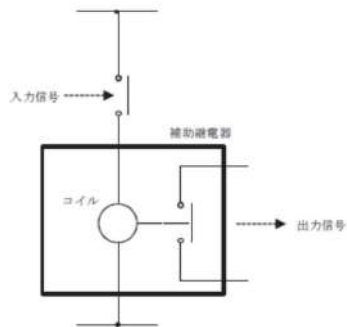
第2.7-3図 計測制御系との分離概念図
