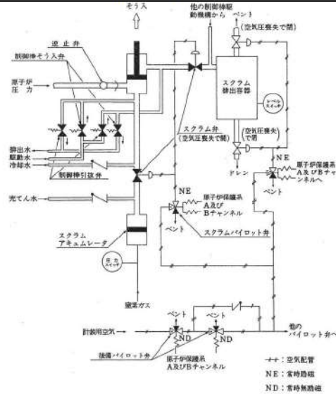
第6.6-2図 原子炉保護系及び制御機駆動系概観図
