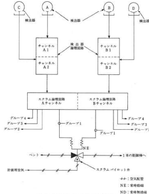
第6.6-3図 原子炉保護系作動回路概観図
