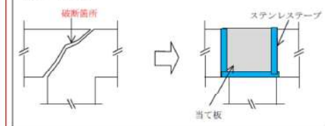
第2.1.2.3図 当て板による修復イメージ
