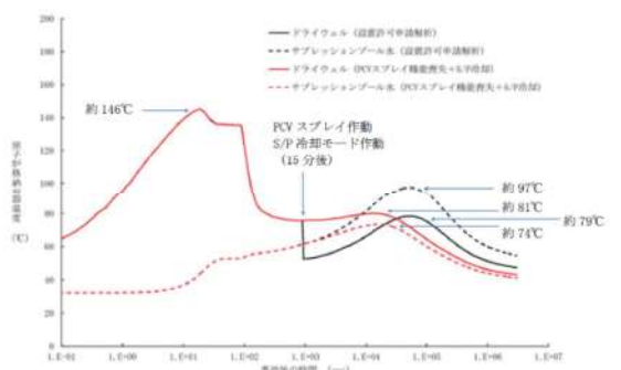
第2.1.3-2図 原子炉格納容器健全性解析結果 (‘レクション’冷却モード‘作動)
