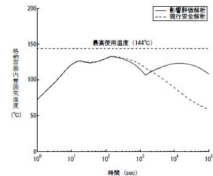
図1.5 スpray配管立上り部の全周破断を想定した場合の格納容器内雰囲気温度 (Spray流量として安全解析で考慮している値の20%の場合)
