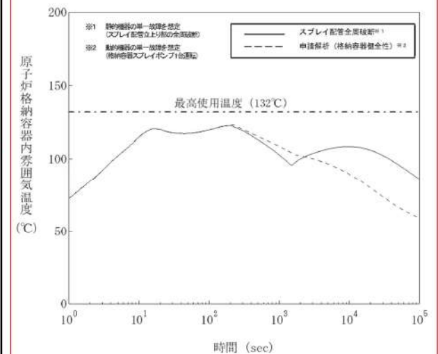
第2.1.3.11図 スpray立上り配管の全周破断を想定した場合の格納容器内雰囲気温度 (Spray流量として安全解析で考慮している値の36%の場合)
