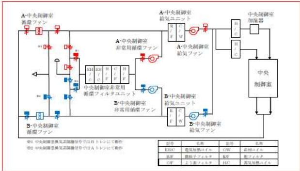
第9図 中央制御室換気空調設備の概要
