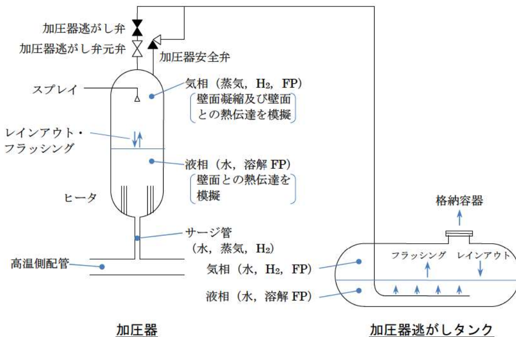
図 3.3-4 加圧器及び加圧器逃がしタンクモデル
