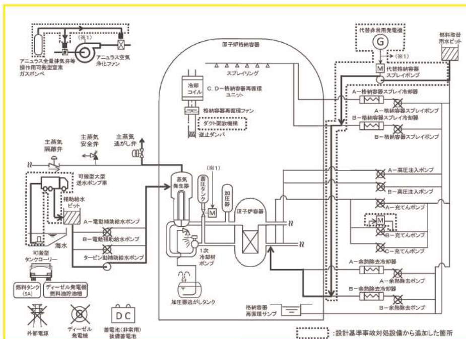
図 1 「外部電源喪失時に非常用所内交流電源が喪失し、原子炉補機冷却機能の喪失及び RCP シール LOCA が発生する事故」の重大事故等対策の概略系統図 (2次冷却系強制冷却及び代替炉心注水)
