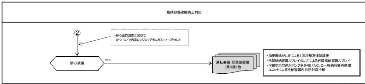
第 7.1.3.2 図 「原子炉補機冷却機能喪失」の対応手順の概要 (判定プロセス) (2 / 2)
