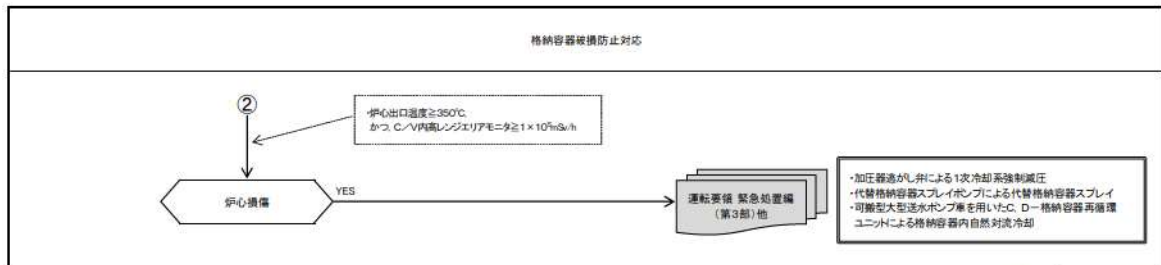
第7.1.2.2図 「全交流動力電源喪失」の対応手順の概要 (判定プロセス) (2/2)
