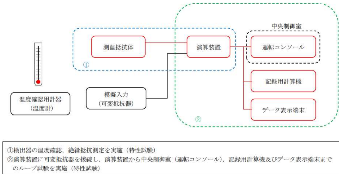
第 13 図 温度計の試験及び検査
