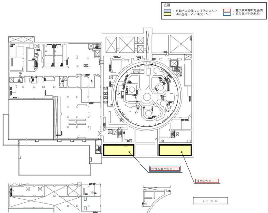
第 2 1 図 代替炉心注水（代替格納容器スプレイポンプ）に関する機器の配置（2 / 2）
