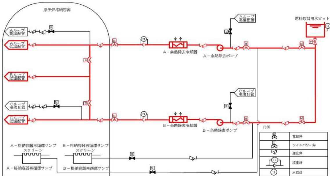
第18-2図 余熱除去ポンプによる炉心注水 系統概要図
