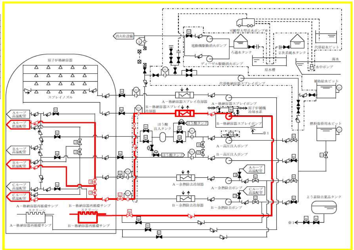
第24-1図 代替再循環運転（B-格納容器スプレイポンプ）系統概要図
