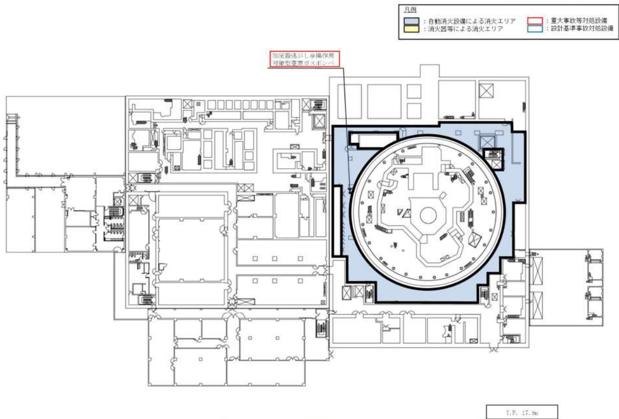
第1図 加圧器逃がし弁の機能回復に関する機器の配置
