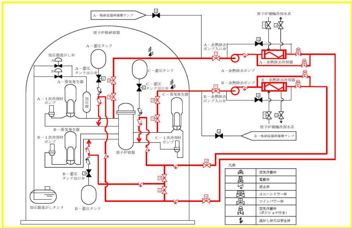
1次冷却系のフィードアンドブリード（余熱除去設備による冷却）
