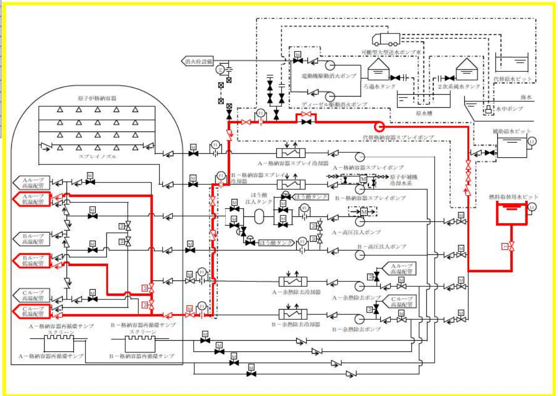
第20-1図 代替炉心注水（代替格納容器スプレイポンプ）系統概要図
