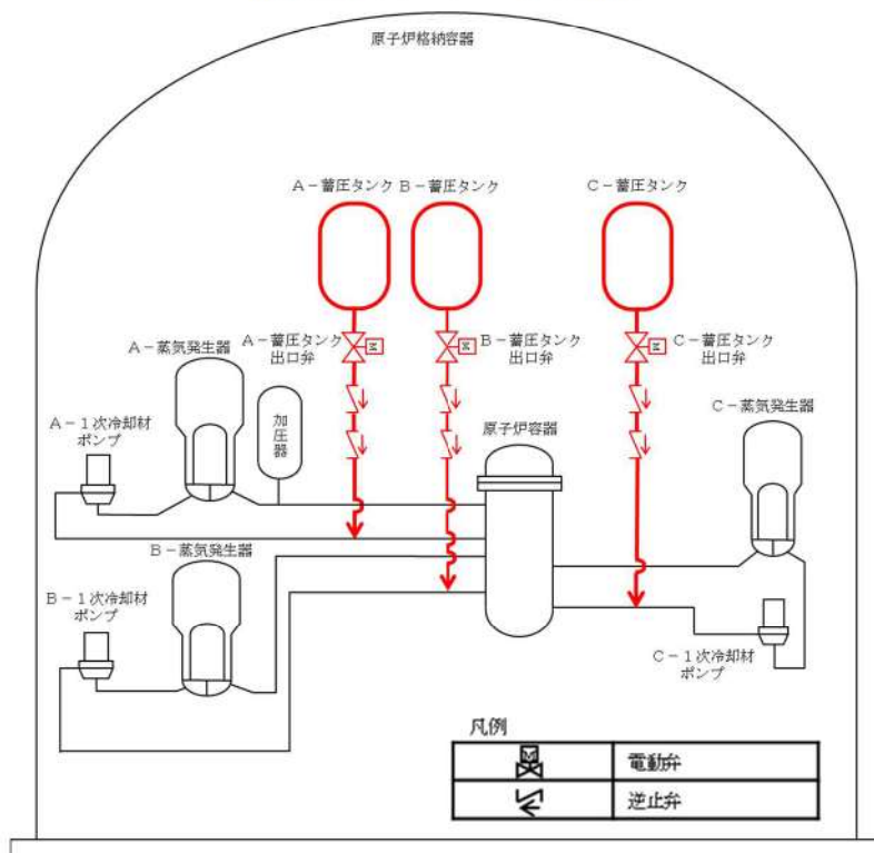
(蓄圧注入系による注水)
