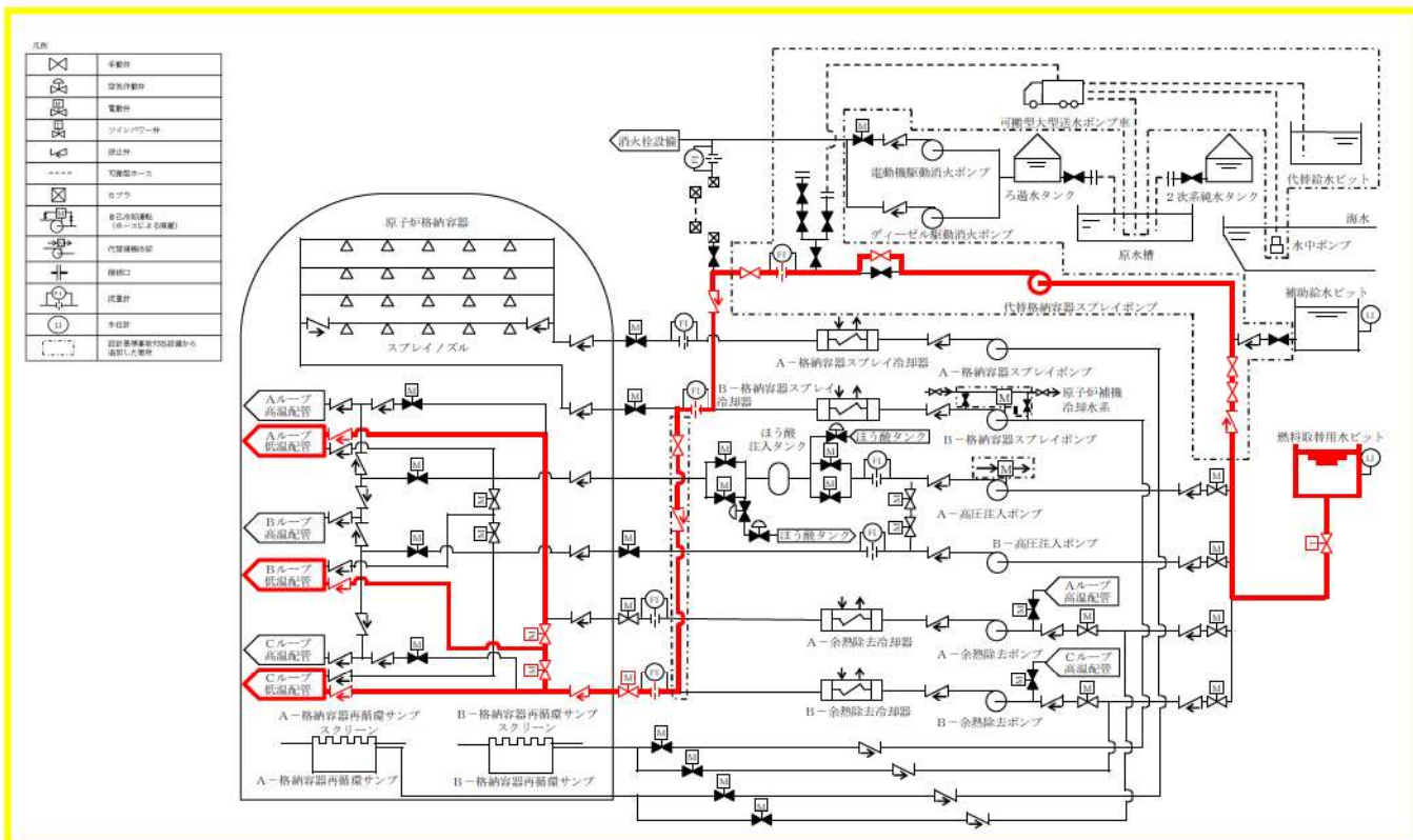
代替炉心注水 (代替格納容器スプレイポンプ)
