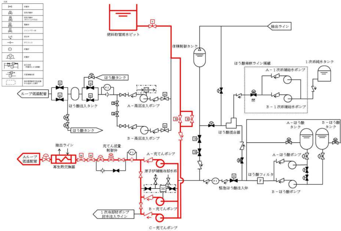
第 10-2 図 ほう酸水注入（燃料取替用水ピット→充電ライン） 系統概要図
