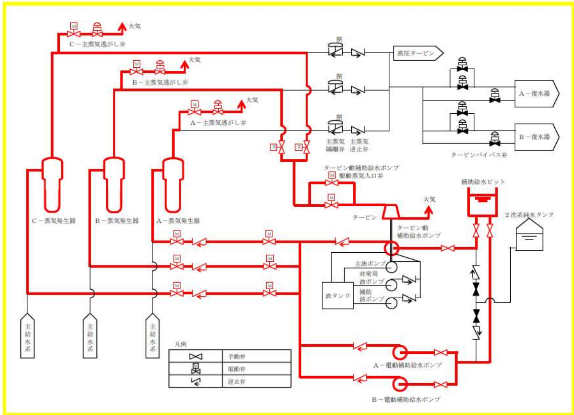
第14-1図 蒸気発生器2次側からの除熱 系統概要図
