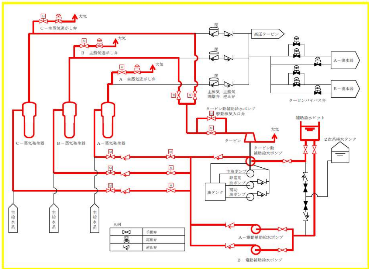
第32-1図 蒸気発生器2次側からの除熱 系統概要図
