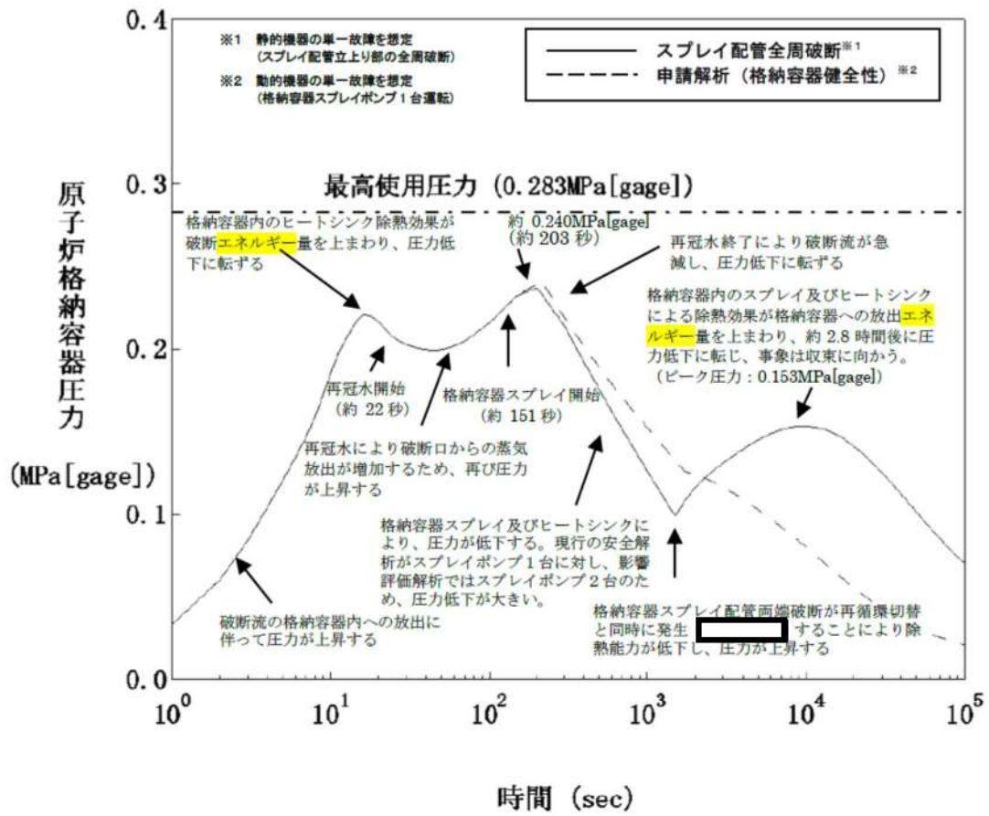
第2.1.3.10図 スプレイ立上り配管の全周破断を想定した場合の格納容器内圧力 (スプレイ流量として安全解析で考慮している値の36%の場合)
