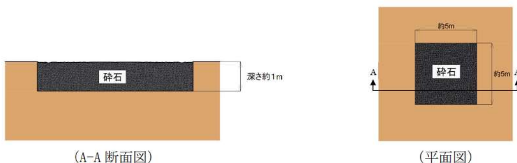
※：縦，横，深さについては，今後の検討により変更となる可能性がある。 段差復旧用の碎石の配備イメージ
