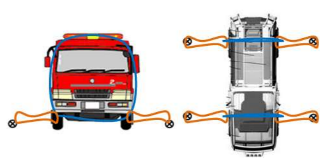
図2 車両の固縛イメージ
