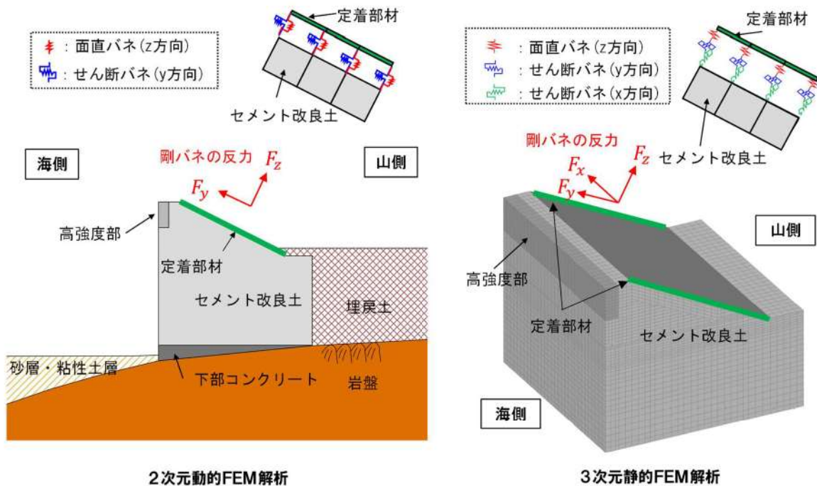
第 7-25 図 解析①から算出する剛バネの反力 ( F_x, F_y, F_z )
