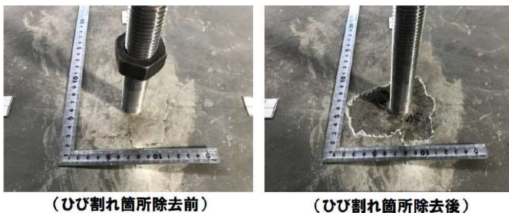
第 7-59 図 引張試験1-4 引張試験後の状況写真
