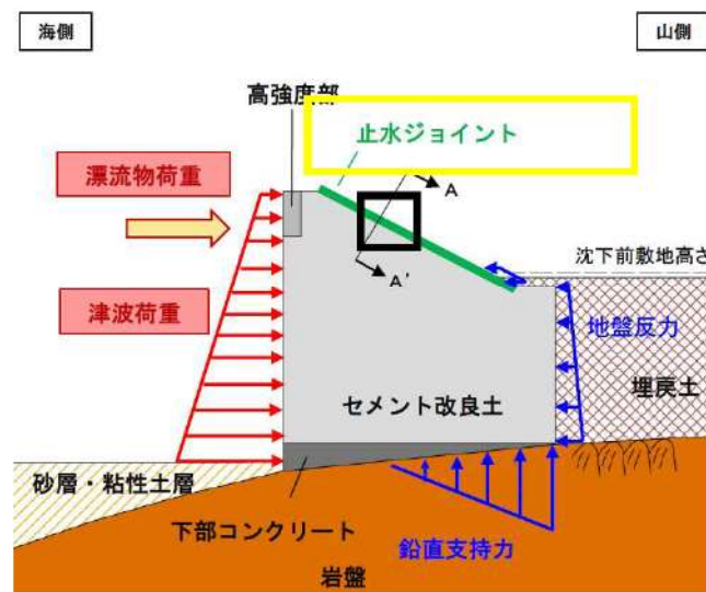
第 7-12 図 津波時に防潮堤に生じる外力
