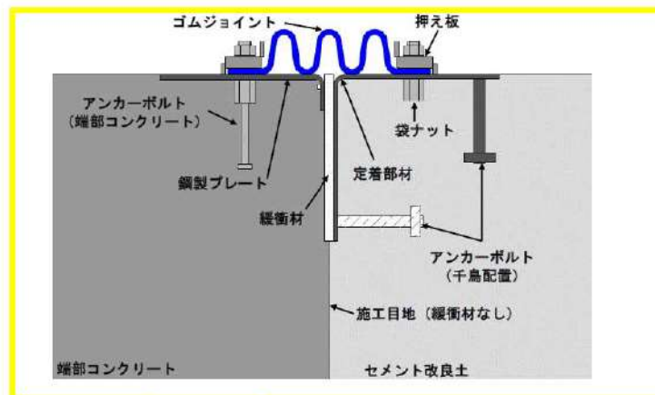
止水ジョイント設置概要（A-A' 断面）
