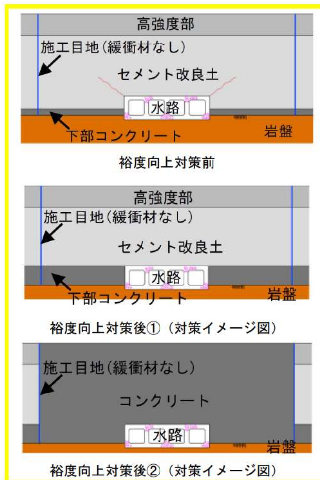
第 5-48 図 取水路及び放水路が横断する範囲の防潮堤の裕度向上対策のイメージ図
