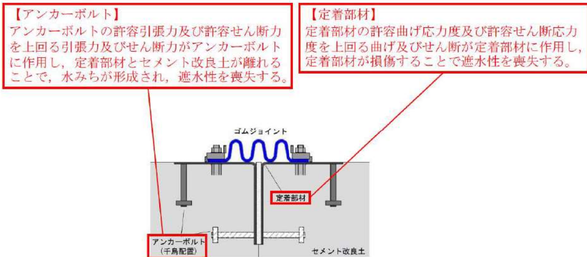
第 7-29 図 止水ジョイントの構造上の弱部となる箇所（地震時）
