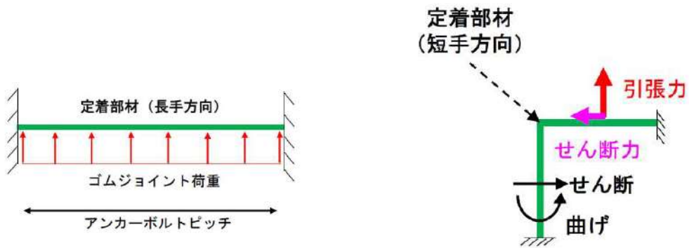
定着部材長手方向のモデル
