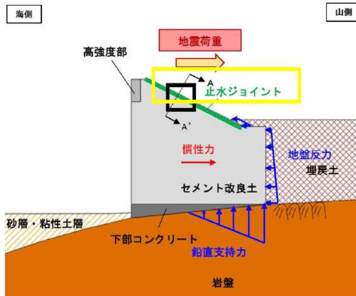
第 7-9 図 地震時に防潮堤に生じる外力
