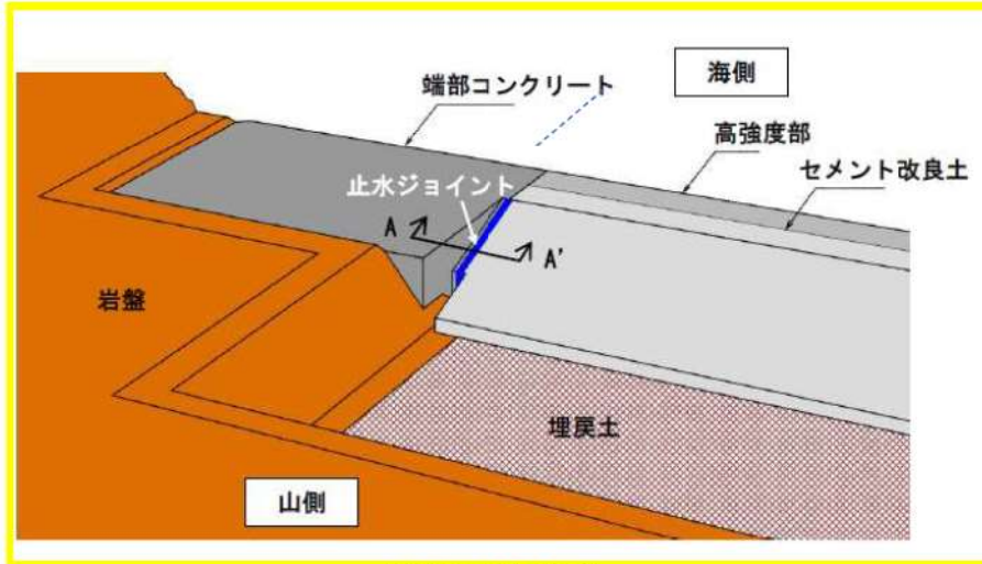
構造境界部の概要
