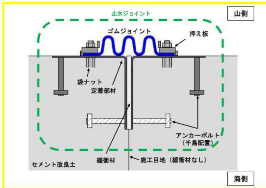
第 7-2 図 防潮堤（標準部）の止水ジョイントの設置概要（A-A' 断面）
