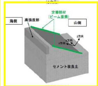
解析モデルイメージ図
