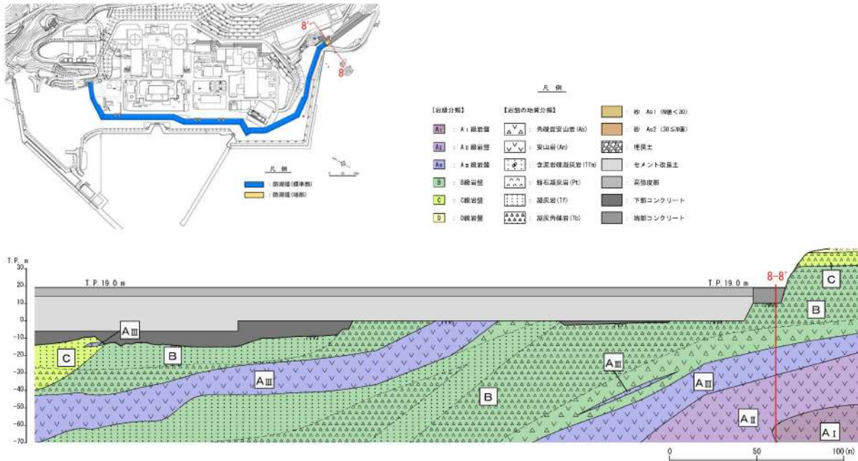
第 6-5 図 防潮堤（端部）の地質縦断面図
