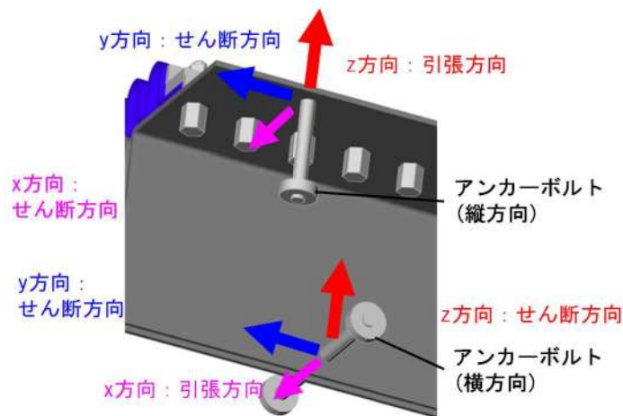
第 7-27 図 アンカーボルトに作用した各方向（x方向，y方向，z方向）の力に対する抵抗方向
