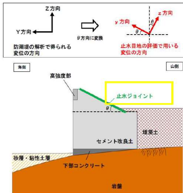
第 7-23 図 防潮堤の法面傾斜角を考慮した変位算出のイメージ図
