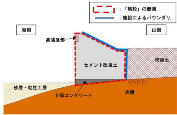
防潮堤断面図(既設護岸及び埋戻土等がない状態)
