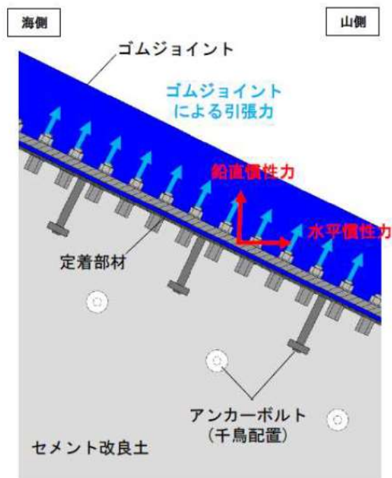
第 7-17 図 重疊時にゴムジョイントの張力及び慣性力により定着部材及びアンカーボルトに生じる外力
