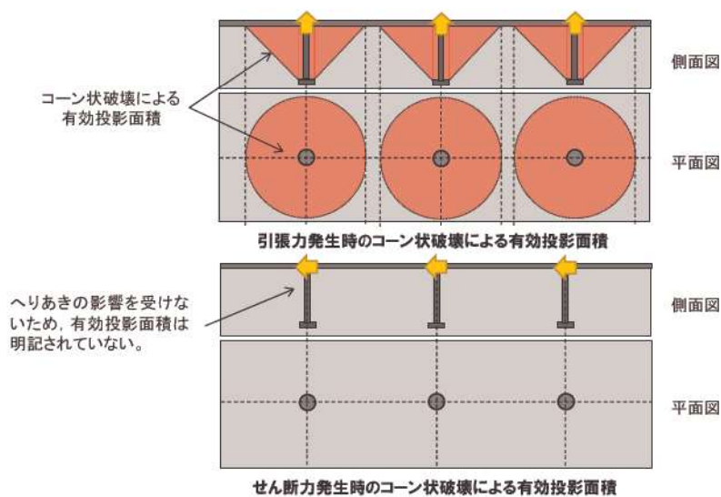
第 7-32 図 「各種合成構造設計指針」におけるアンカーボルトのコーン状破壊による有効投影面積
