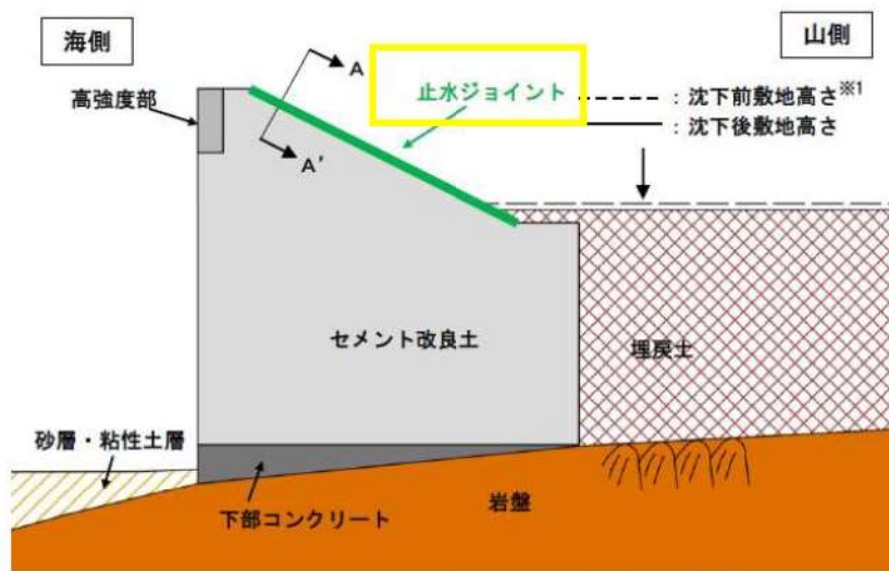
第 7-1 図 防潮堤（標準部）の目地止水ジョイント設置位置
