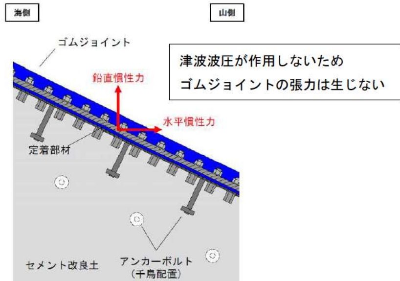
第 7-11 図 地震時にゴムジョイントの張力及び慣性力により定着部材及びアンカーボルトに生じる外力
