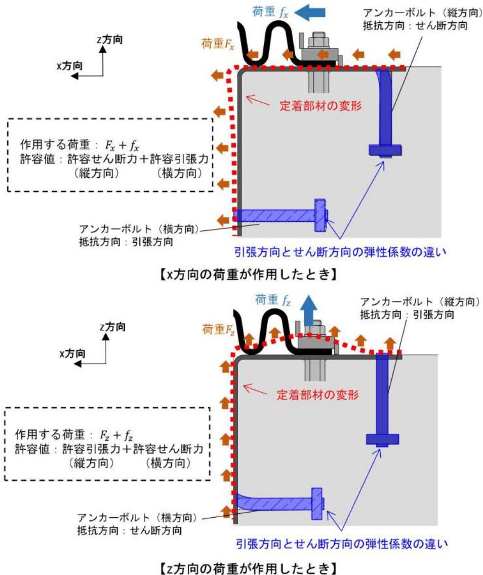
第 7-28 図 各方向の荷重がアンカーボルトに作用する際のイメージ図
