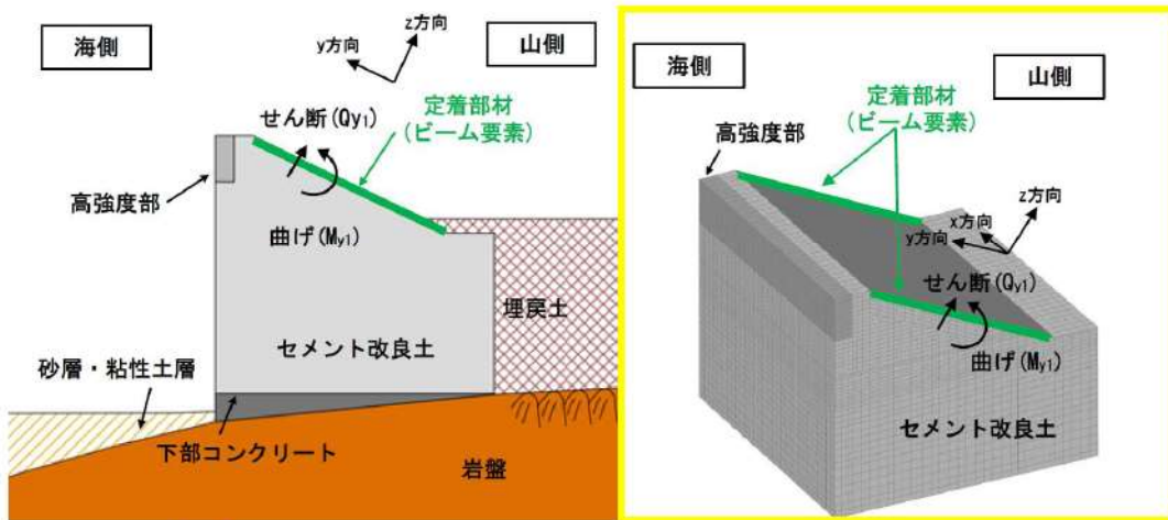
第 7-21 図 解析①のモデルと曲げ及びせん断のイメージ図 (左：地震時及び重畳時，右：津波時)
