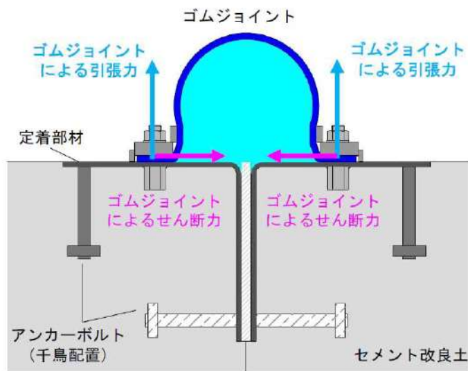
第 7-16 図 重畳時にゴムジョイントの張力により定着部材及びアンカーボルトに生じる外力 (A—A' 断面)
