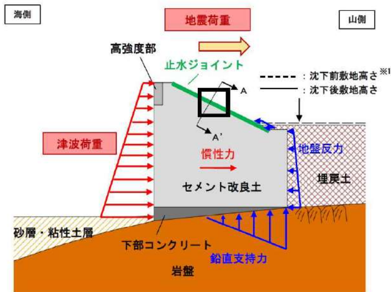
第 7-15 図 重畳時に防潮堤に生じる外力
