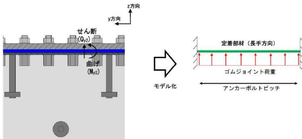
第 7-22 図 ゴムジョイントの張力により定着部材（長手方向）に生じる曲げ及びせん断の算出イメージ図（解析②）
