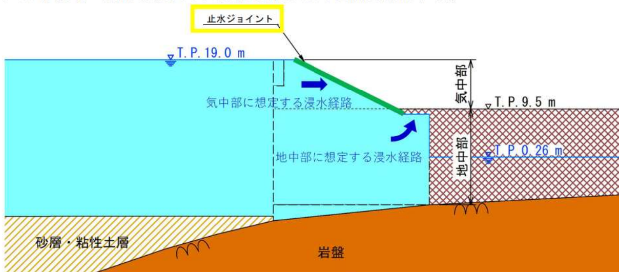
第 7-40 図 施工目地に津波の水が滞水した場合の浸水経路
