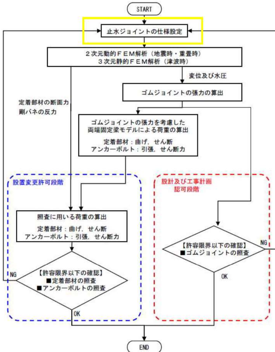
第 7-7 図 定着部材，アンカーボルト及びゴムジョイントの照査の流れ
