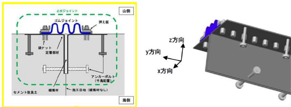
第 7-8 図 アンカーボルトの配置イメージ図
