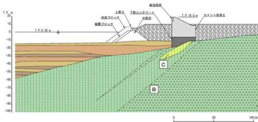
第 1-11 図 地質縦断図 (2-2')
