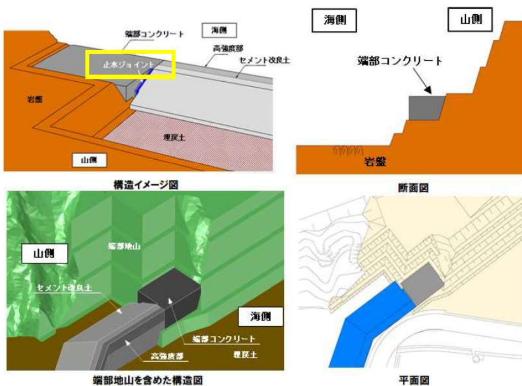
第 6-1 図 防潮堤（端部）の構造概要図
