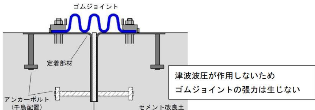
第 7-10 図 地震時にゴムジョイントの張力により定着部材及びアンカーボルトに生じる外力 (A—A' 断面)
