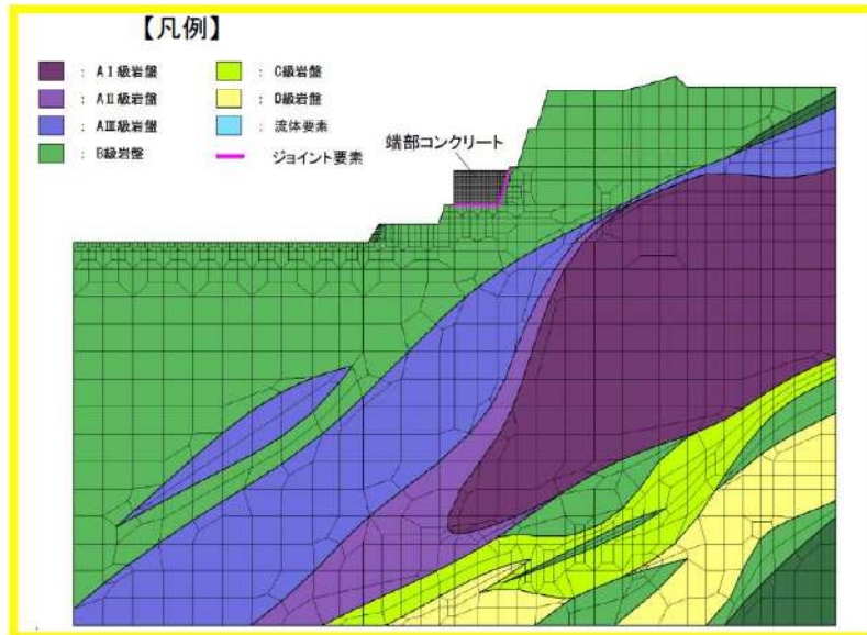
第 6-9 図 防潮堤（端部）の解析モデル
