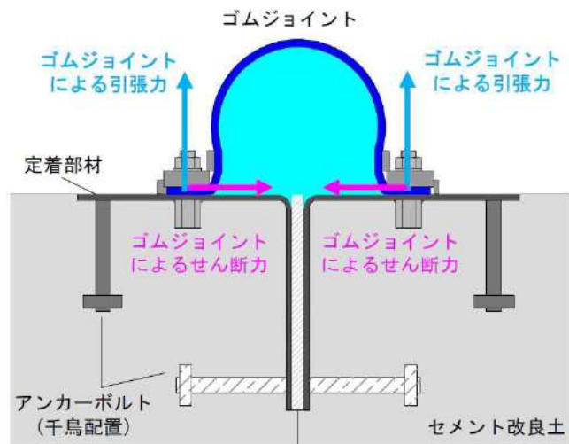
第 7-13 図 津波時にゴムジョイントの張力により定着部材及びアンカーボルトに生じる外力 (A—A' 断面)
