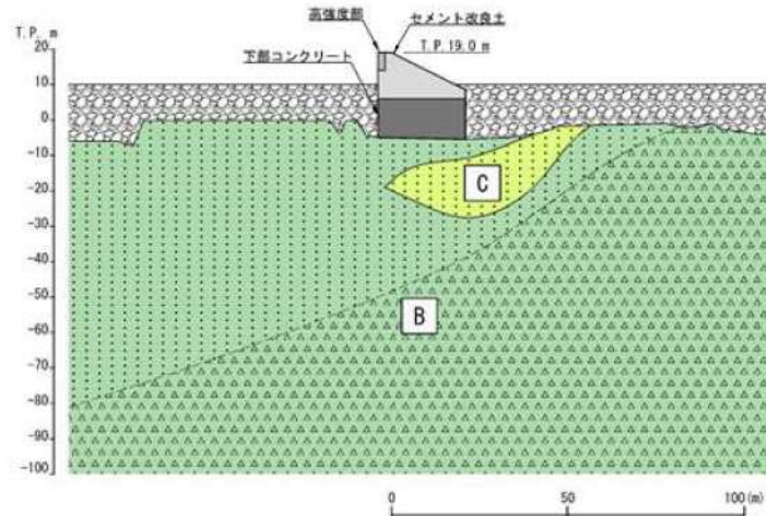
第 1-10 図 地質縦断図 (1-1')
