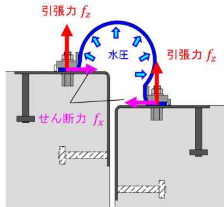
第 7-26 図 ゴムジョイントの張力により定着部材に作用する引張力 f_z ，せん断力 f_x
