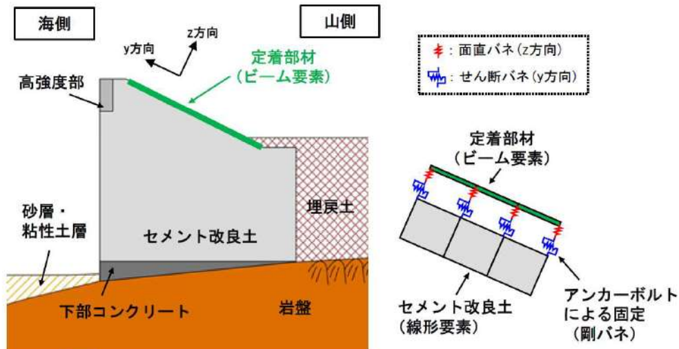
第7-18図 2次元動的FEM解析による解析モデルのイメージ図 （地震時及び重畳時の解析①）
