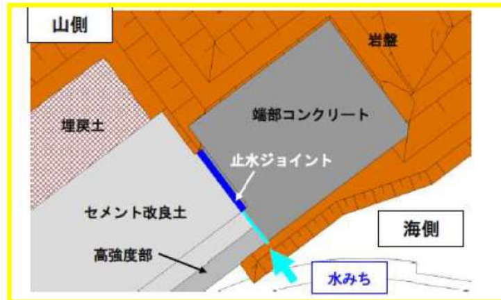
水みちのイメージ図（平面図）
