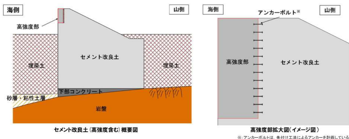
第 5-31 図 防潮堤（標準部）のセメント改良土及び高強度部の概略図
