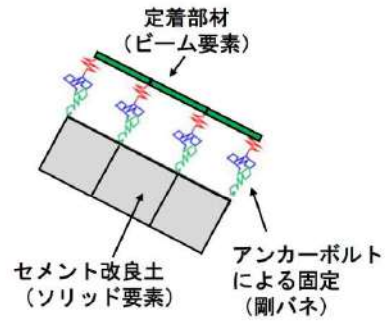
第 7-19 図 3次元静的FEM解析による解析モデルのイメージ図 (津波時の解析①)
