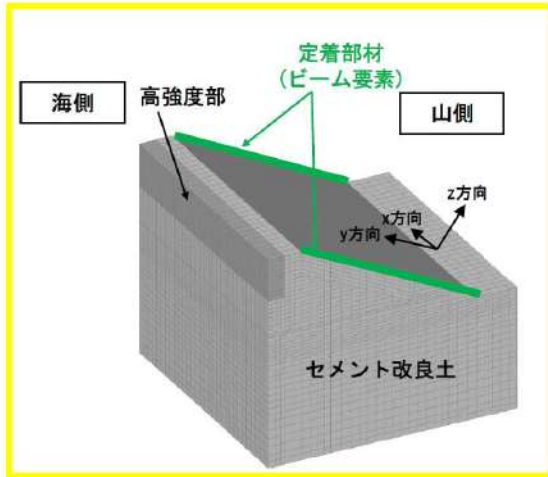
第 7-19 図 3次元静的FEM解析による解析モデルのイメージ図 (津波時の解析①)
