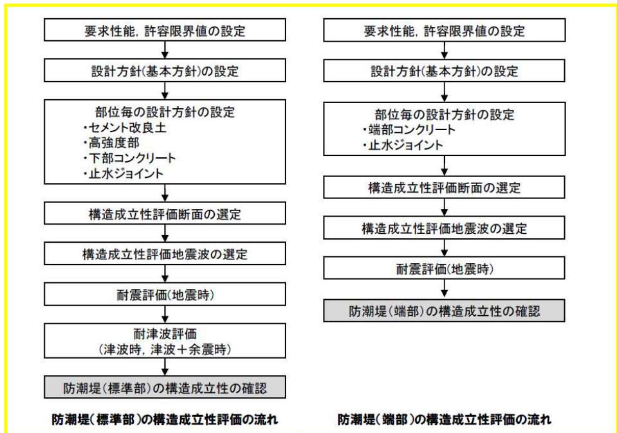
第 8-3 図 防潮堤の構造成立性評価の流れ
