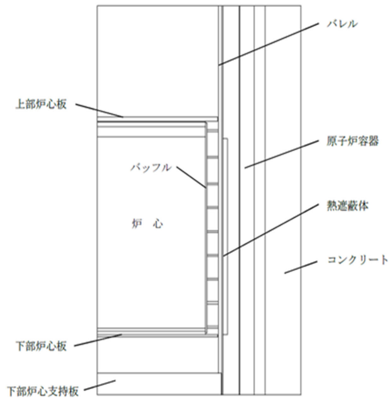
図2 計算モデル図[(R, Z)形状]
