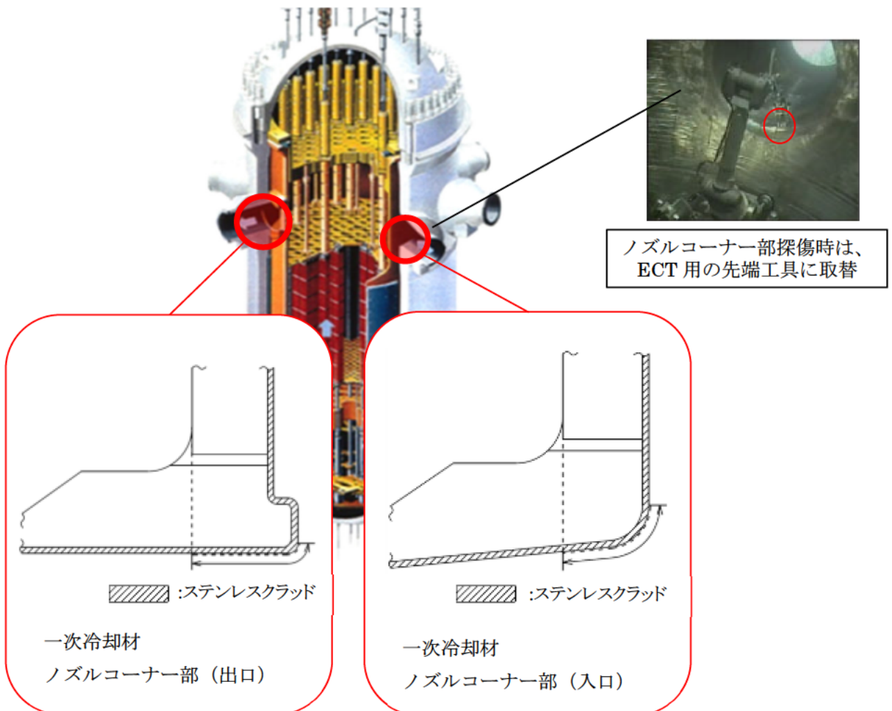
図 3.2.2.1 試験対象（一次冷却材ノズルコーナー部）
