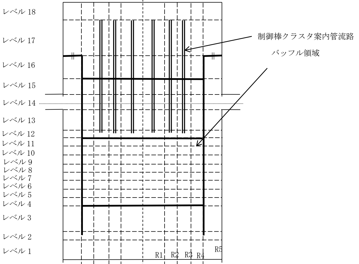
図2 PWR 3 ループプラントの原子炉容器内の炉心領域を除くセル分割
