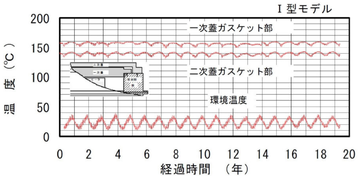
図6 金属ガスケット(二次蓋)の長期密封性能試験結果(眼鏡型) (2)
