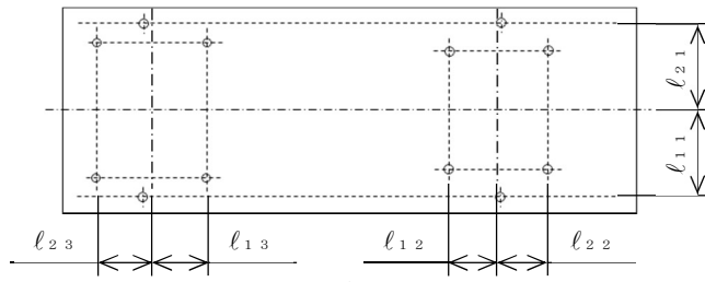
A~A矢视图
