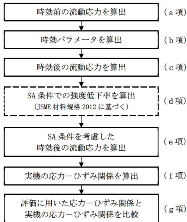
図1 JSME維持規格2016/2019を用いた応力-ひずみ関係の妥当性確認フロー（一部、JSME材料規格2012に基づく）
