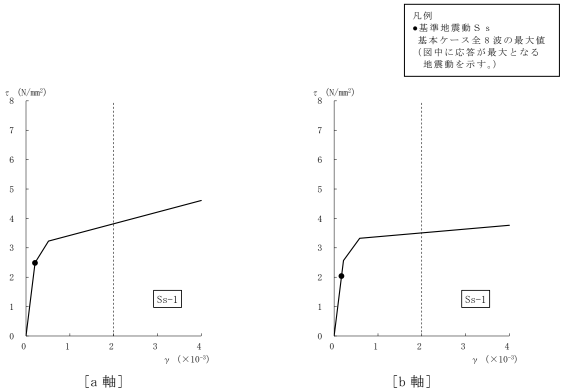
図 4-14 せん断スケルトン曲線上の最大応答値 (基準地震動 S s , NS 方向, B2F) (4/4)
