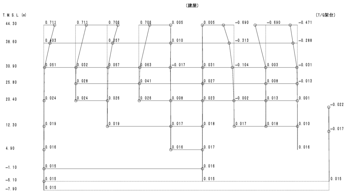
図 4-1 刺激関数図 (Ss-1, EW 方向) (3/4)
