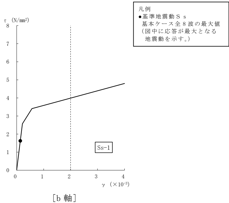
図 4-14 せん断スケルトン曲線上の最大応答値 (基準地震動 S s , NS 方向, MB2F) (3/4)
