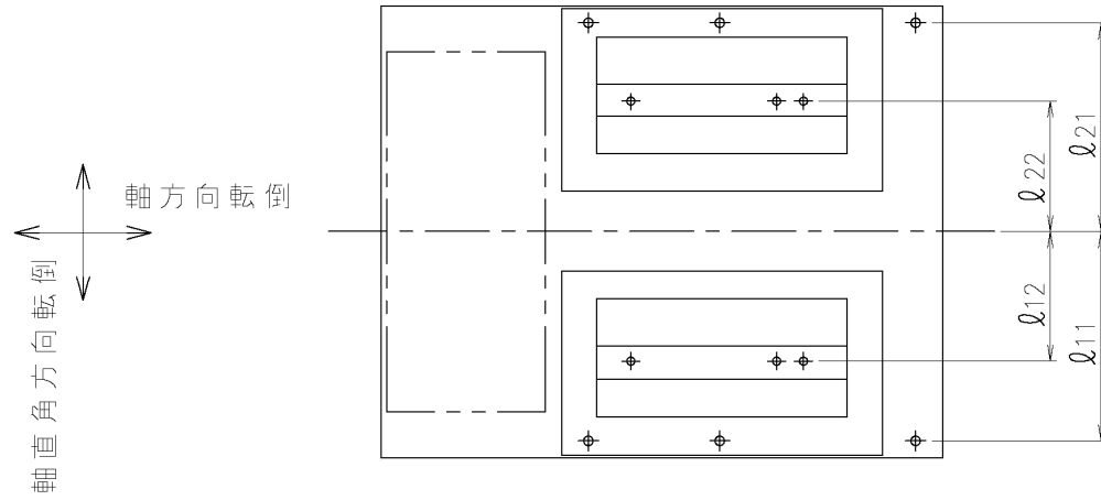
A~A矢視図
