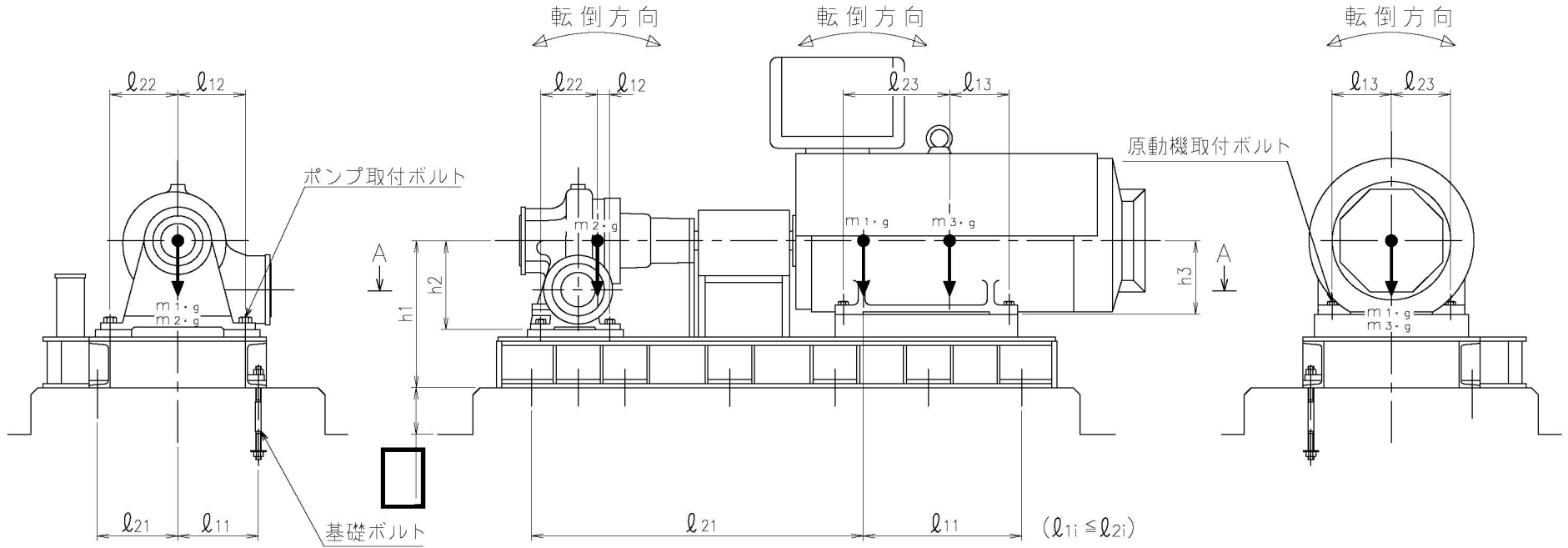
A~A矢視図
