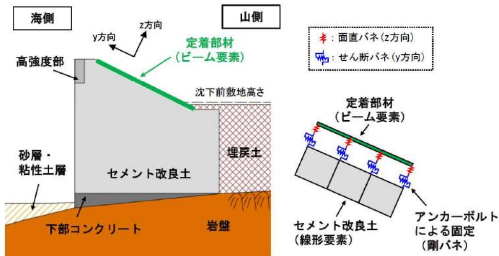
第7-21図 2次元動的FEM解析による解析モデルのイメージ図 （地震時及び重畳時の解析①）
