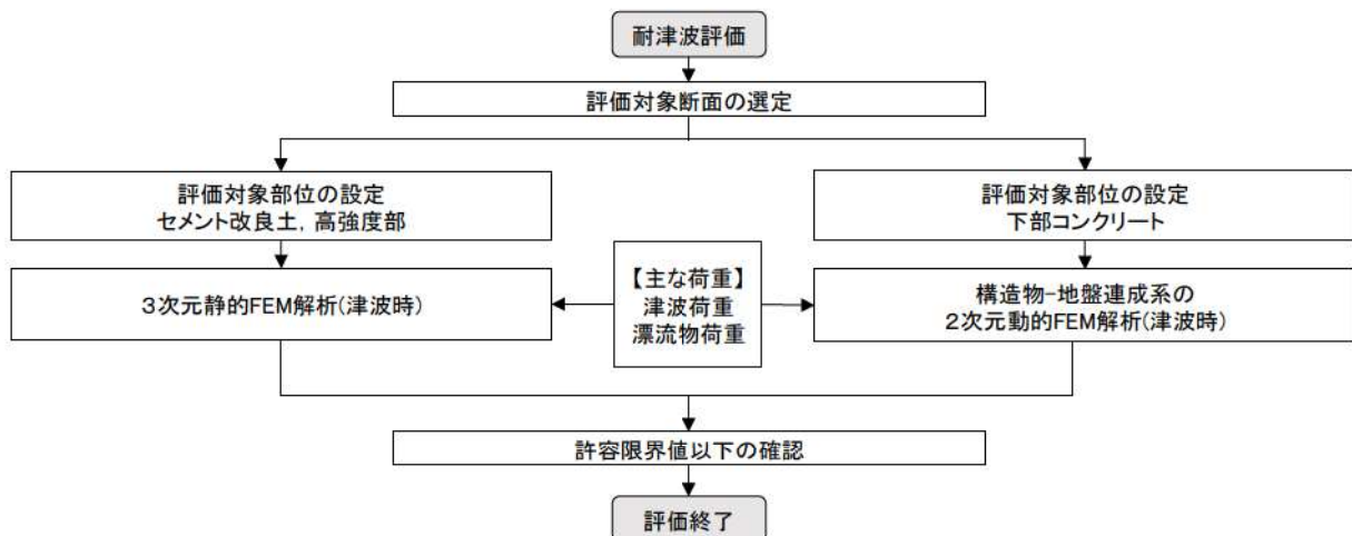
第 5-24 図 設計フロー
