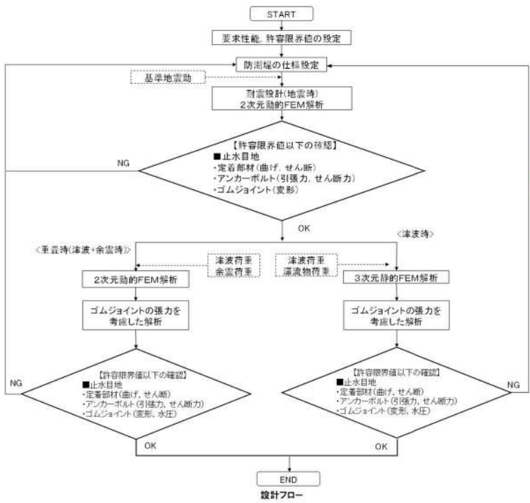
第 7-9 図 止水目地に関する解析の流れ
