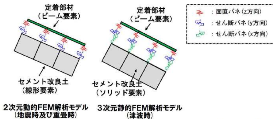
第 7-28 図 セメント改良土と定着部材の境界部のモデル化イメージ図（解析①）
