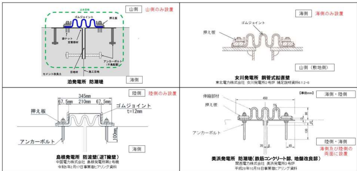
第 7-34 図 止水目地の構造概要 (泊発電所，女川発電所，島根発電所，美浜発電所)
