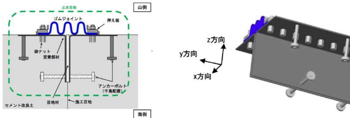
第 7-11 図 アンカーボルトの配置イメージ図
