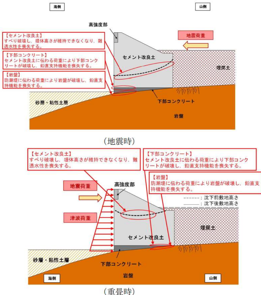
第 5-32 図 防潮堤（標準部）の構造上の弱部（地震時，重畳時）
