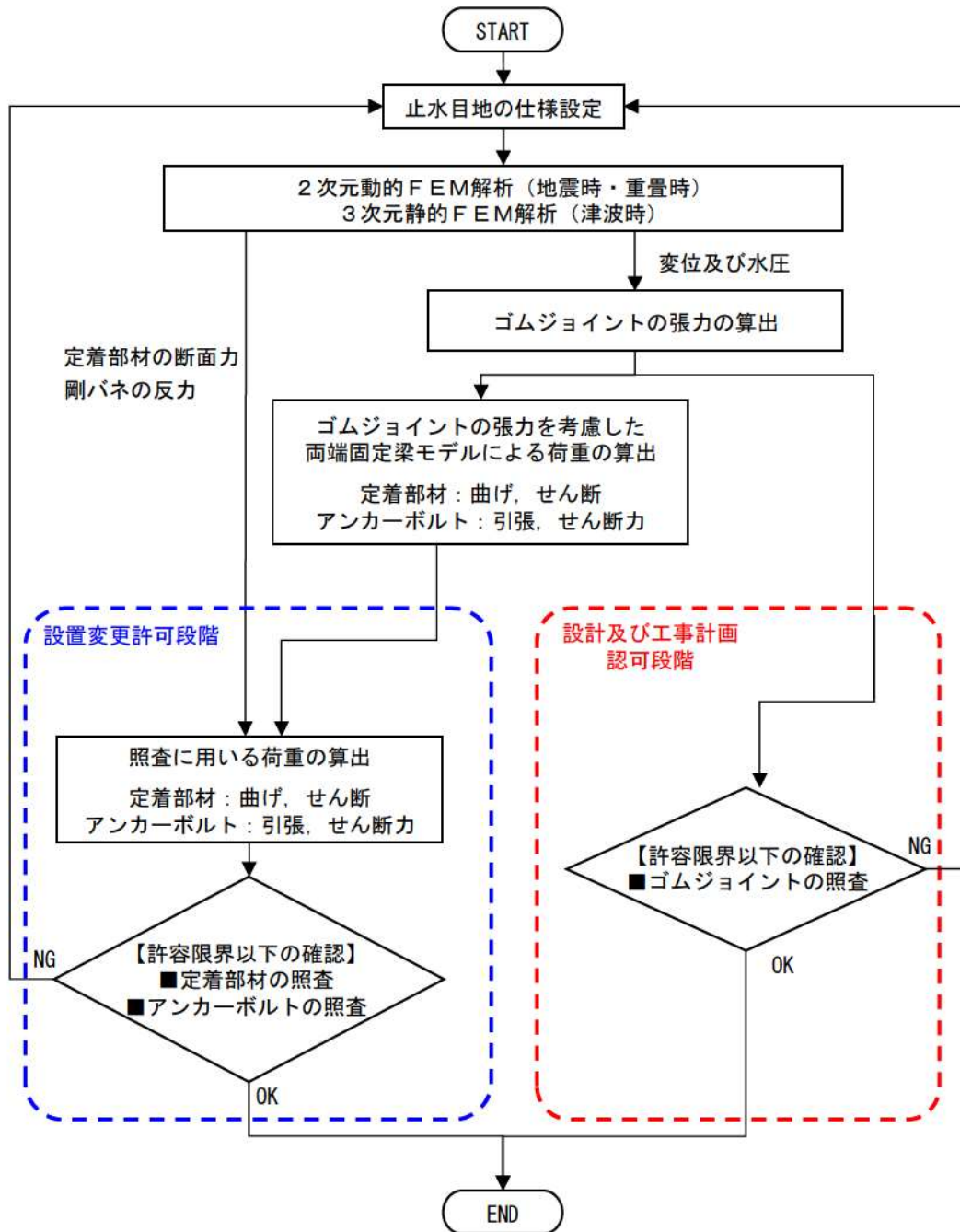
第 7-10 図 定着部材，アンカーボルト及びゴムジョイントの照査の流れ
