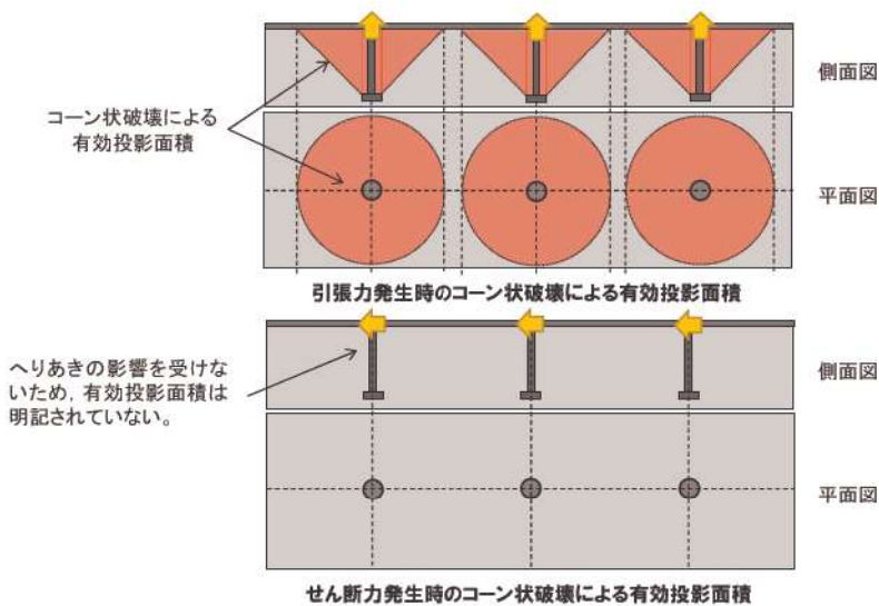
第 7-35 図 「各種合成構造設計指針」におけるコーン状破壊による有効投影面積の考え方
