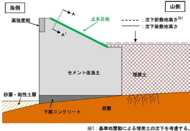
第 7-4 図 防潮堤（標準部）の止水目地設置位置
