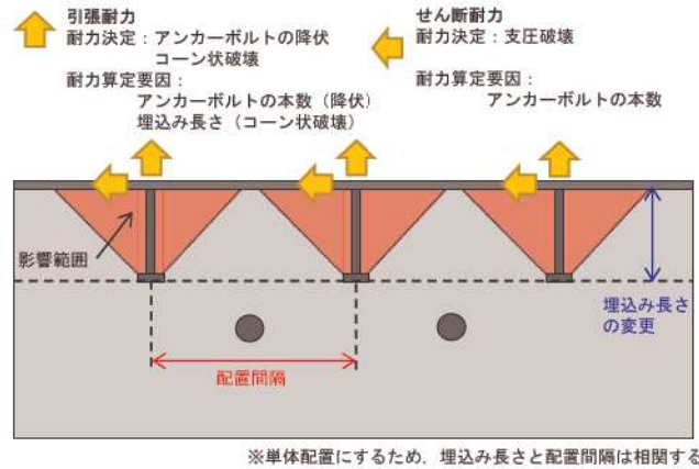
第 7-75 図 アンカーボルトの埋込み長さと配置間隔の考え方
