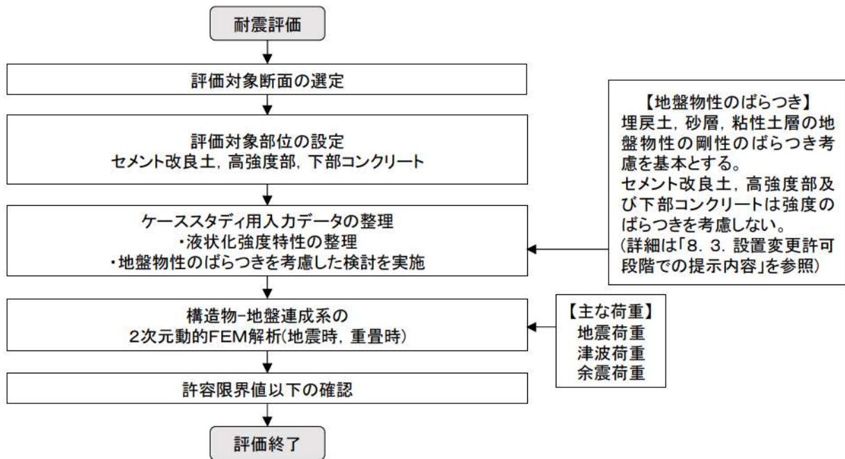
第 5-21 図 設計フロー
