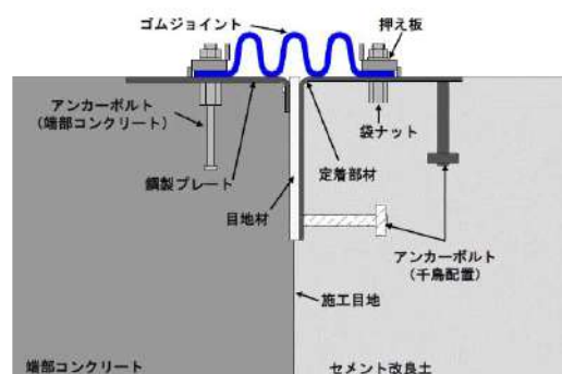
止水目地設置概要（端部）
