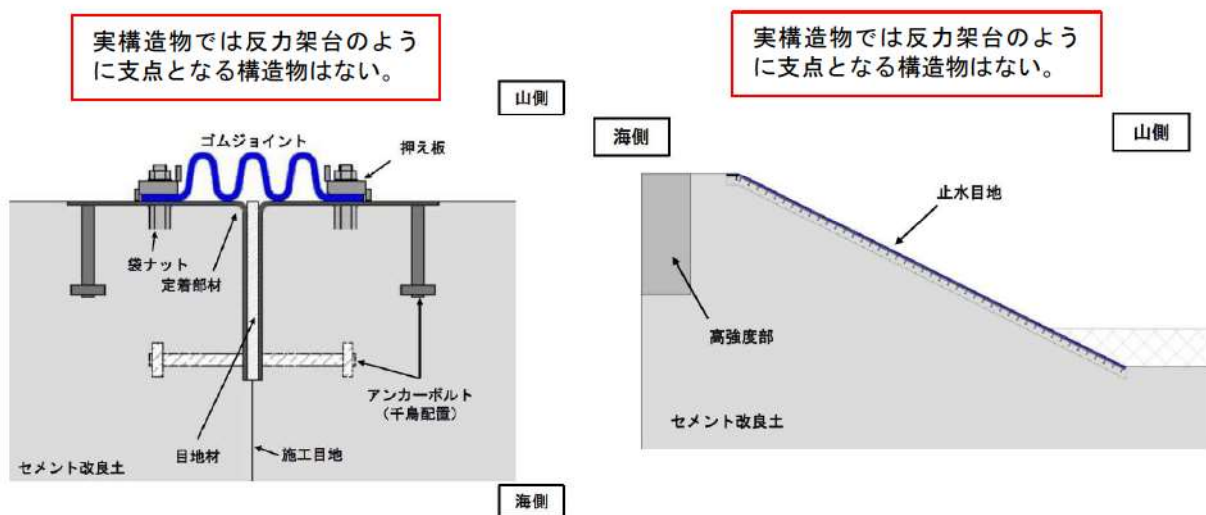
第 7-70 図 防潮堤イメージ図
