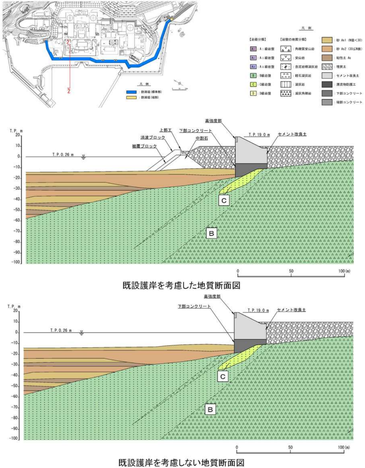
第 5-46 図 既設護岸の考慮しない地質断面図
