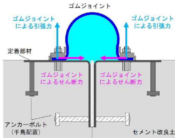
第 7-19 図 重畳時にゴムジョイントの張力により定着部材及びアンカーボルトに生じる外力 (A—A' 断面)
