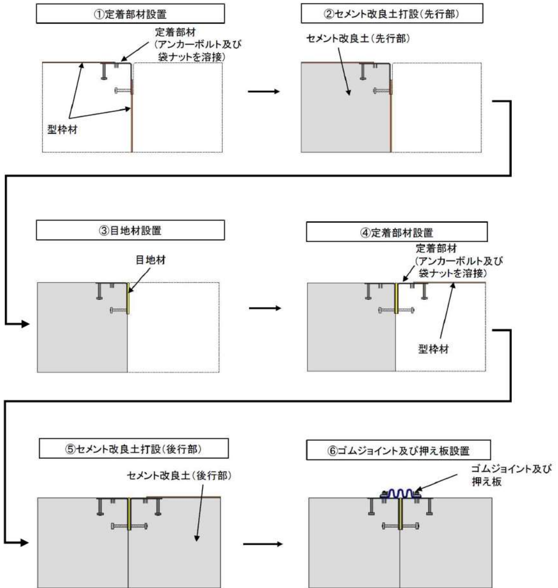
第 7-8 図 止水目地の施工方法
