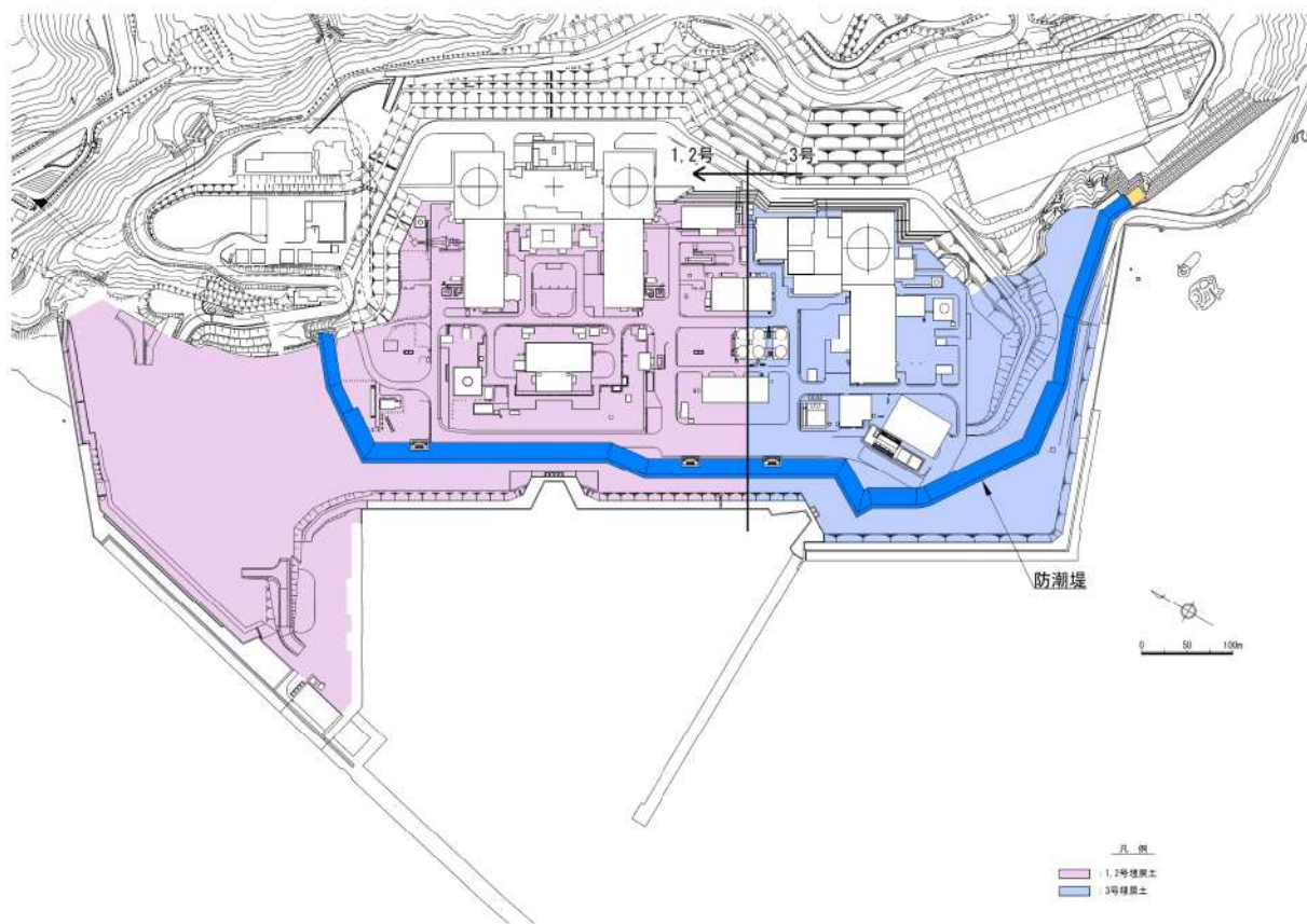
第 5-8 図 敷地の被覆層 平面図
