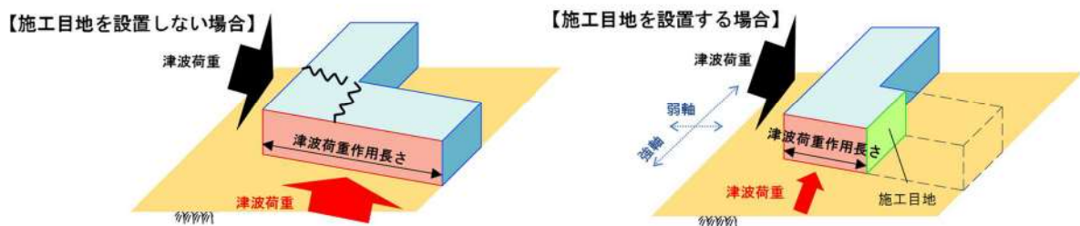
第5-40図 水平2方向荷重による損傷モードのイメージ
