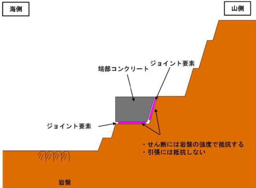
第 6-10 図 境界面のジョイント要素のイメージ図
