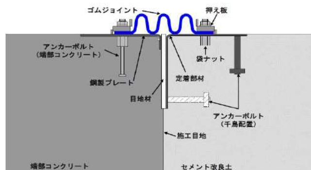
第 6-2 図 止水目地の設置概要
