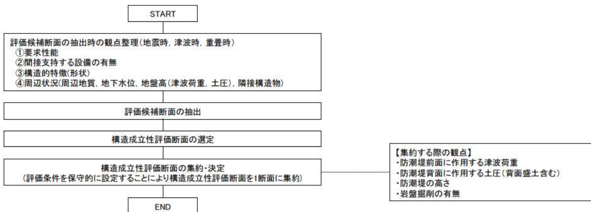
第 5-34 図 構造成立性評価断面選定フロー
