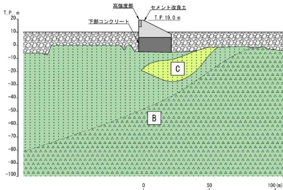
第 5-13 図 防潮堤（標準部）の地質横断面図（1-1'）
