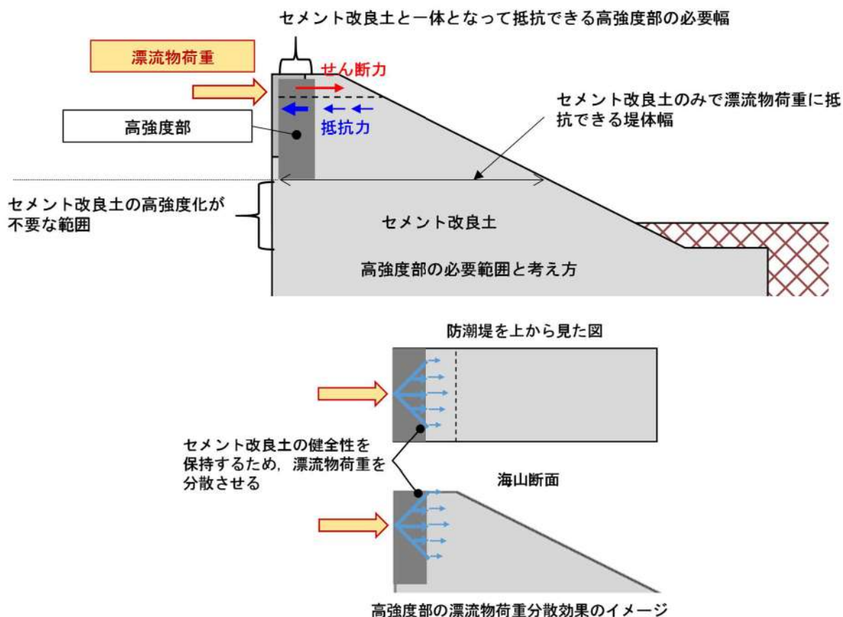
第 5-28 図 高強度部に期待する効果及び効果を発揮するためのメカニズム
