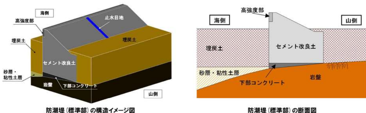
第 5-1 図 防潮堤（標準部）の構造概要
