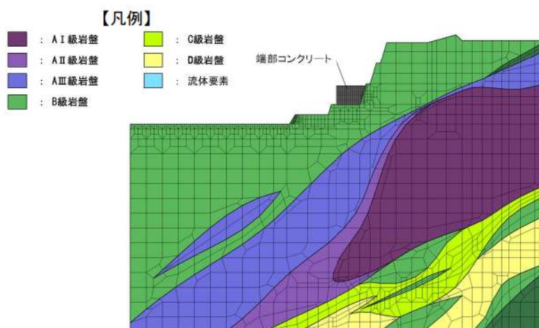
第 6-9 図 防潮堤（端部）の解析モデル
