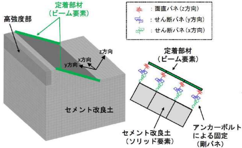
第 7-22 図 3次元静的FEM解析による解析モデルのイメージ図 (津波時の解析①)
