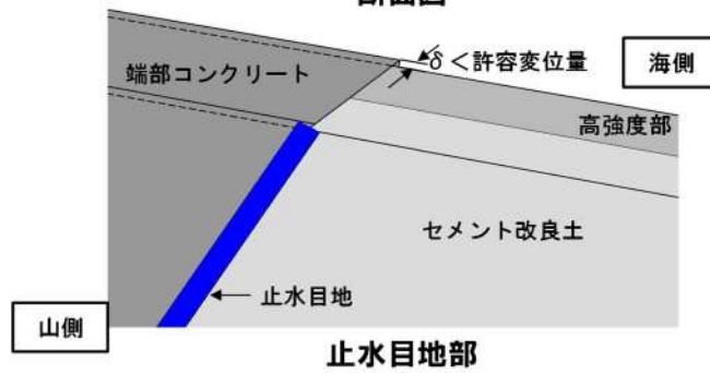
第 6-11 図 岩盤の押し出しによる端部コンクリートへの影響
