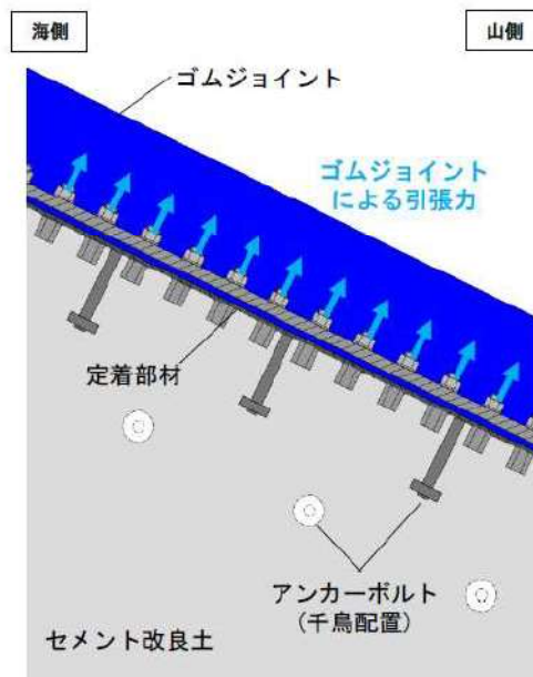
第 7-17 図 津波時にゴムジョイントの張力及び慣性力により定着部材及びアンカーボルトに生じる外力
