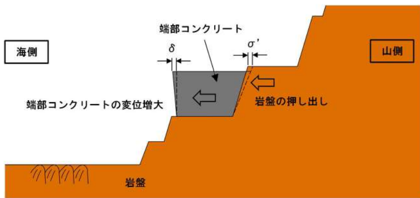
第 6-10 図 境界面のジョイント要素のイメージ図
