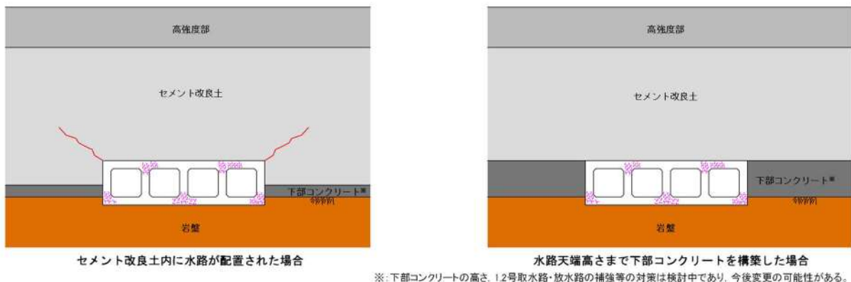
第5-48図 1号及び2号炉放水路が及ぼす堤体構造への悪影響
