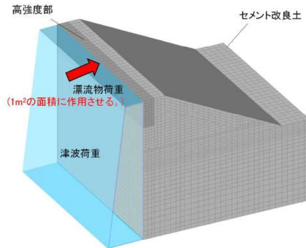
第 5-25 図 3次元静的FEM解析 解析モデル図（津波時）
