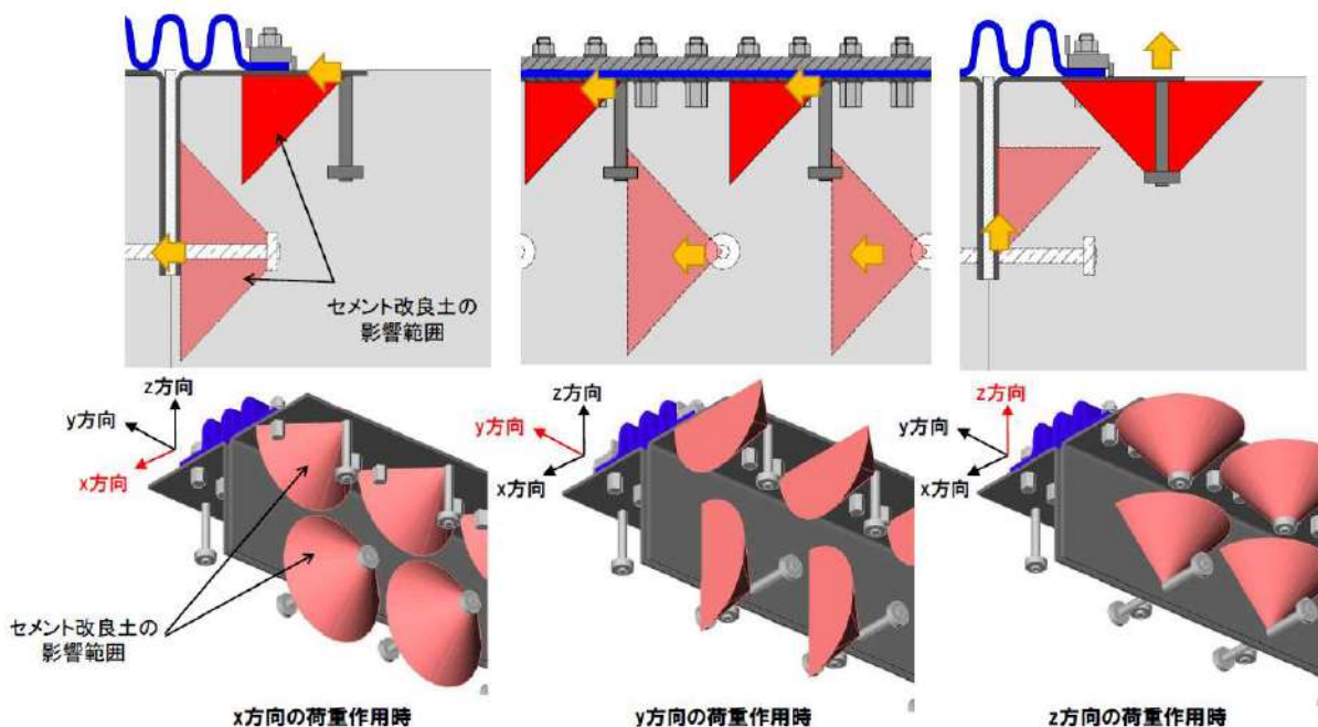
第 7-39 図 止水目地に作用した荷重により生じるセメント改良土の影響範囲
