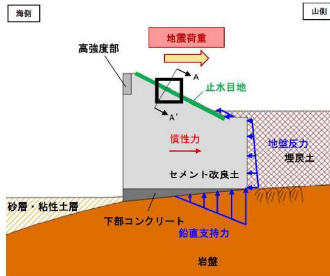
第 7-12 図 地震時に防潮堤に生じる外力
