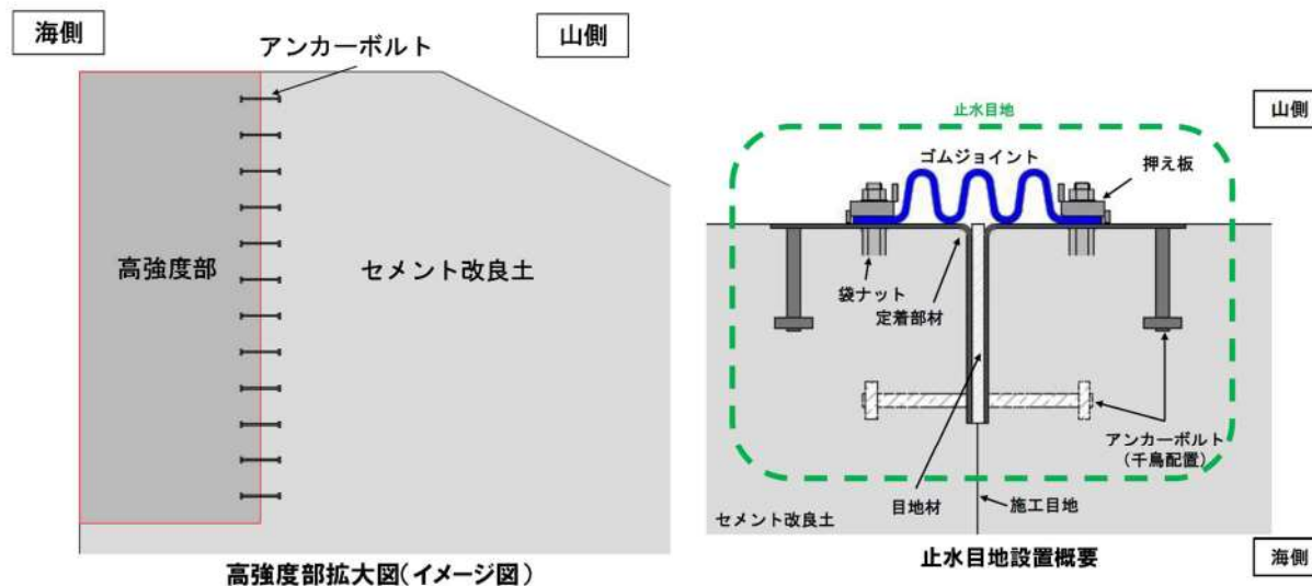
第 5-2 図 高強度部及び止水目地の構造概要
