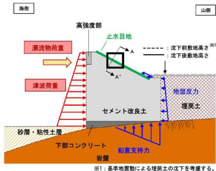
第 7-15 図 津波時に防潮堤に生じる外力
