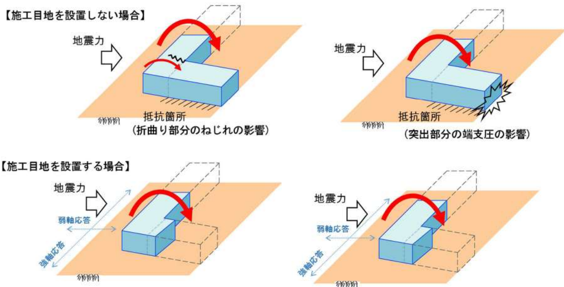
第5-39図 屈曲部形状による損傷モード(応力集中)のイメージ
