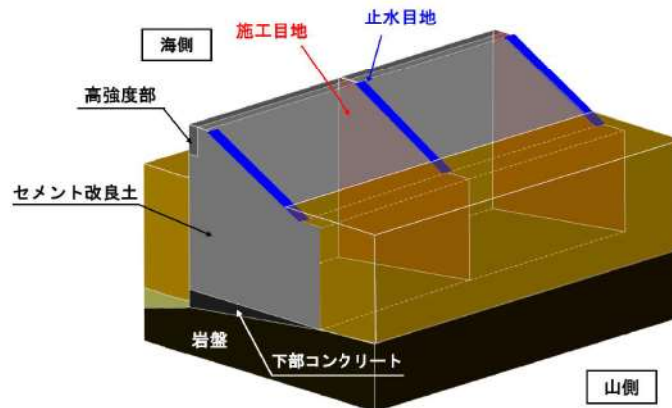
第 7-1 図 施工目地と止水目地の位置関係
