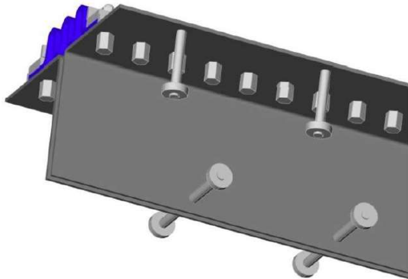
第 7-6 図 アンカーボルトの配置イメージ図
