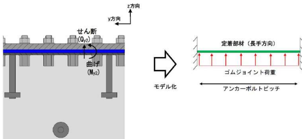
第 7-25 図 ゴムジョイントの張力により定着部材（長手方向）に生じる曲げ及びせん断の算出イメージ図（解析②）
