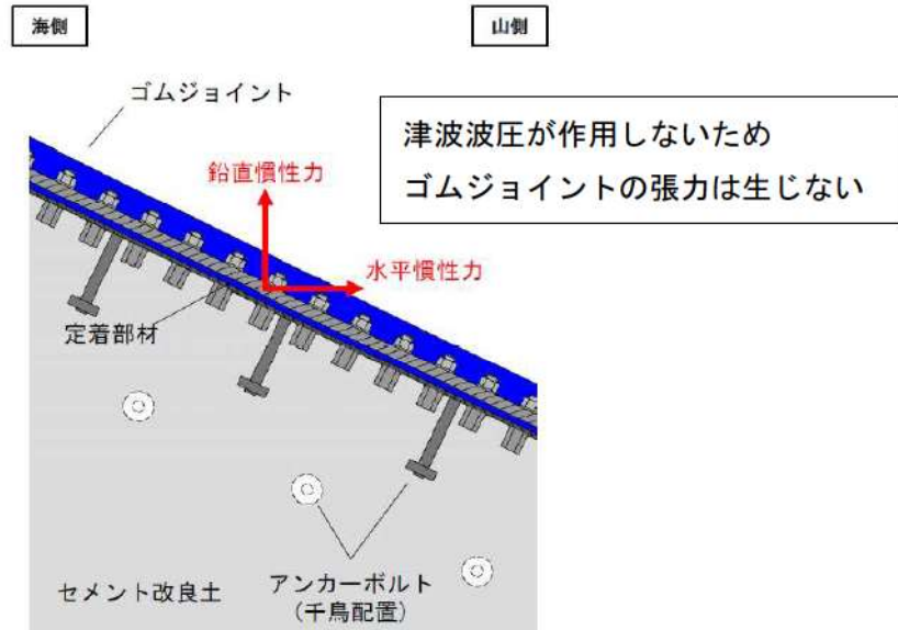
第 7-14 図 地震時にゴムジョイントの張力及び慣性力により定着部材及びアンカーボルトに生じる外力
