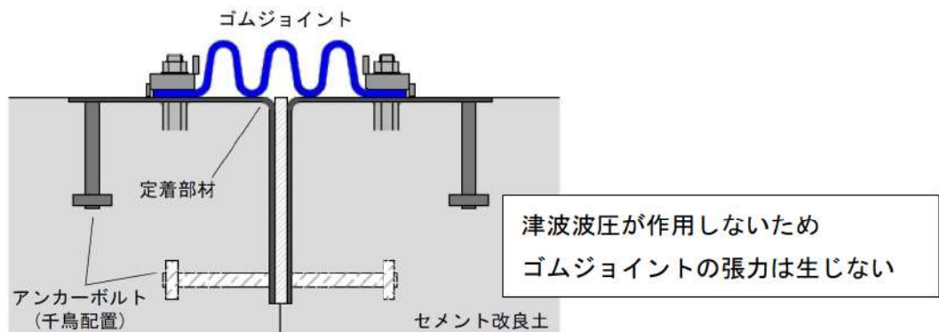
第 7-13 図 地震時にゴムジョイントの張力により定着部材及びアンカーボルトに生じる外力 (A-A' 断面)
