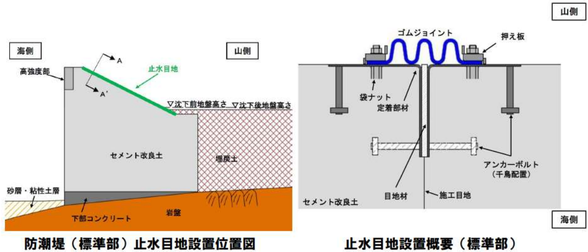
第 7-43 図 アンカーボルトの設置箇所（止水目地）
