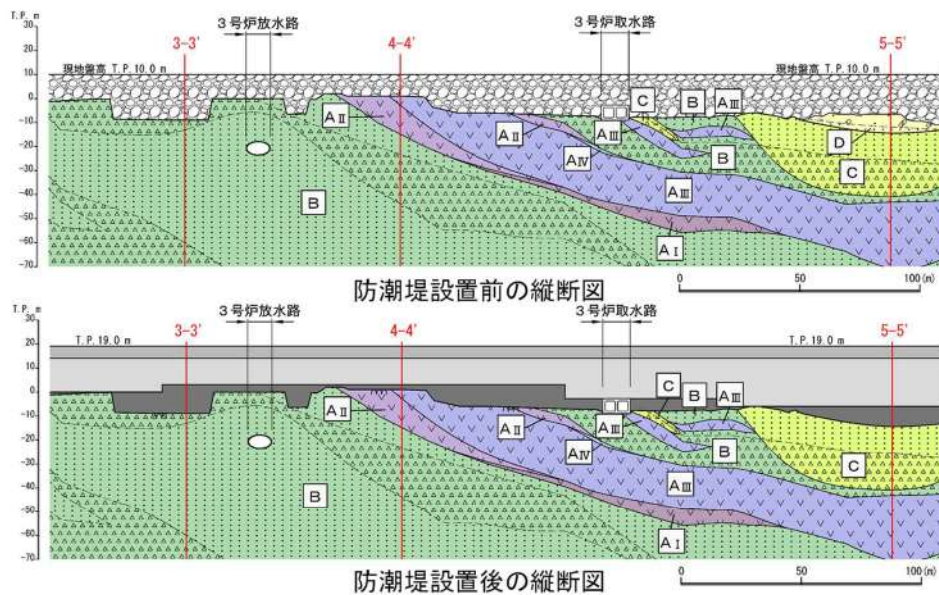
第 5-11 図 防潮堤（標準部）の地質縦断面図②
