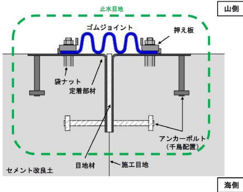
第 7-5 図 防潮堤（標準部）の止水目地の設置概要（A-A' 断面）
