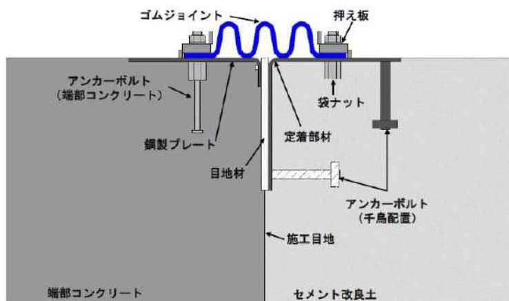
止水目地設置概要（A-A' 断面）
