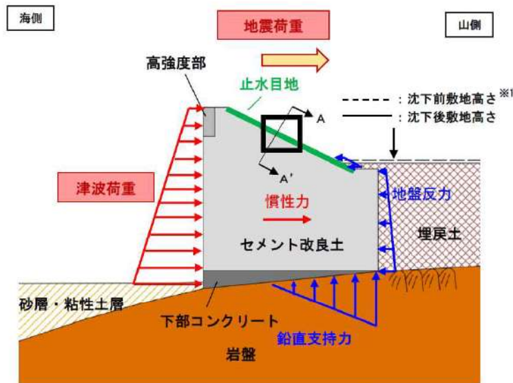
第 7-18 図 重畳時に防潮堤に生じる外力
