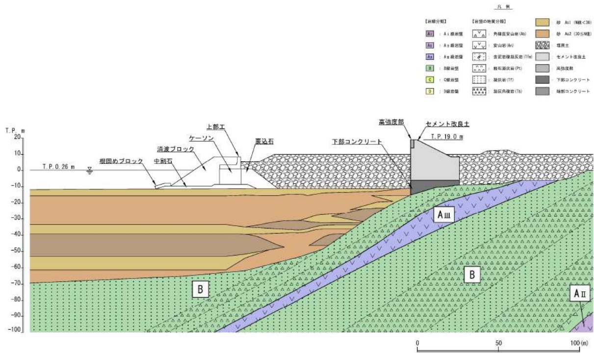
第 5-18 図 防潮堤（標準部）の地質横断図（6-6'）
