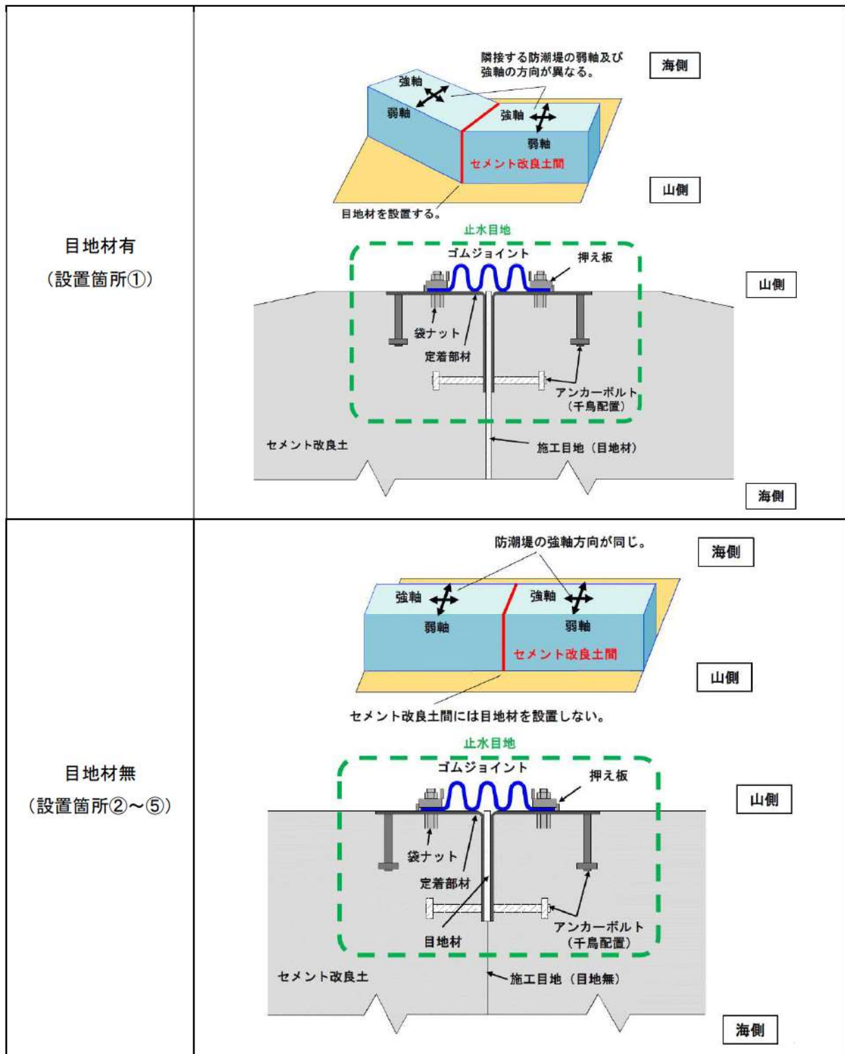
第 7-3 図 施工目地構造及び止水目地構造
