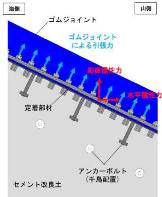
第 7-20 図 重疊時にゴムジョイントの張力及び慣性力により定着部材及びアンカーボルトに生じる外力
