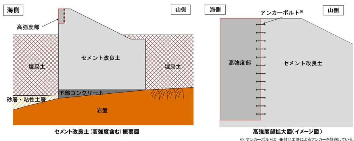
第 5-27 図 防潮堤（標準部）のセメント改良土及び高強度部の概略図
