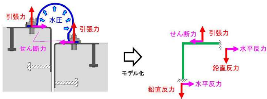
第 7-31 図 ゴムジョイントの張力によるアンカーボルト位置の反力算出イメージ図（解析②）
