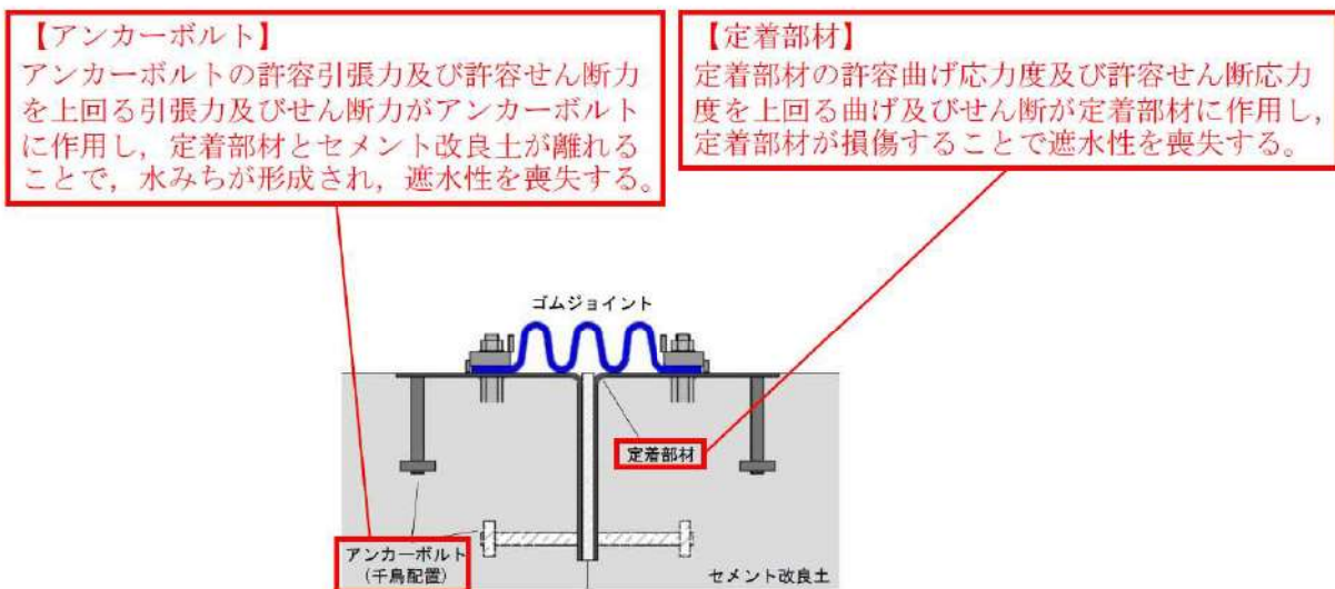
第 7-32 図 止水目地の構造上の弱部となる箇所（地震時）
