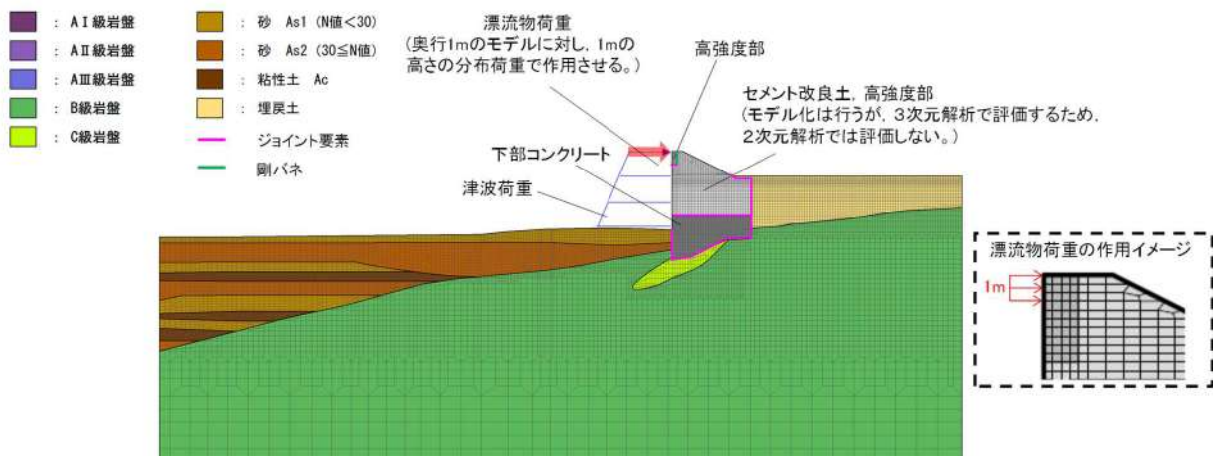
第 5-26 図 2次元動的FEM解析 解析モデル図（津波時）
