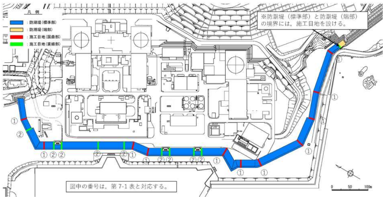
第 7-2 図 施工目地設置位置図
