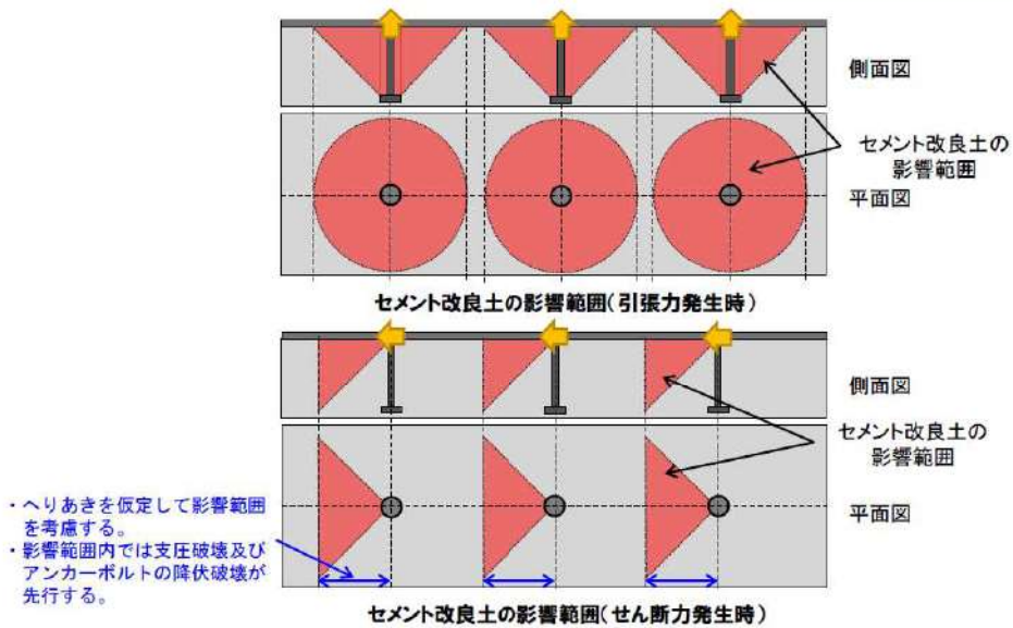
第 7-38 図 止水目地のアンカーボルトにおける引張力、せん断力発生時に生じるセメント改良土の影響範囲
