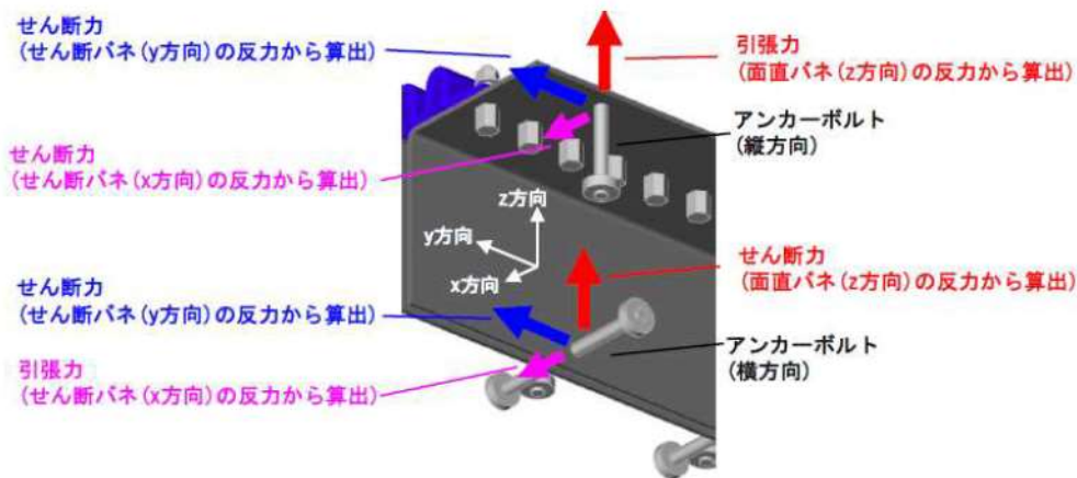
第 7-29 図 剛バネの反力とアンカーボルトに作用する引張力及びせん断力の方向（解析①）
