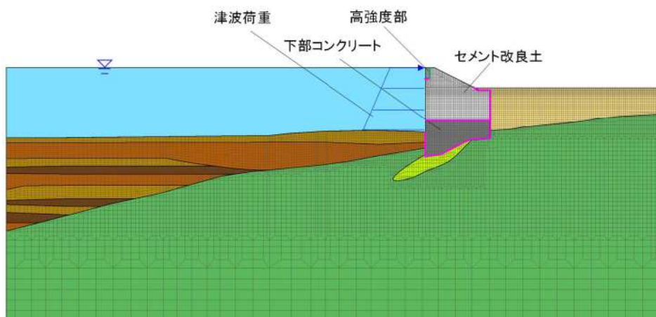
第 5-23 図 防潮堤（標準部）の2次元動的FEM解析モデル図（重畳時）
