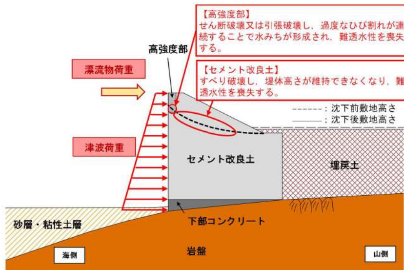
第 5-33 図 防潮堤（標準部）の構造上の弱部（津波時）
