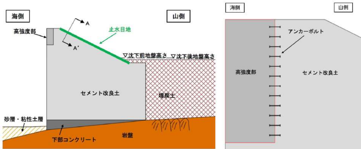
セメント改良土（高強度含む）概要図
