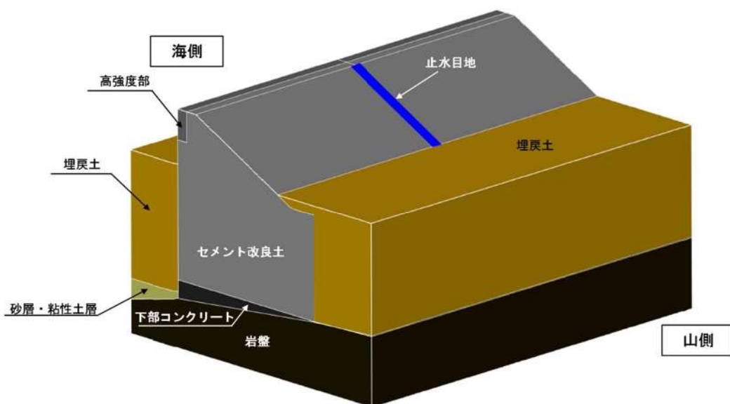
第 4-2 図 防潮堤（標準部）の概要図
