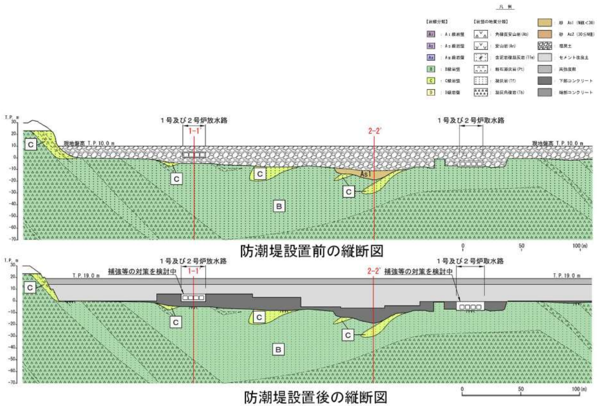
第 5-10 図 防潮堤（標準部）の地質縦断面図①
