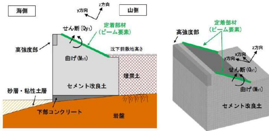
第 7-24 図 解析①のモデルと曲げ及びせん断のイメージ図 (左：地震時及び重畳時，右：津波時)
