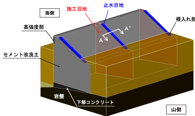
施工目地及び止水目地の設置位置
