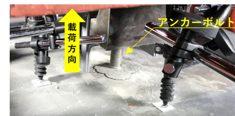
引張試験最大荷重載荷時の状況写真※2
