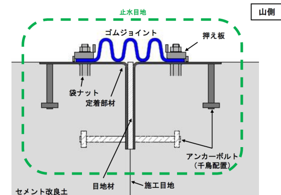
施工目地(直線部)における止水目地構造(A-A'断面)
