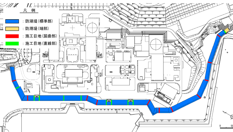
平面図(施工目地の位置)
