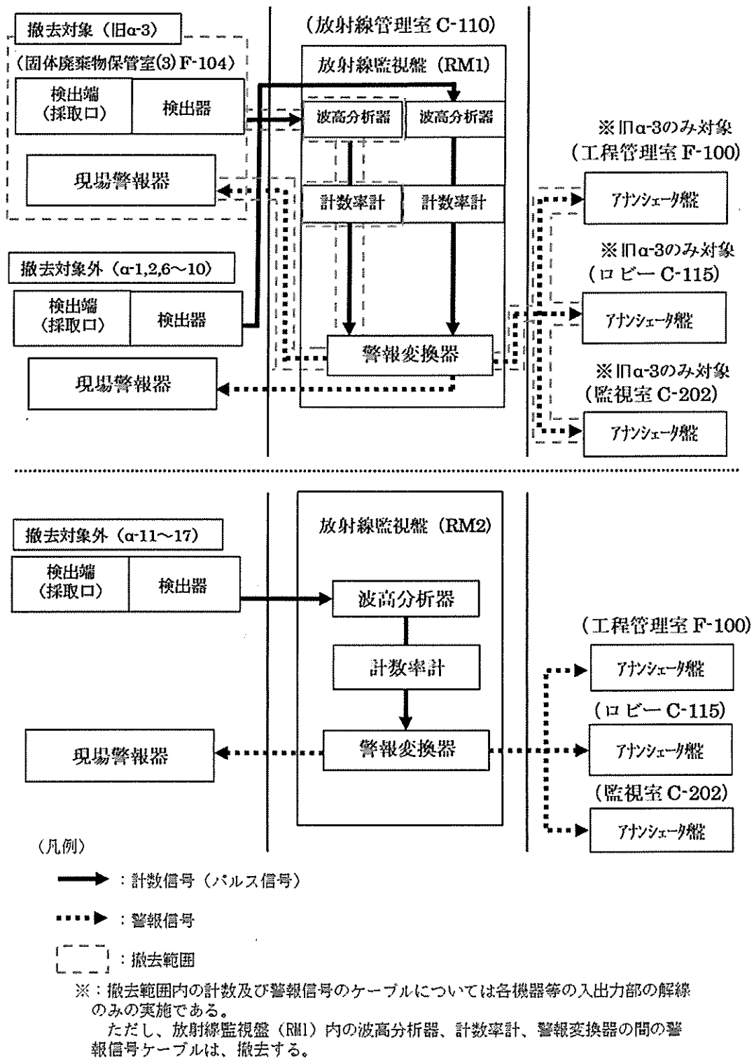
図 1-7 α線用空気モニタの構成図
