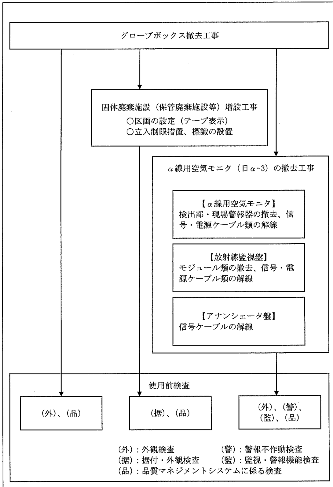
図1-4 工事フロー
