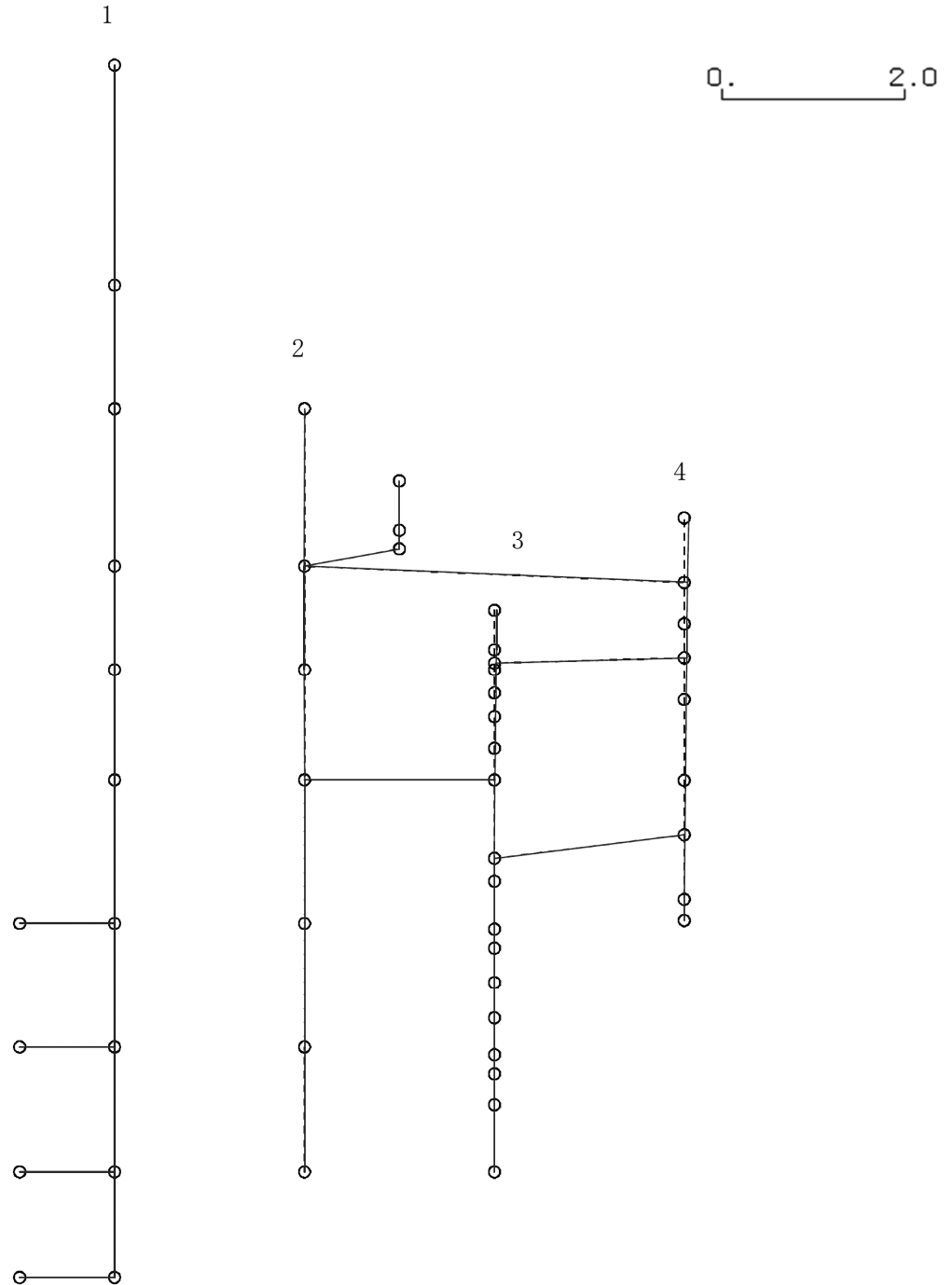
図 4-41 第 6 次刺激関数モード (EW 方向, Sd-3)
