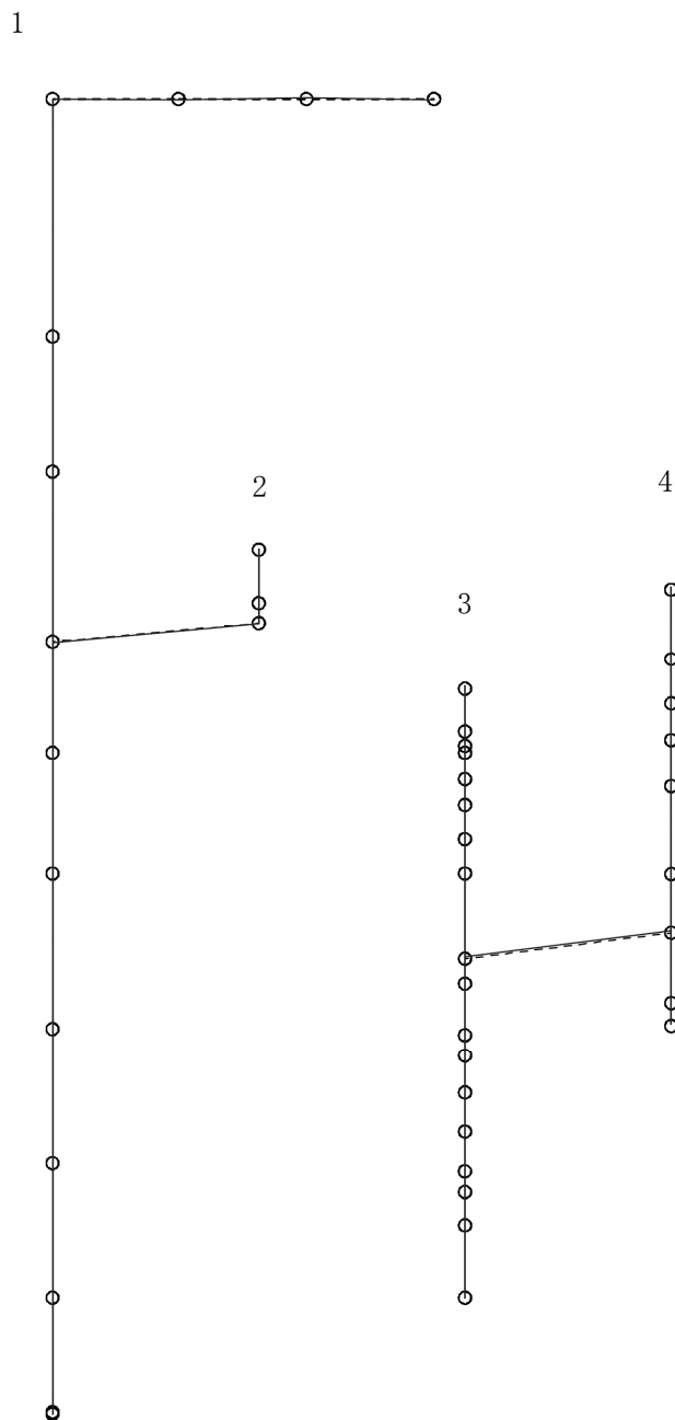
図 4-151 第 4 次刺激関数モード (鉛直方向, Sd-8)
