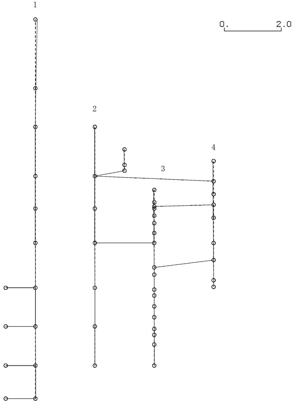
図 4-197 第 3 次刺激関数モード (NS 方向, Ss-4)
