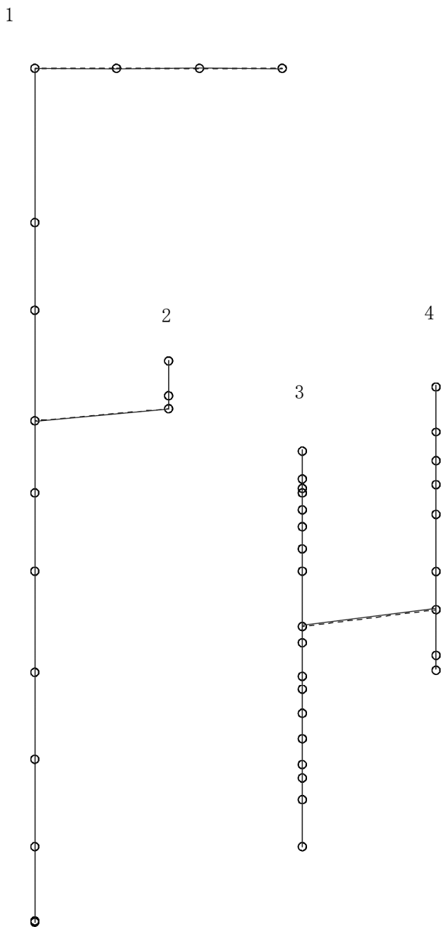
図 4-298 第4次刺激関数モード（鉛直方向, Ss-7)
