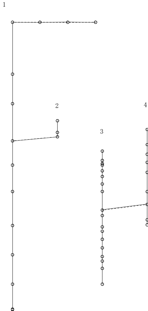
図 4-136 第 4 次刺激関数モード (鉛直方向, Sd-5)
