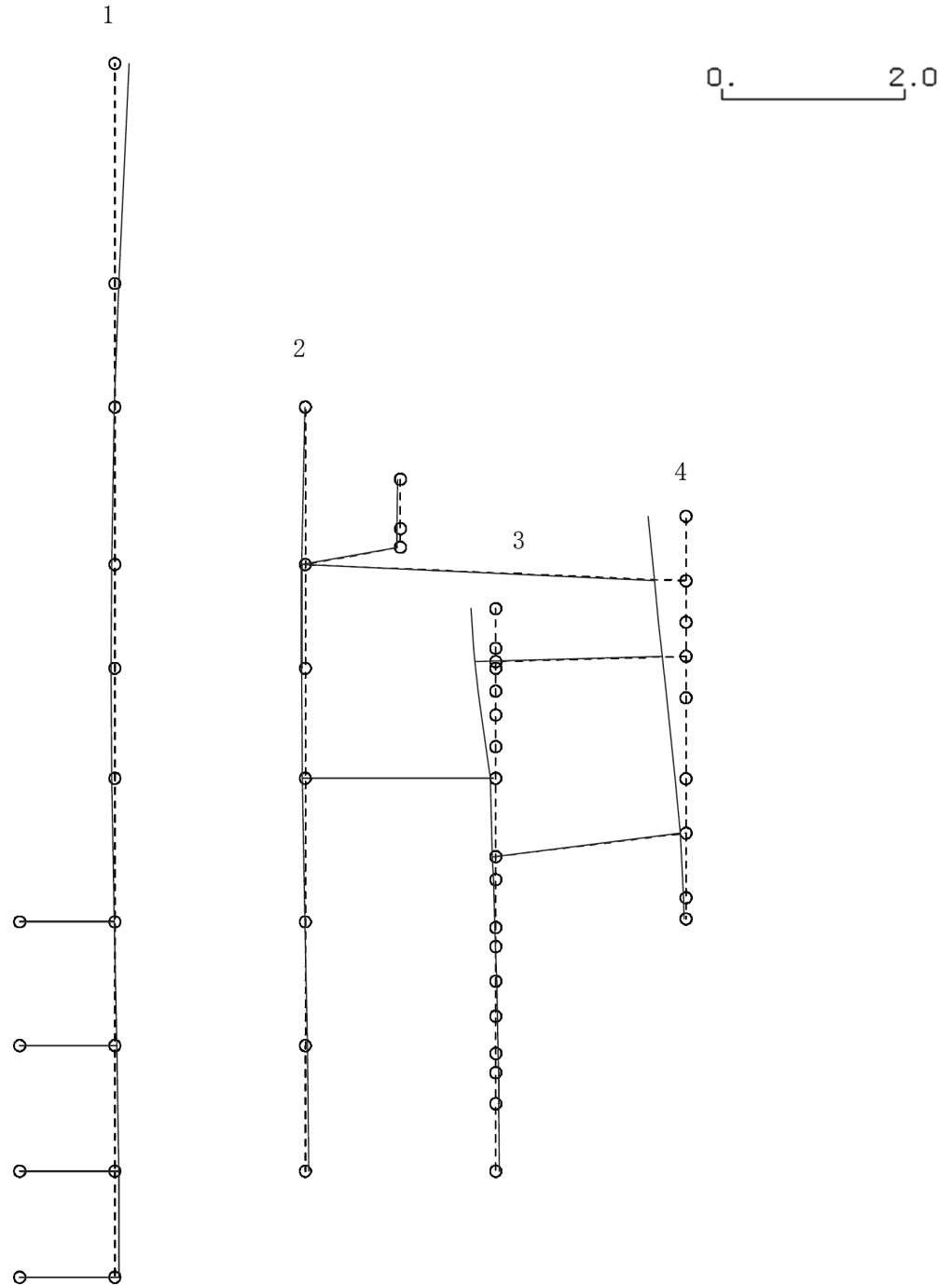
図4-11 第4次刺激関数モード (EW方向, Sd-1)
