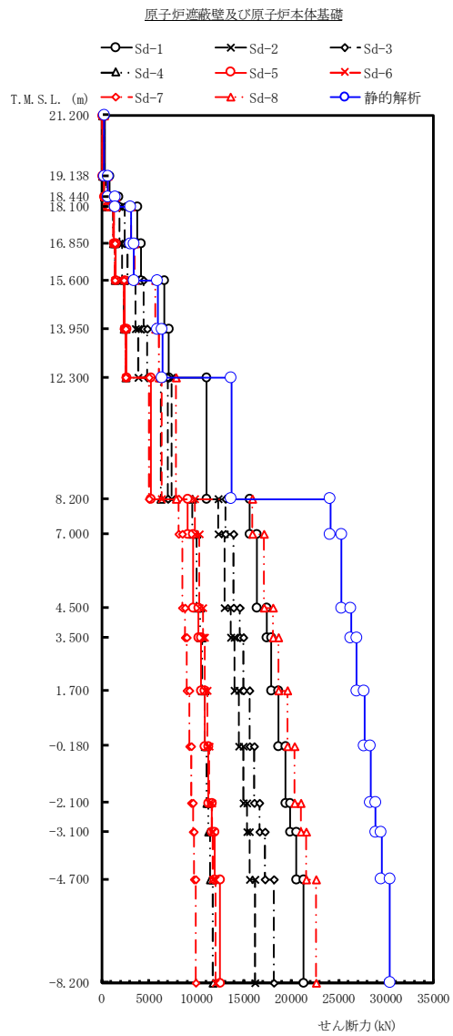
図 4-307 最大応答せん断力 弾性設計用地震動 S d 及び静的解析 (NS 方向 原子炉遮蔽壁及び原子炉本体基礎)
