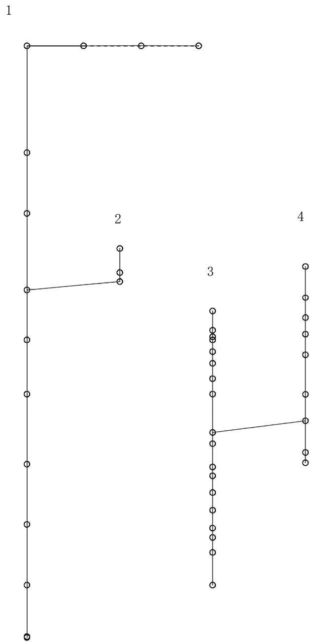
図 4-137 第 5 次刺激関数モード (鉛直方向, Sd-5)
