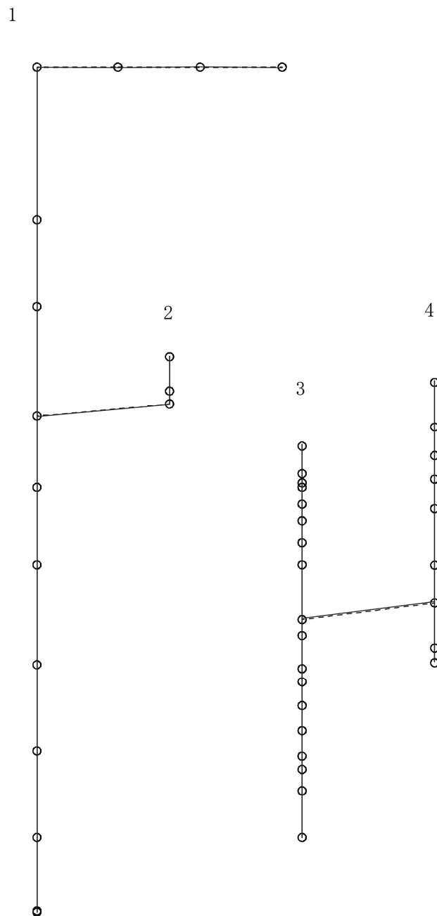
図4-288 第4次刺激関数モード（鉛直方向，Ss-5）
