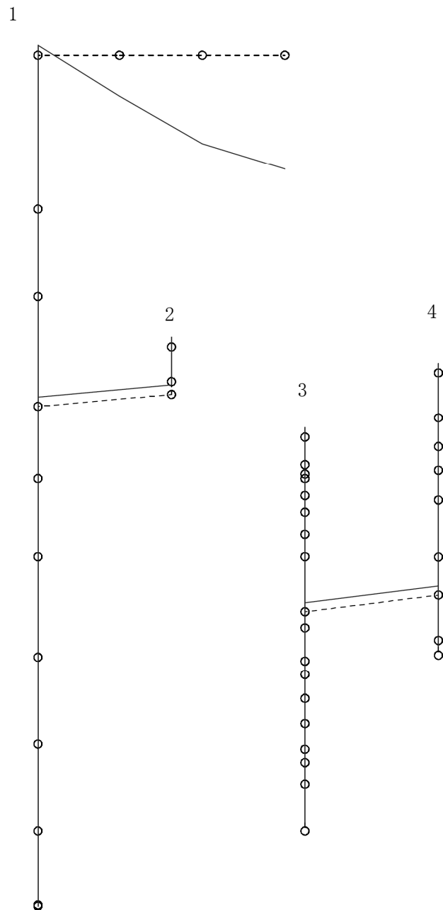
図 4-266 第2次刺激関数モード（鉛直方向, Ss-1)
