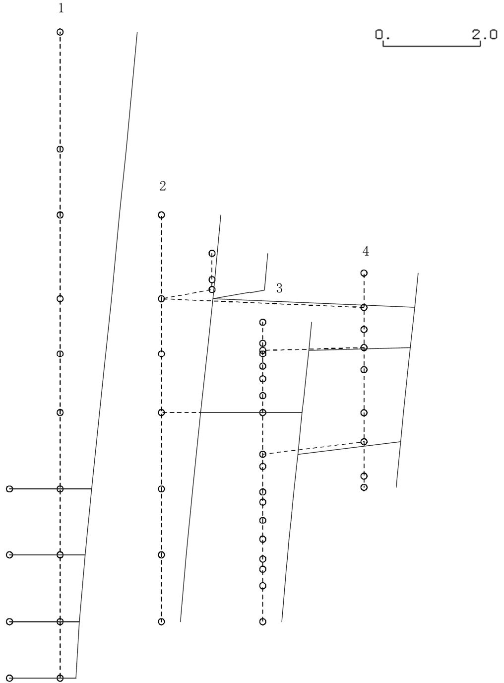
図 4-1 第 1 次刺激関数モード (NS 方向, Sd-1)
