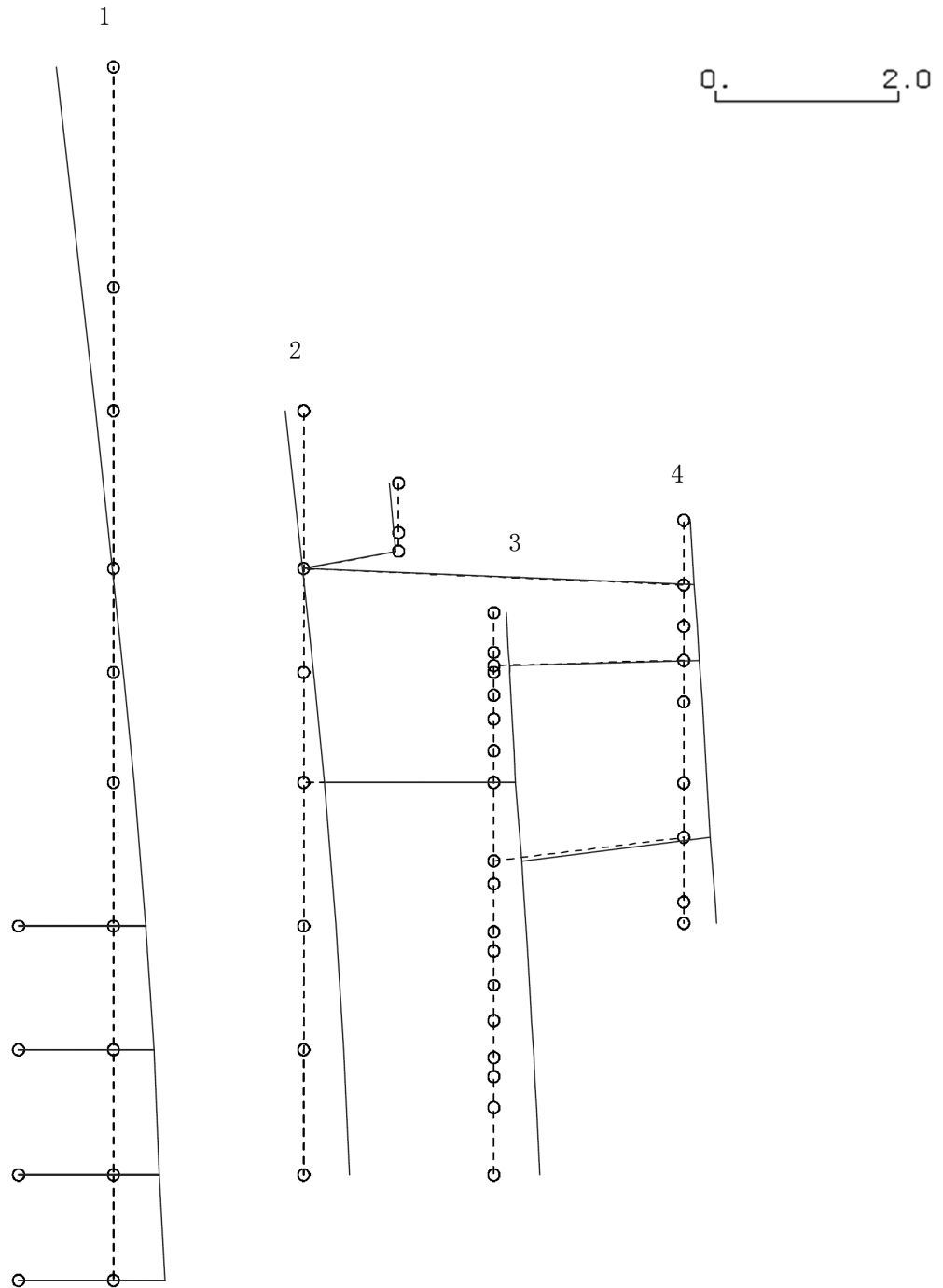
図4-37 第2次刺激関数モード (EW方向, Sd-3)
