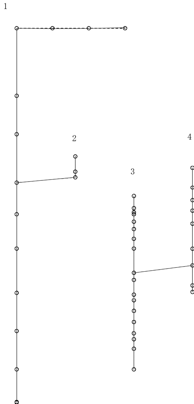
図 4-120 第 3 次刺激関数モード (鉛直方向, Sd-2)
