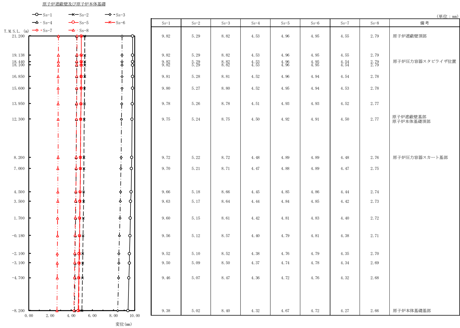
図 4-390 最大応答変位 基準地震動 S s (鉛直方向 原子炉遮蔽壁及び原子炉本体基礎)
