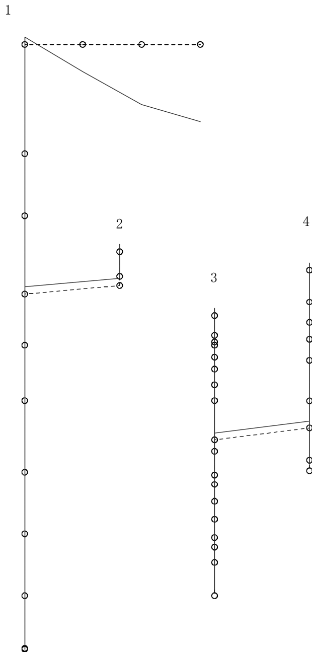
図4-271 第2次刺激関数モード(鉛直方向, Ss-2)
