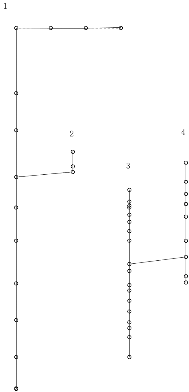
図4-272 第3次刺激関数モード（鉛直方向，Ss-2）
