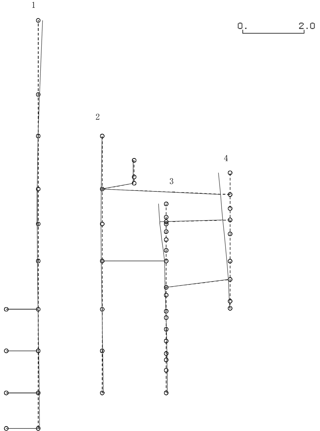
図 4-191 第 4 次刺激関数モード (EW 方向, Ss-3)
