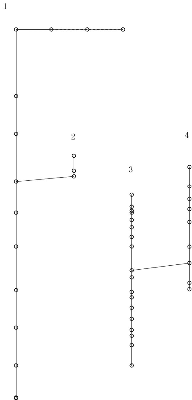
図 4-132 第 5 次刺激関数モード（鉛直方向，Sd-4）
