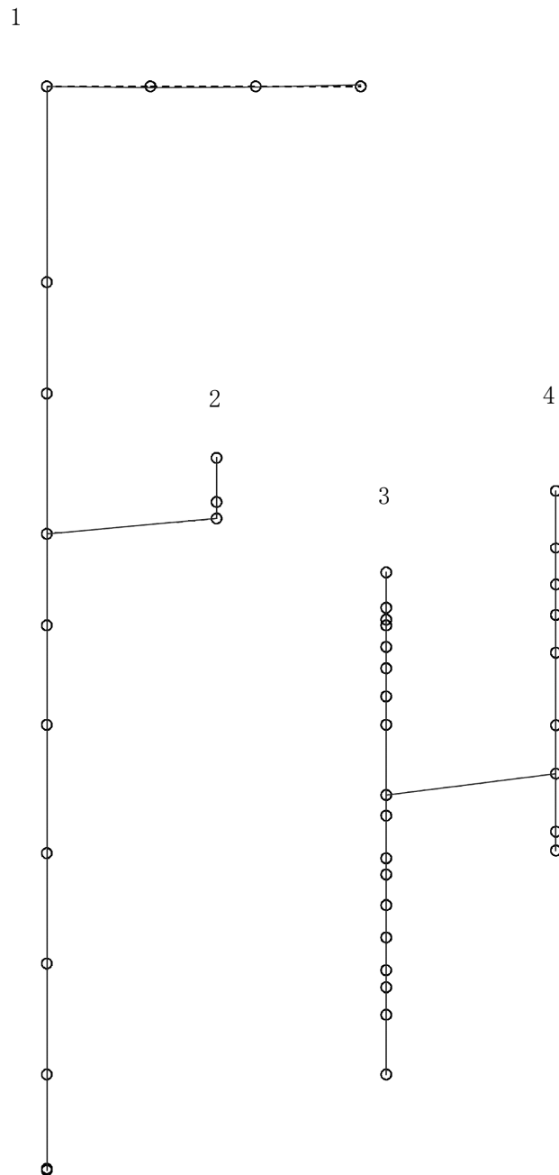
図 4-150 第 3 次刺激関数モード (鉛直方向, Sd-8)
