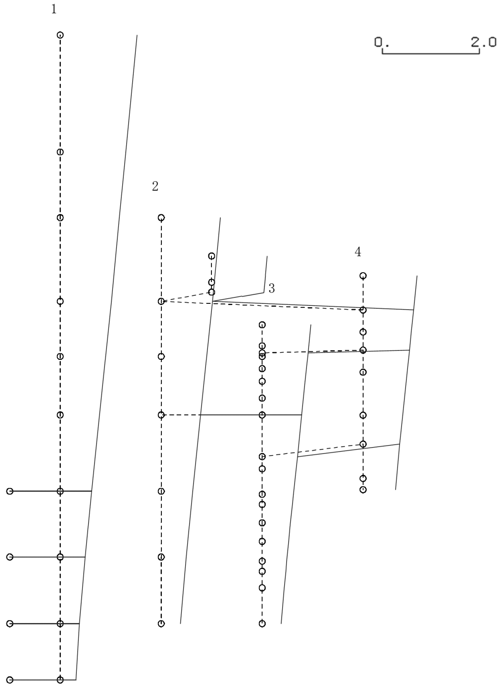
図 4-195 第 1 次刺激関数モード (NS 方向, Ss-4)
