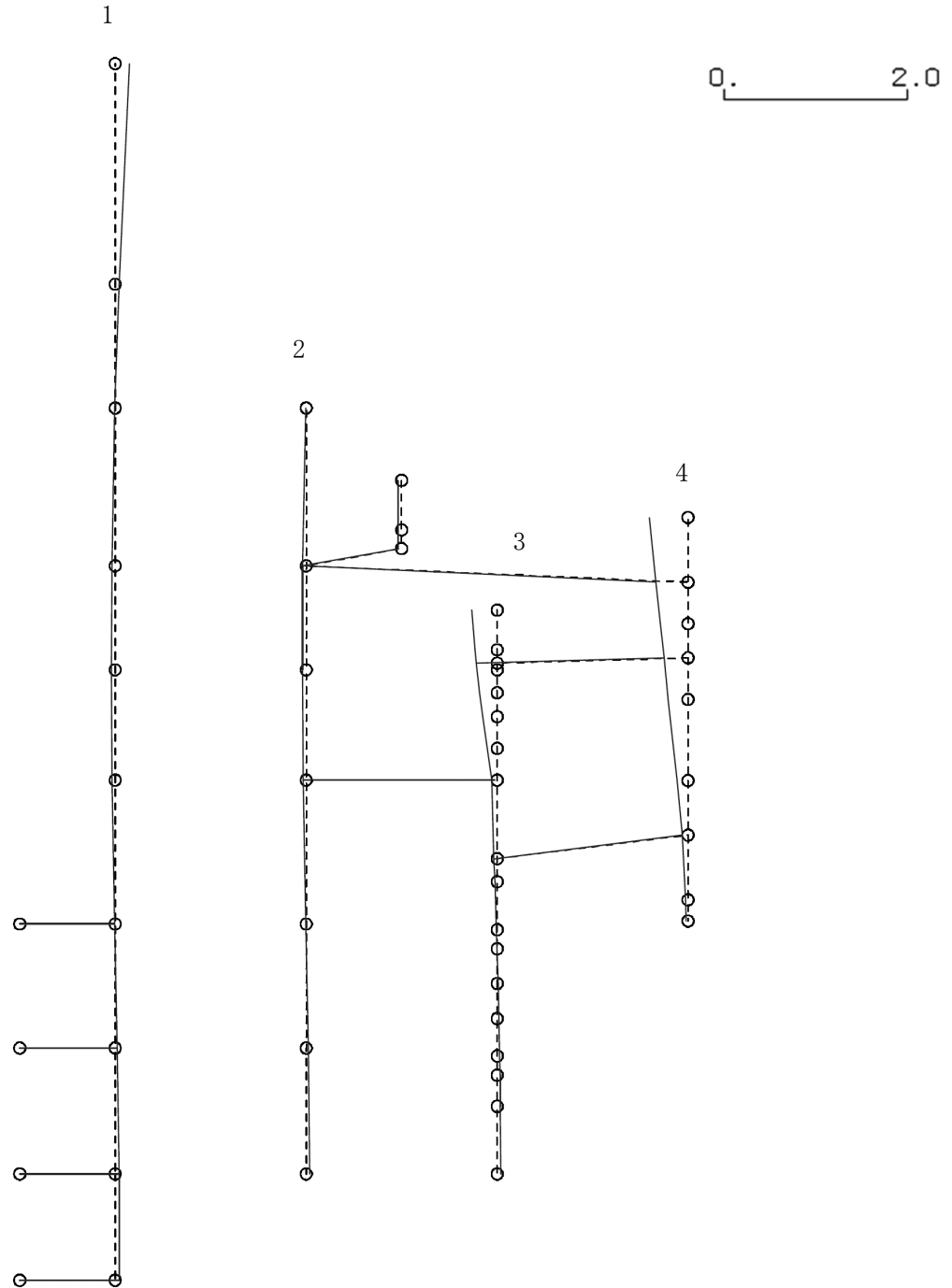
図4-95 第4次刺激関数モード (EW方向, Sd-7)
