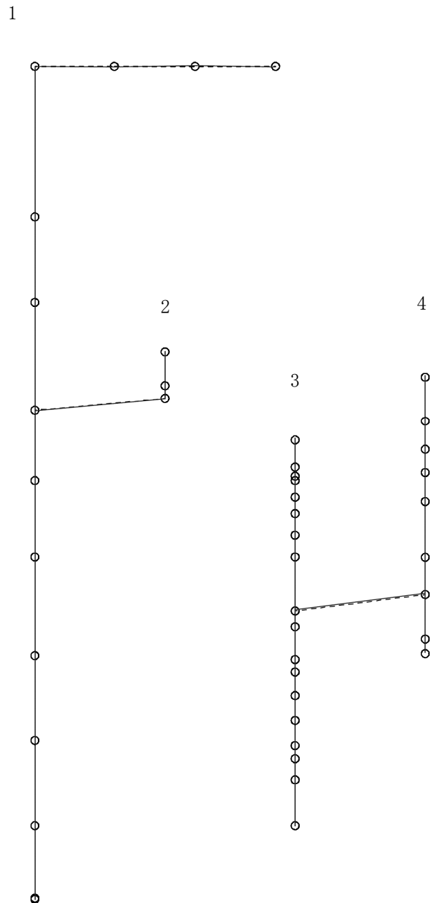
図4-121 第4次刺激関数モード（鉛直方向、Sd-2）
