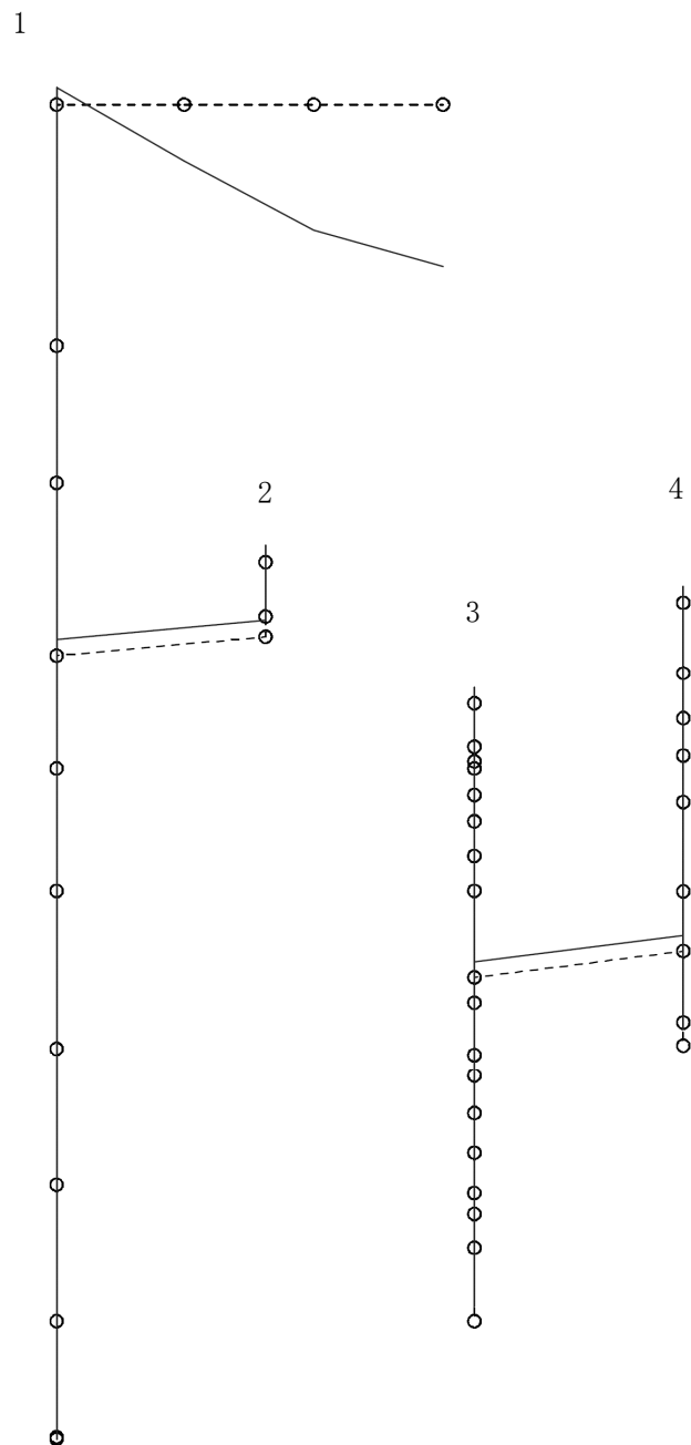
図 4-281 第 2 次刺激関数モード (鉛直方向, Ss-4)
