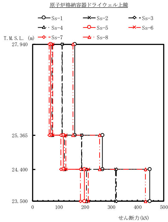
図 4-367 最大応答せん断力 基準地震動 S s (NS 方向 原子炉格納容器ドライウエル上鏡)
