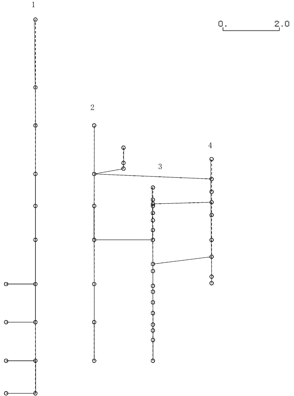
図 4-162 第 3 次刺激関数モード (EW 方向, Ss-1)
