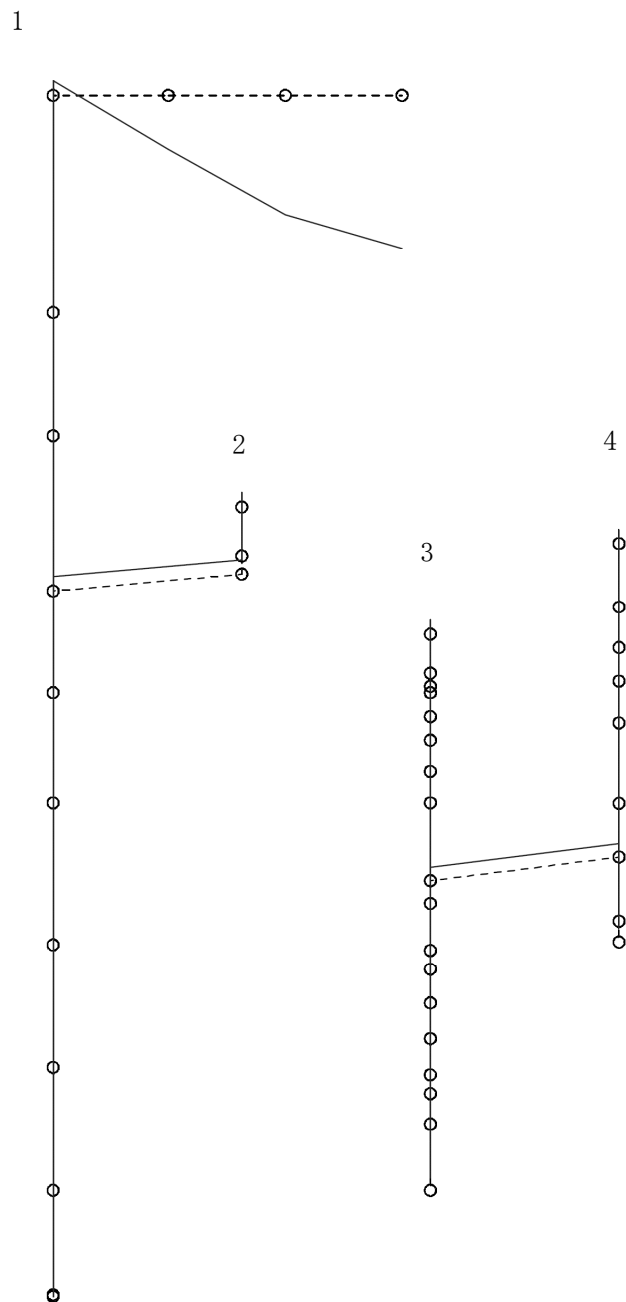
図 4-286 第 2 次刺激関数モード (鉛直方向, Ss-5)
