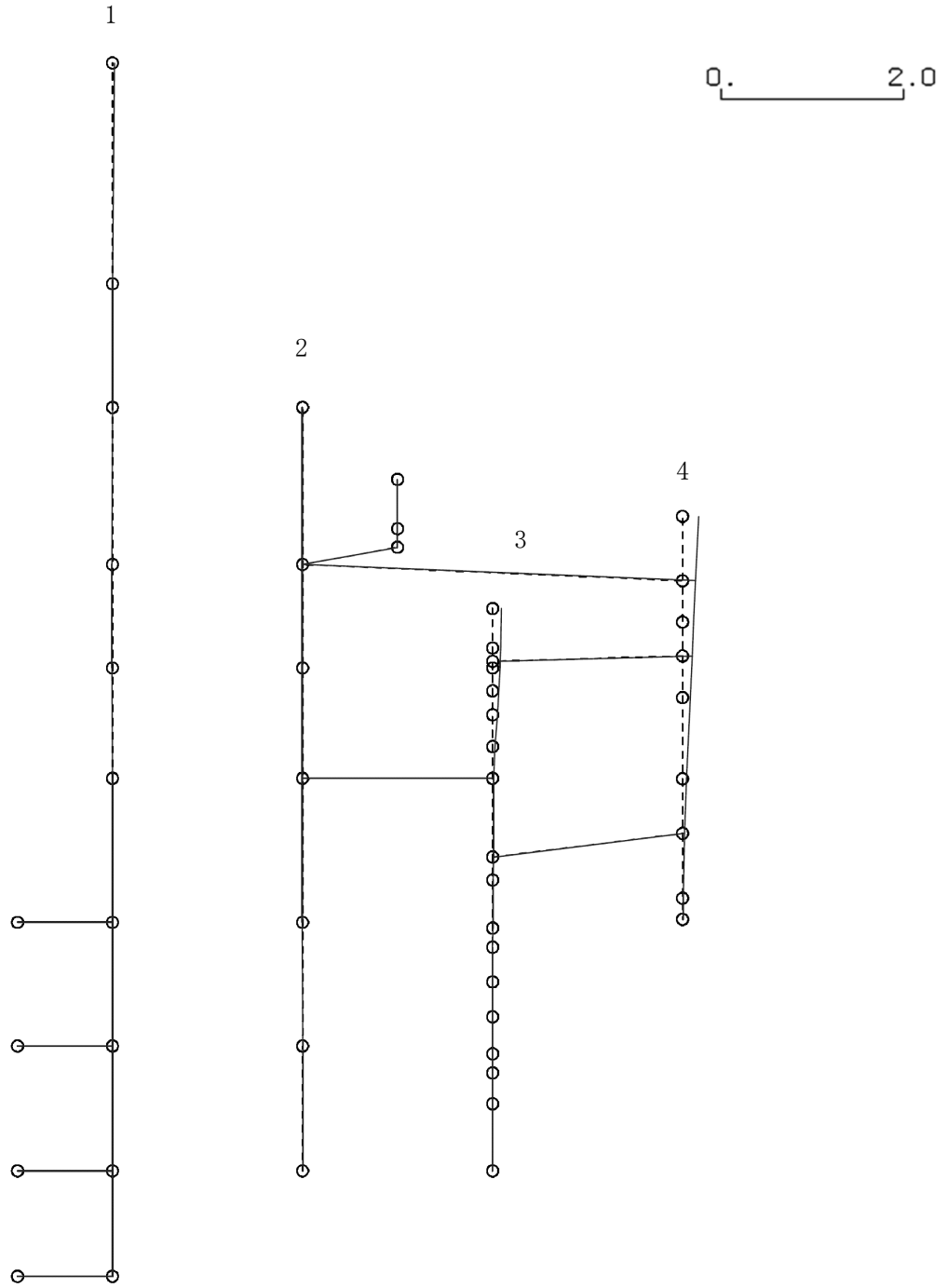
図 4-242 第 6 次刺激関数モード (NS 方向, Ss-7)
