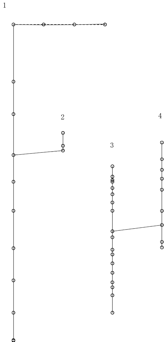
図 4-115 第 3 次刺激関数モード (鉛直方向, Sd-1)
