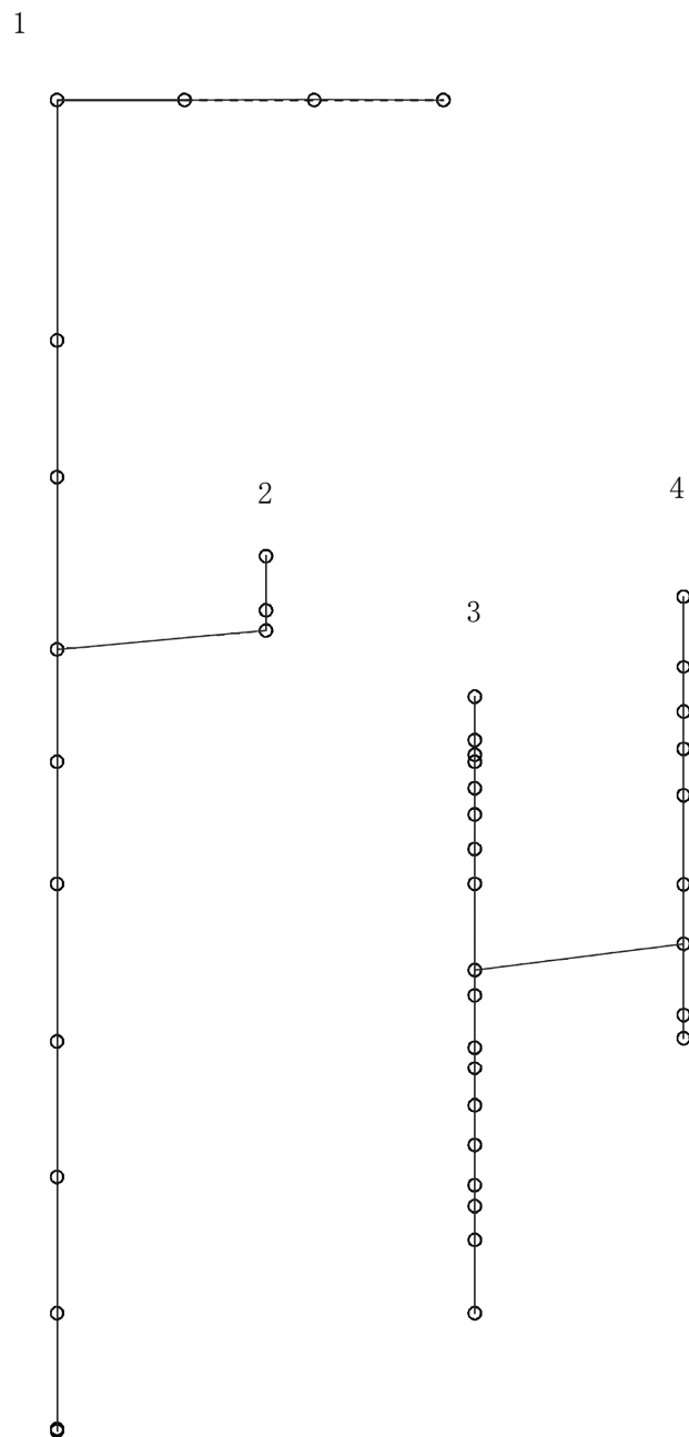
図 4-304 第 5 次刺激関数モード (鉛直方向, Ss-8)
