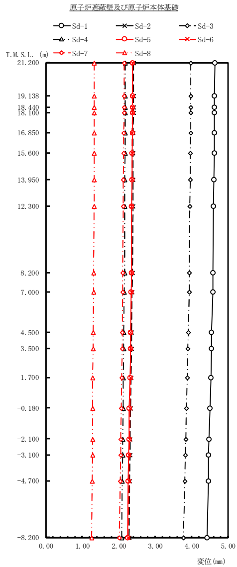
図 4-342 最大応答変位 弾性設計用地震動 S d (鉛直方向 原子炉遮蔽壁及び原子炉本体基礎)
