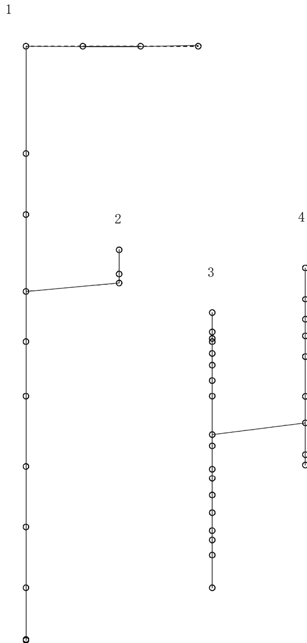
図 4-302 第 3 次刺激関数モード (鉛直方向, Ss-8)
