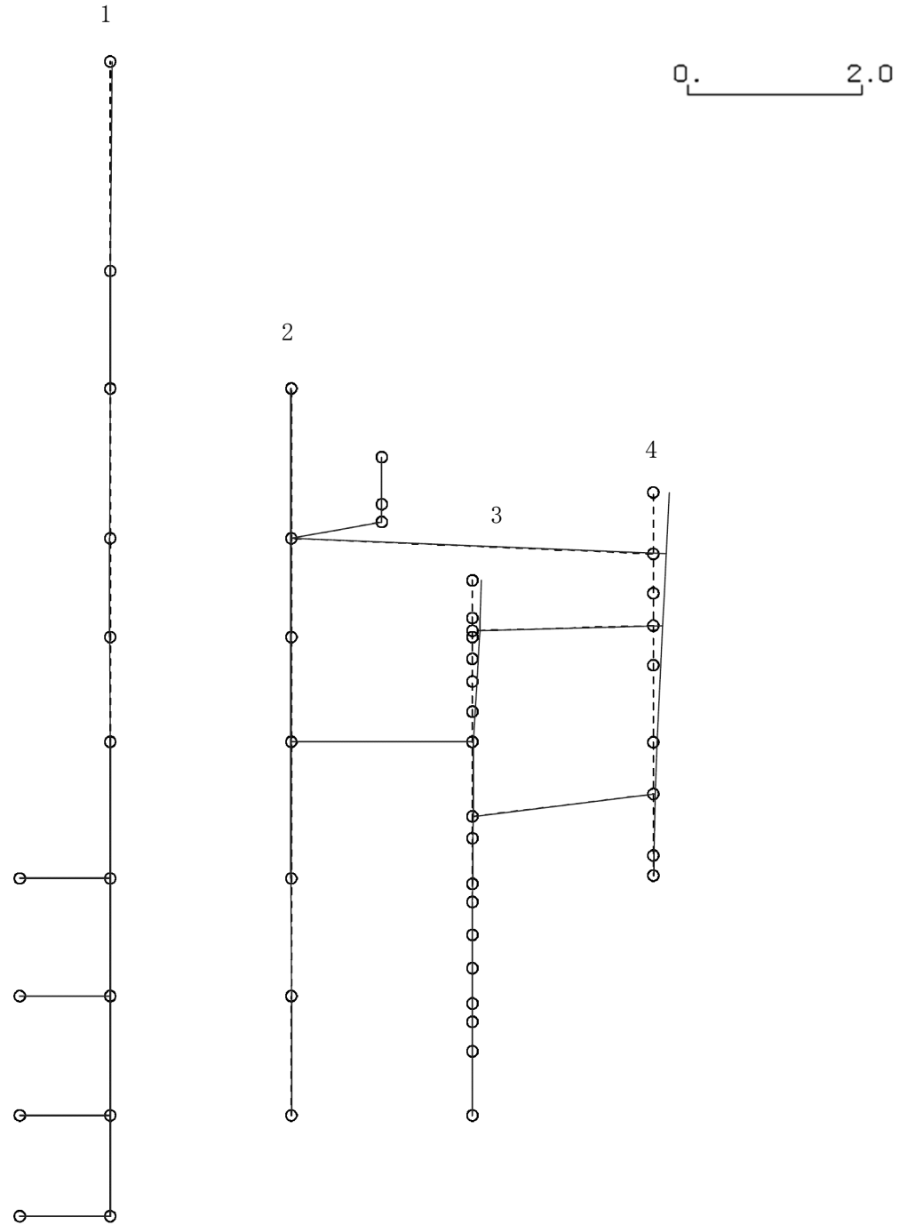
図4-90 第6次刺激関数モード (NS方向, Sd-7)
