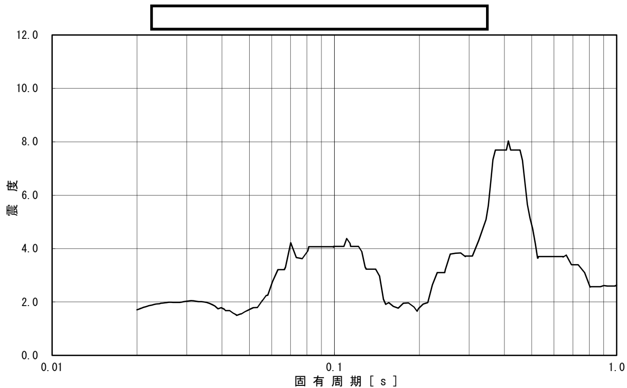
図 12(1) 検討用床応答曲線（主蒸気系配管用）
