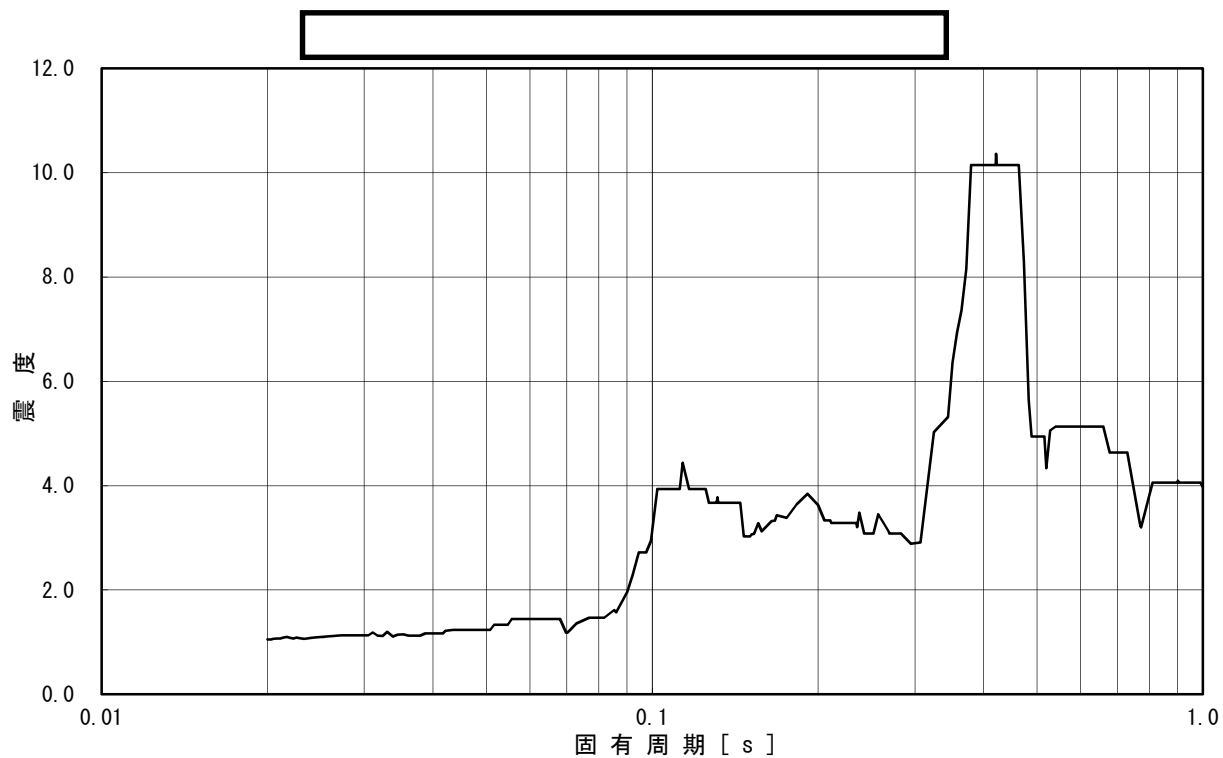
図 12(3) 検討用床応答曲線 (原子炉補機冷却水系配管用)
