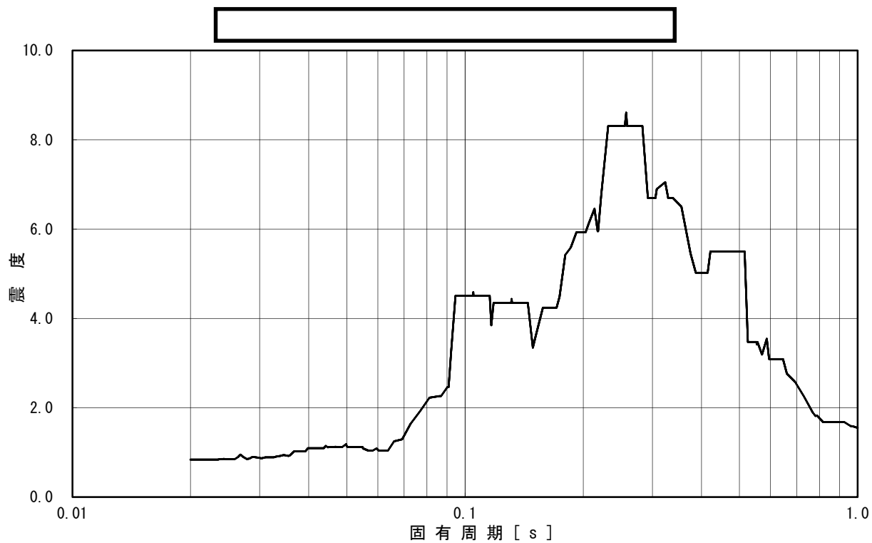
図 12(4) 検討用床応答曲線 (原子炉補機冷却水系配管用)
