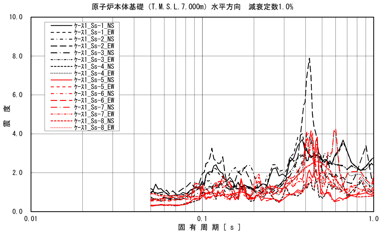
添付図 3(10) 原子炉本体基礎 (T. M. S. L. 7. 000m) の加速度応答スペクトル (水平方向, 減衰定数 1.0%)
