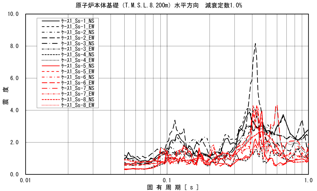
添付図 3(9) 原子炉本体基礎 (T. M. S. L. 8. 200m) の加速度応答スペクトル (水平方向, 減衰定数 1.0%)
