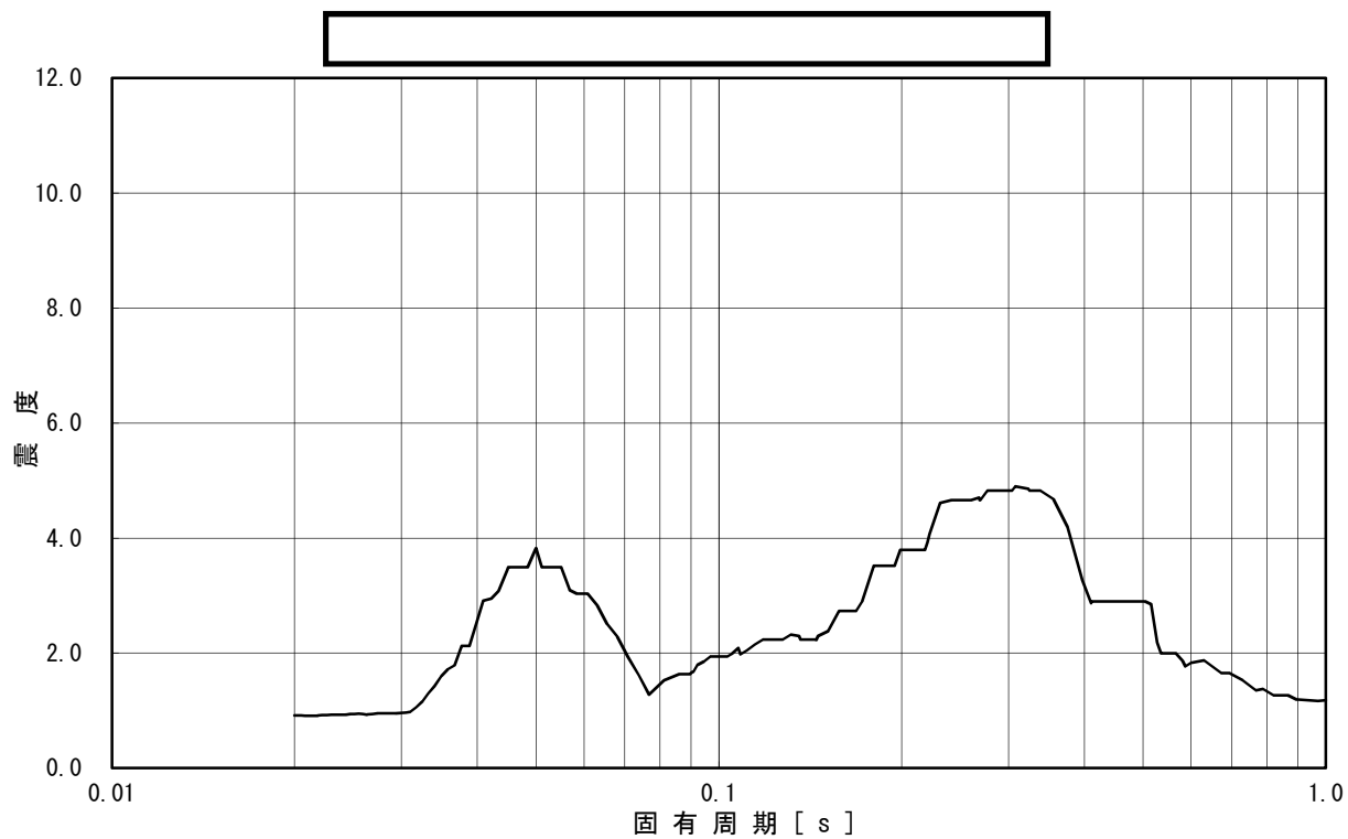
図 12(2) 検討用床応答曲線（主蒸気系配管用）
